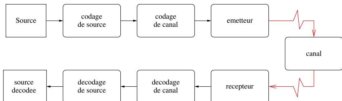
FIG. 1.1 – Schéma de transmission séparé.
