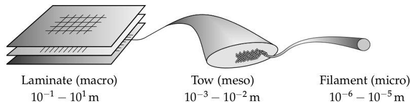
Figure 1.1 Exemple de hiérarchie multi-échelles des milieux fibreux : un renfort textile constitué de mèches de fibres pour composite, d'après CORNELISSEN [22].
