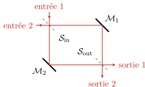
Fig. 1.8 – Interféromètre de Mach–Zehnder optique. Un faisceau lumineux entrant est séparé par une lame séparatrice d'entrée \mathcal{S}_{in} . Les faisceaux émergents parcourent une des voies de l'interféromètre en se réfléchissant sur l'un des miroirs \mathcal{M}_1 ou \mathcal{M}_2 et sont recombinés par la lame séparatrice de sortie \mathcal{S}_{out} . Les interférences sont observables dans les deux voies de sortie, qui sont dans des états d'interférences opposés.
