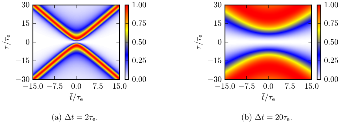
Fig. 3.12 – Degré de cohérence à deux électrons de paires de levitons. Les deux levitons sont monoélectroniques, séparés de (a) \Delta t = 2\tau_e , et (b) \Delta t = 20\tau_e . Le calcul se base sur le théorème de Wick et prend en compte le recouvrement. Les échelles de temps sont les mêmes sur les deux figures et sur la figure 3.11.
