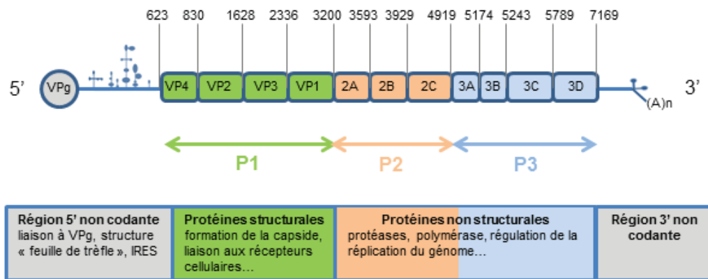
Figure 3. Organisation génomique des rhinovirus.
