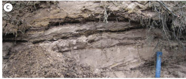
Sigmoïdes tidales
