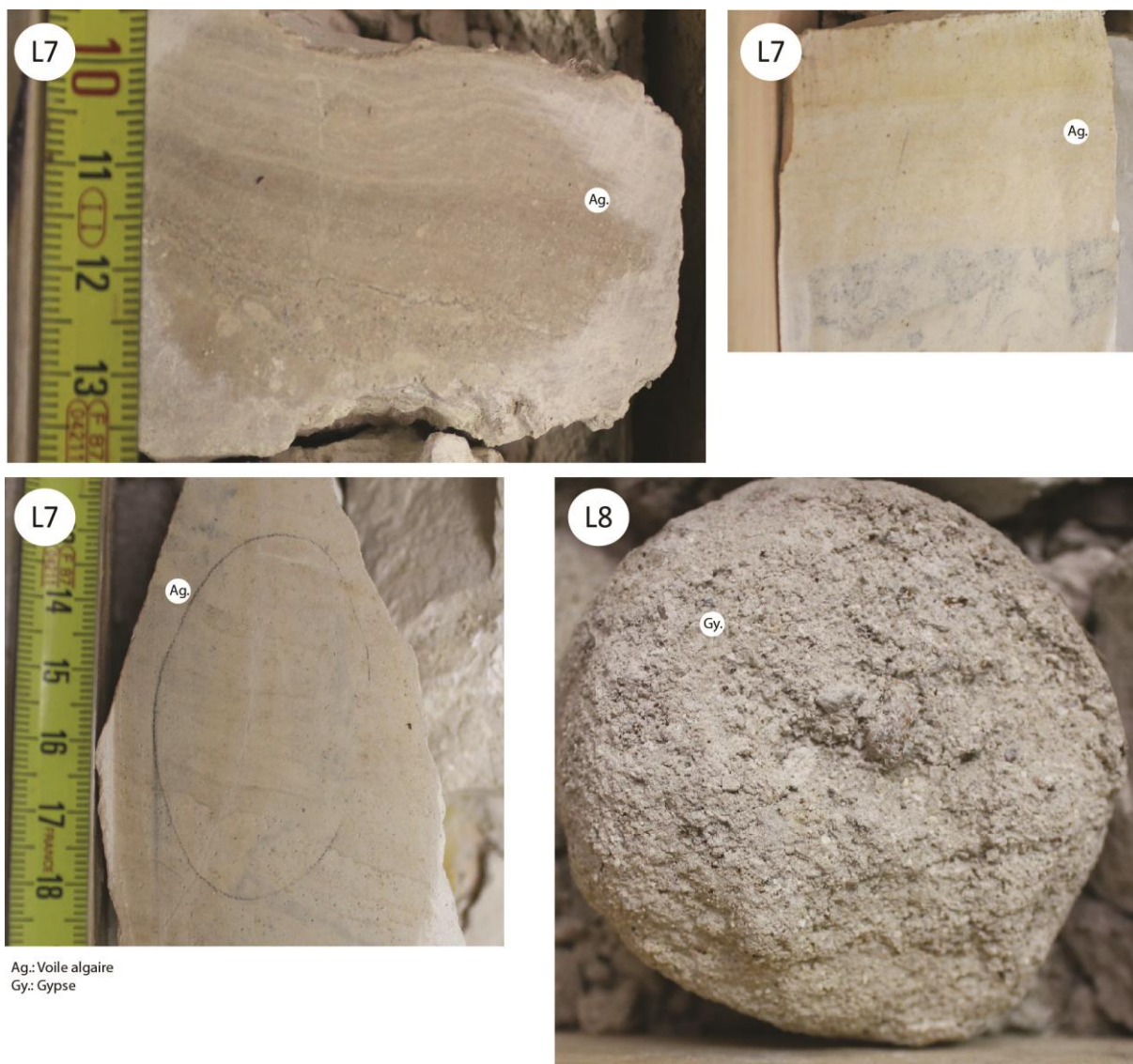
Figure 4.16 : Faciès d'Ussy-sur-Marne
