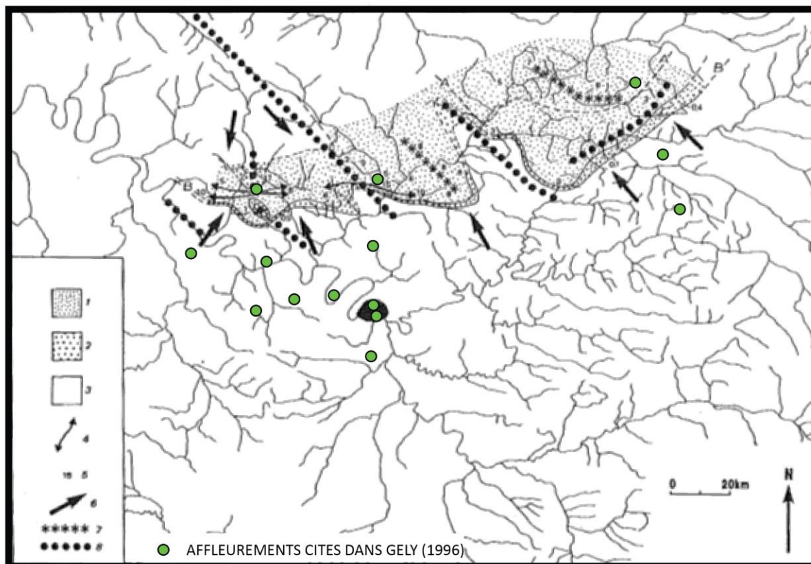
Figure 4.3 : Carte paléogéographique de la paraséquence A4, sommet de la "Glaucolie Grossière". Les lignes en pointillés représentent (A) la limite de la paraséquence A3 et (B) la limite de la paraséquences A4. Légende : (1) faciès transgressif calcaire ; (2) faciès transgressif sableux ; (3) domaine émergé ; (4) chenaux majeurs ; (5) épaisseurs cumulées des paraséquences A1 à A4 ; (6) directions des apports détritiques continentaux ; (7) région subsidente ; (8) région faiblement subsidente ou en surrection.
