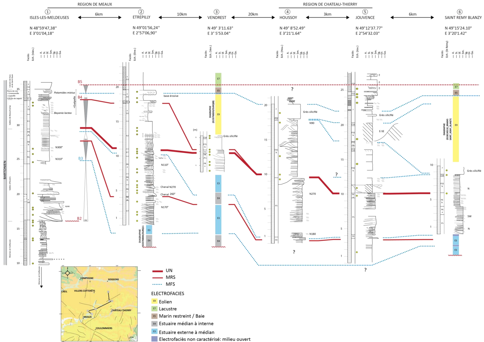
Figure 5.22 : Corrélation des coupes sédimentologiques des sables bartoniens de la région de Meaux à la région de Château-Thierry
