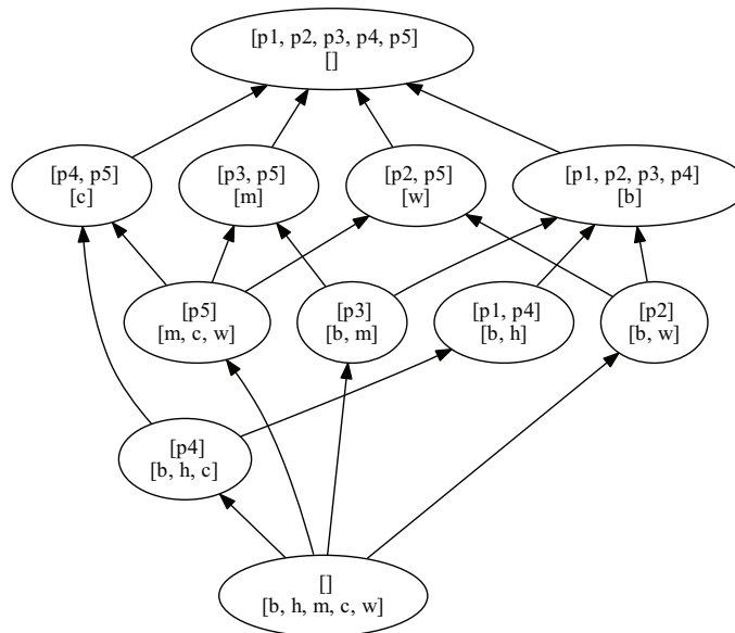
FIGURE 7.11 – Treillis des concepts généré à partir de l'inversion du contexte du tableau 7.3. Les observations constituent l'intension des concepts, les attributs forment leurs extensions.
