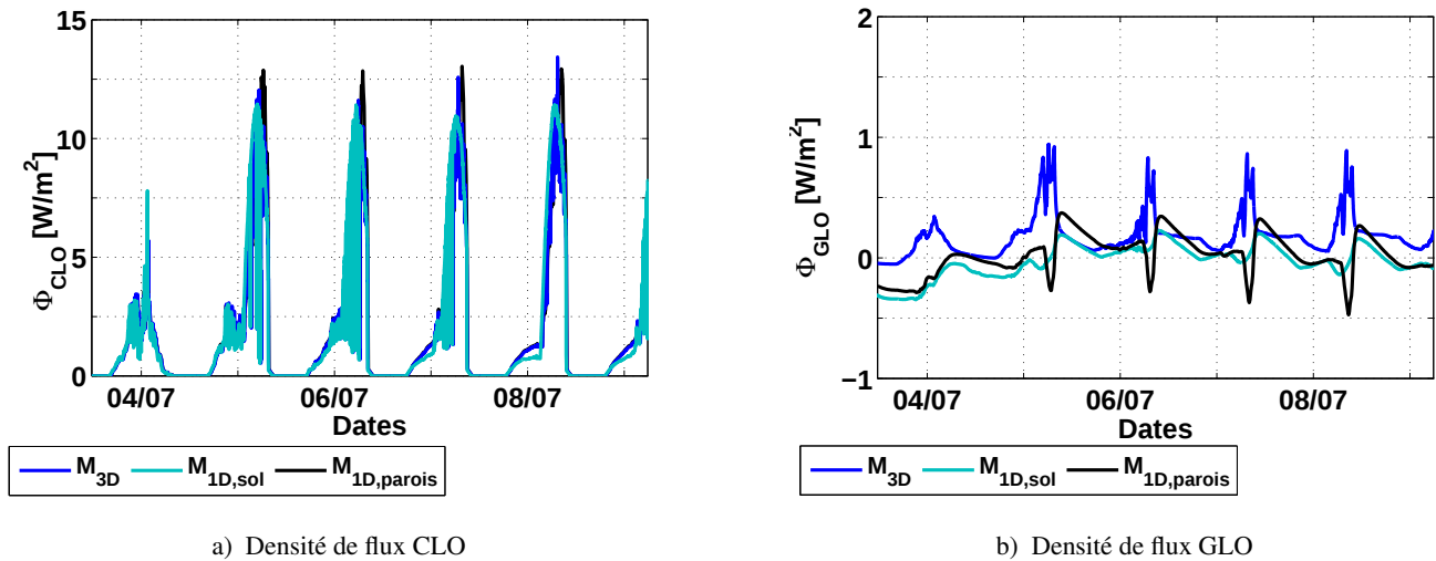
FIGURE IV.16 – Densités de flux radiatifs, moyennées sur l'ensemble des parois de la cellule, calculés avec le modèle 3D et le modèle M_{1D,sol}
