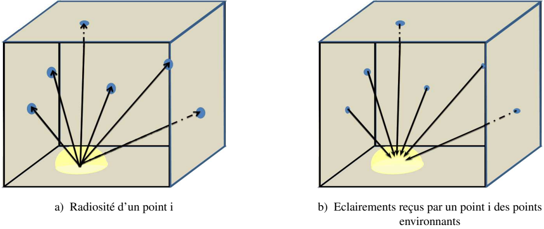
FIGURE II.6 – Radiosit  d'un point i et contribution de l'ensemble des points environnants
