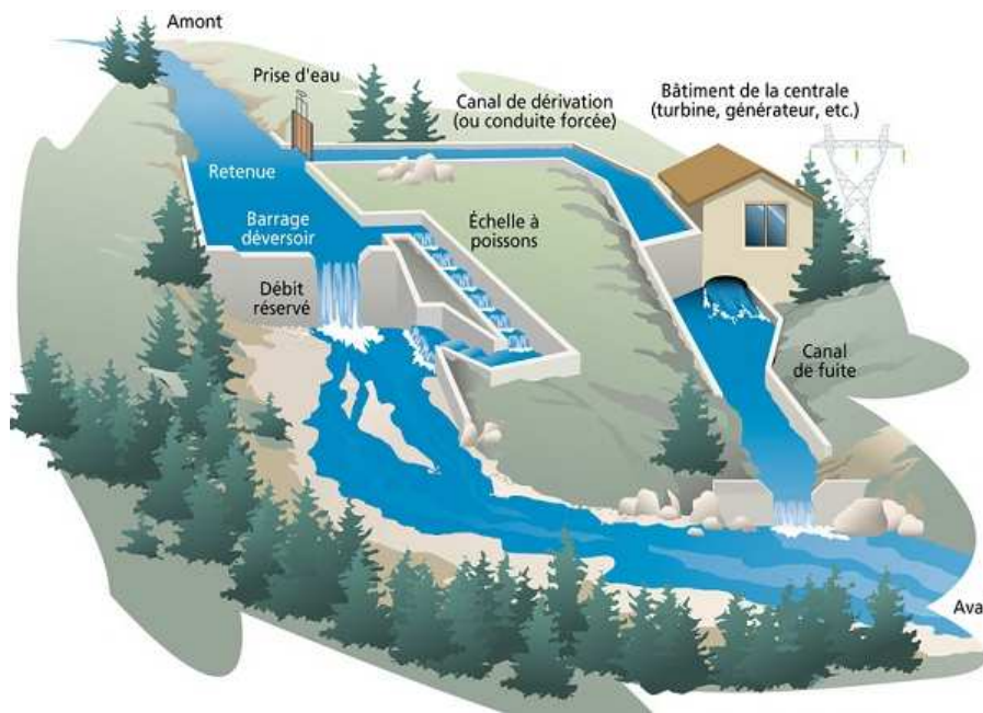
Figure 1. Schéma général du fonctionnement d'une centrale hydroélectrique par écluse. (Source : www.tenergie.fr )
