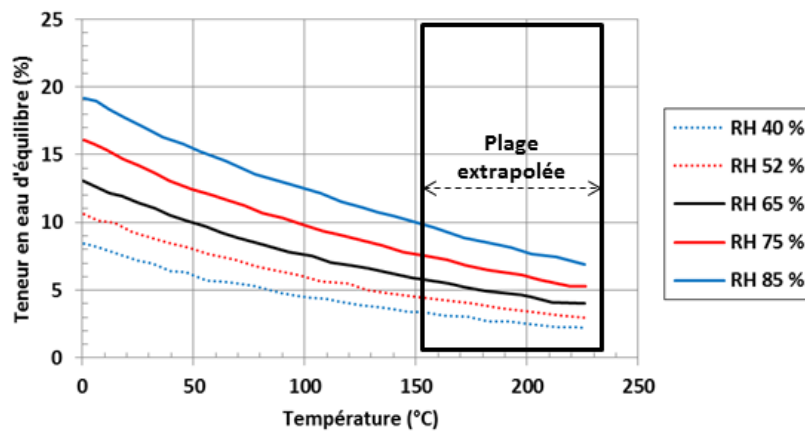
Figure 1.5 – Teneur en eau d'équilibre à différentes humidités relatives en fonction de la température [29].
