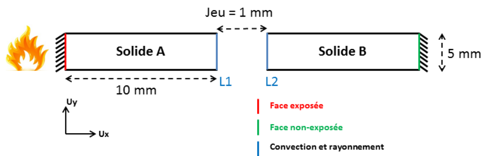
Figure A1.1 : Schématisation du blocage d'un jeu de fonctionnement dans CAST3M ® .
