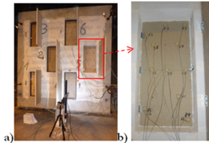
FIG. 3 – a) Vue de la face non-exposée du four d'essai de dimension 3 x 3 m, b) Echantillon de lin d'épaisseur 33,5 mm monté sur paumelles.
