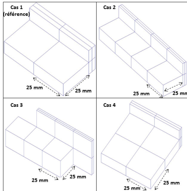
Figure 5.9 – Les différentes configurations de paumelles simulées.
