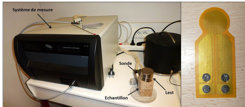
Figure 2.15 – A gauche : exemple de mesure TPS à 20 °C, à droite : la sonde Kapton de diamètre 9,719 mm utilisée.
