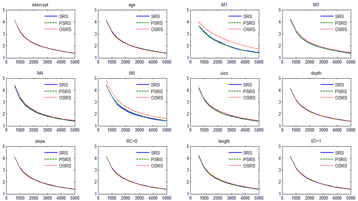
Figure 1-12: moyenne des erreurs types des coefficients estimés vs. taille de l'échantillon, pour les différents facteurs explicatifs présumés, dont : M1: Brick, M2: vitrified clay, M3: clay tile, M4: béton armé, M5: béton, RC : type de rue, ST : type de réseau (1 : unitaire).
