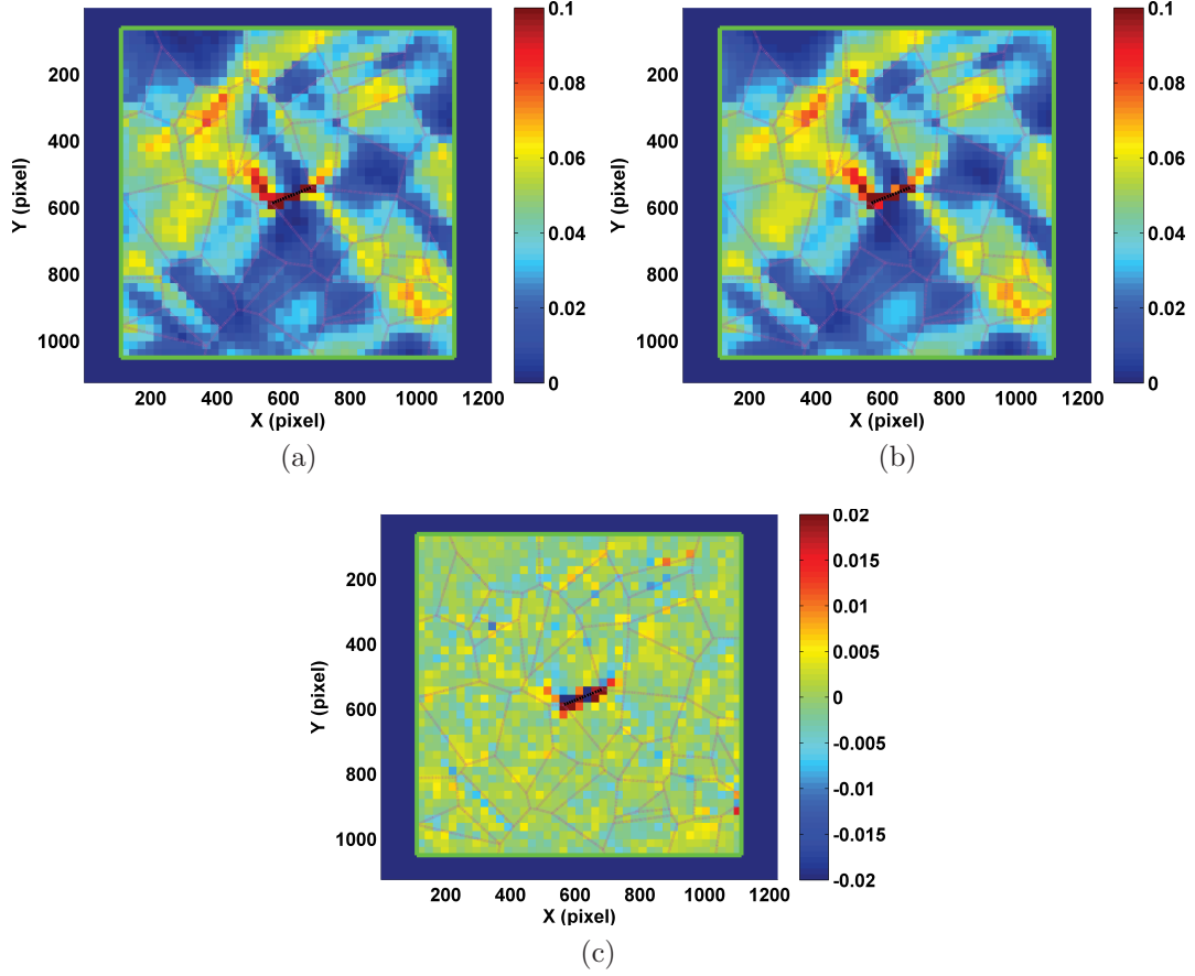
FIGURE 4.17 – Traitement Cinématique I-F : Champ de déformation équivalente moyen par élément \varepsilon_{eq} et \varepsilon_{eq}^{Aster} ainsi que l'erreur de calcul en déformation équivalente
