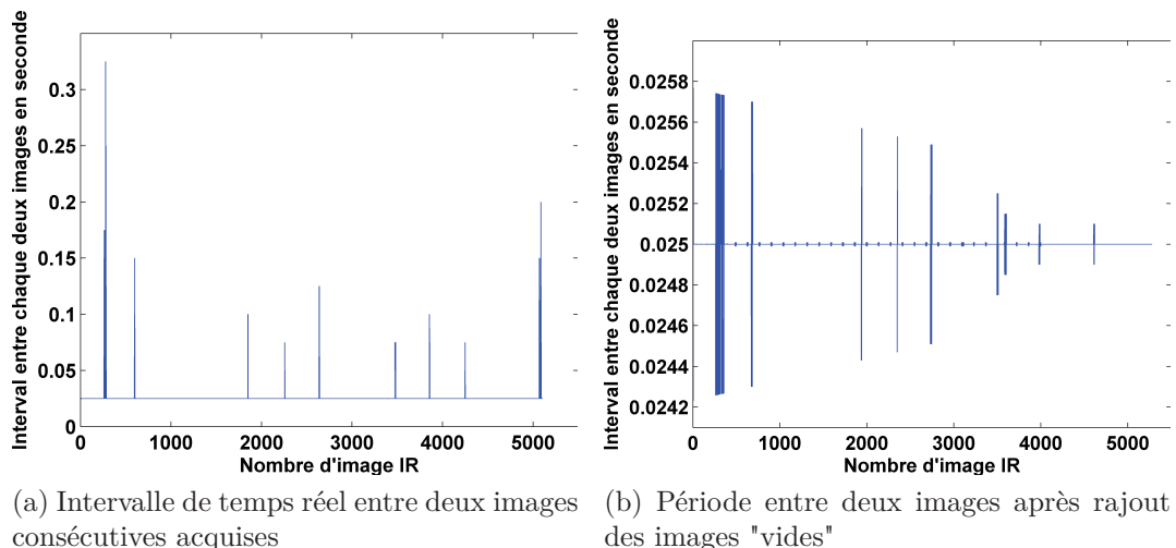
FIGURE 6.2 – Caractérisation des images infrarouges perdues
