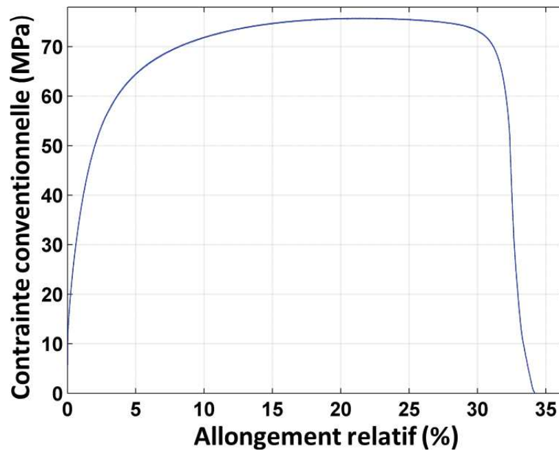
FIGURE 2.8 – Courbe conventionnelle de traction jusqu'à la rupture
