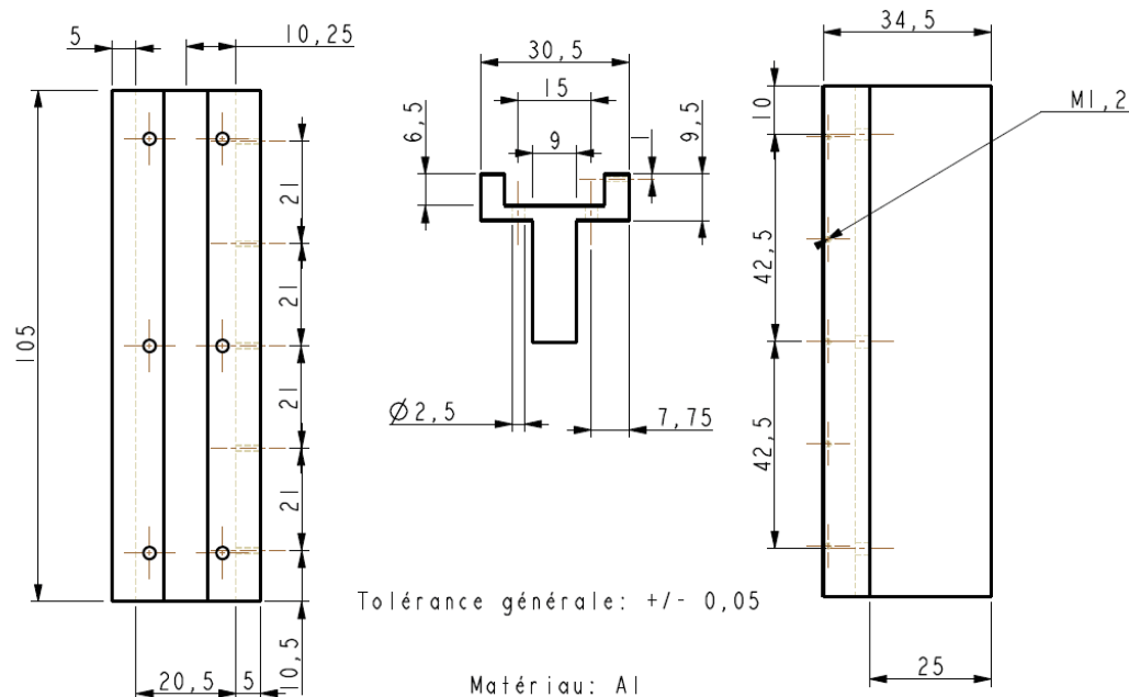
FIGURE 2.10 – Dessin technique du support de l'échantillon (dimensions en \text{mm} )
