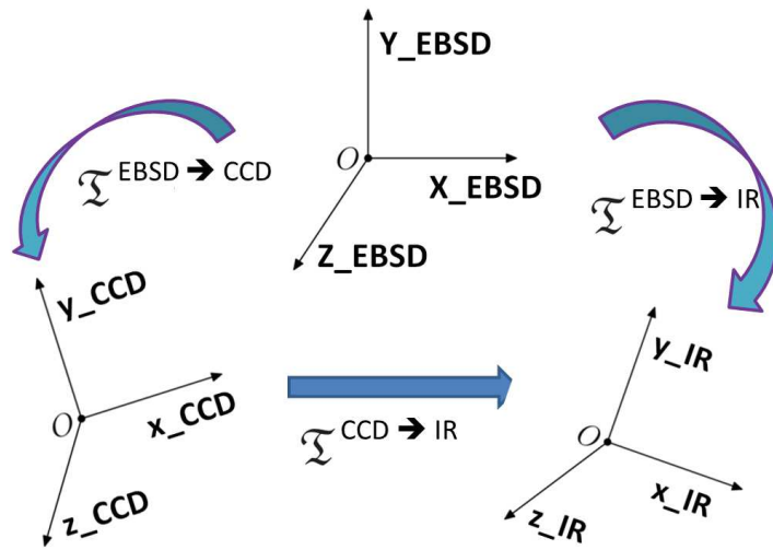
FIGURE 2.26 – Les transformations spatiales parmi les trois repères
