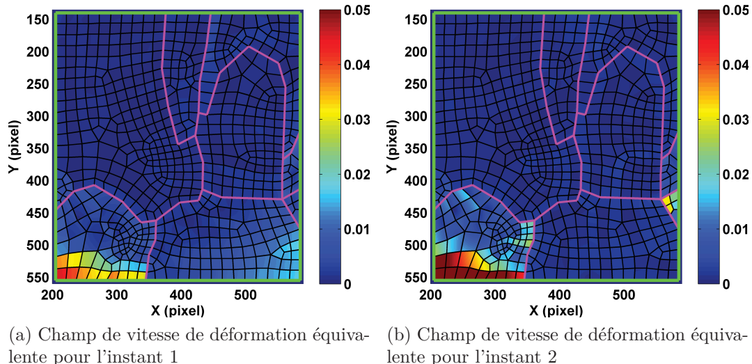
FIGURE 6.20 – Champ de vitesse de déformation équivalente en utilisant une représentation Lagrangienne pour l’instant 1 et 2
