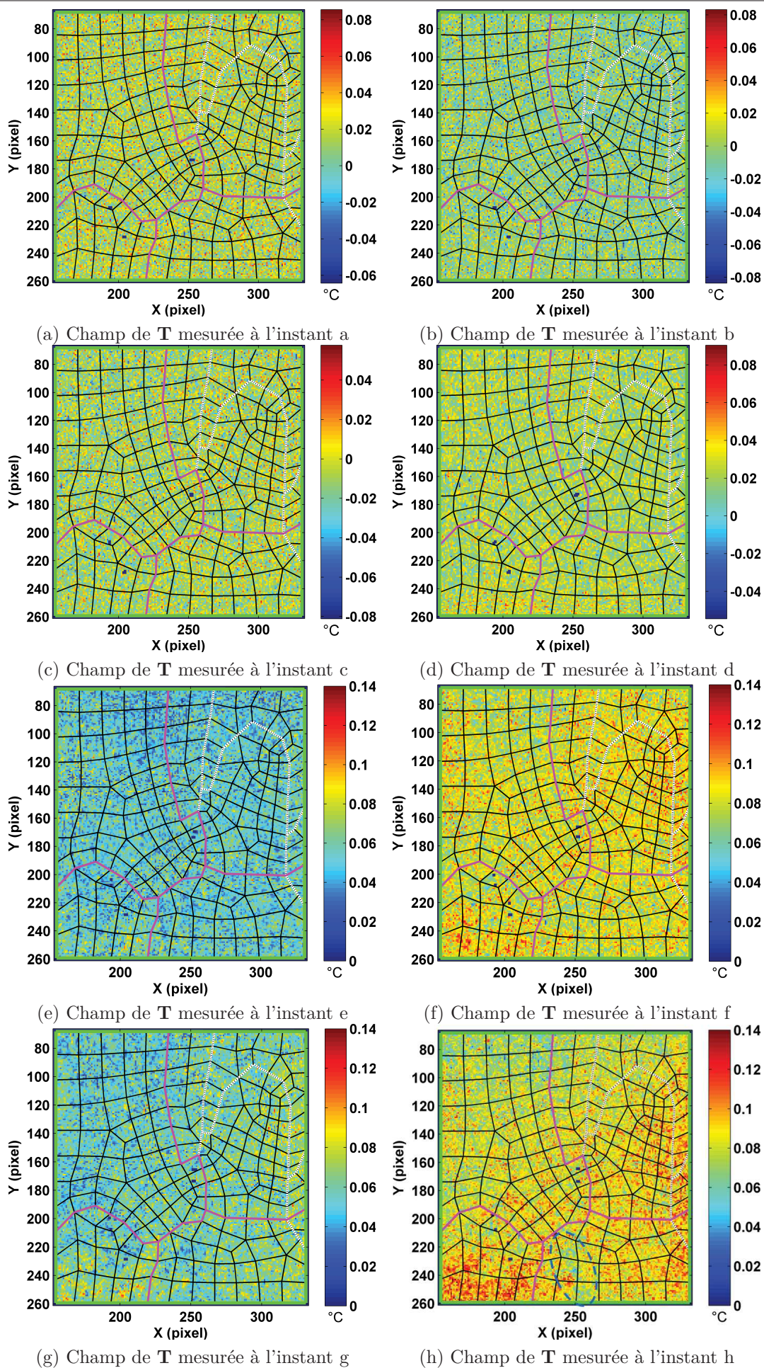
FIGURE 6.27 – Vérification de l'émissivité de l'éprouvette
