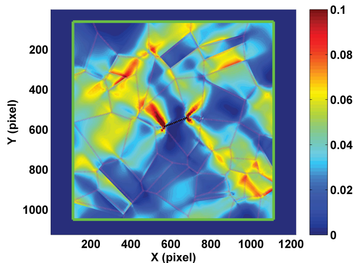
FIGURE 4.6 – Champ de déformation équivalente obtenu par la simulation numérique pour la microstructure fissurée \epsilon_{\text{eq}}^{\text{Aster}}
