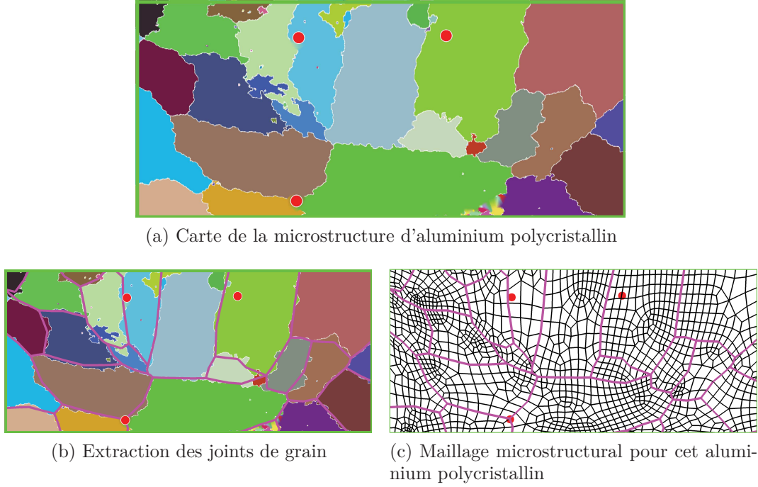
FIGURE 3.12 – Description spatiale de la géométrie d'un agrégat polycristallin
