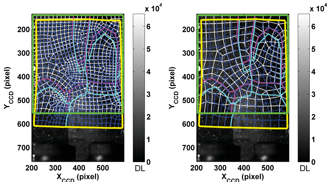
(a) Maillage de calcul CIN dans la configuration Lagrangienne (vert : ZE, magenta : grains et blanc : éléments) et Eulérienne (jaune : ZE, cyan : grain et bleu : élément)
