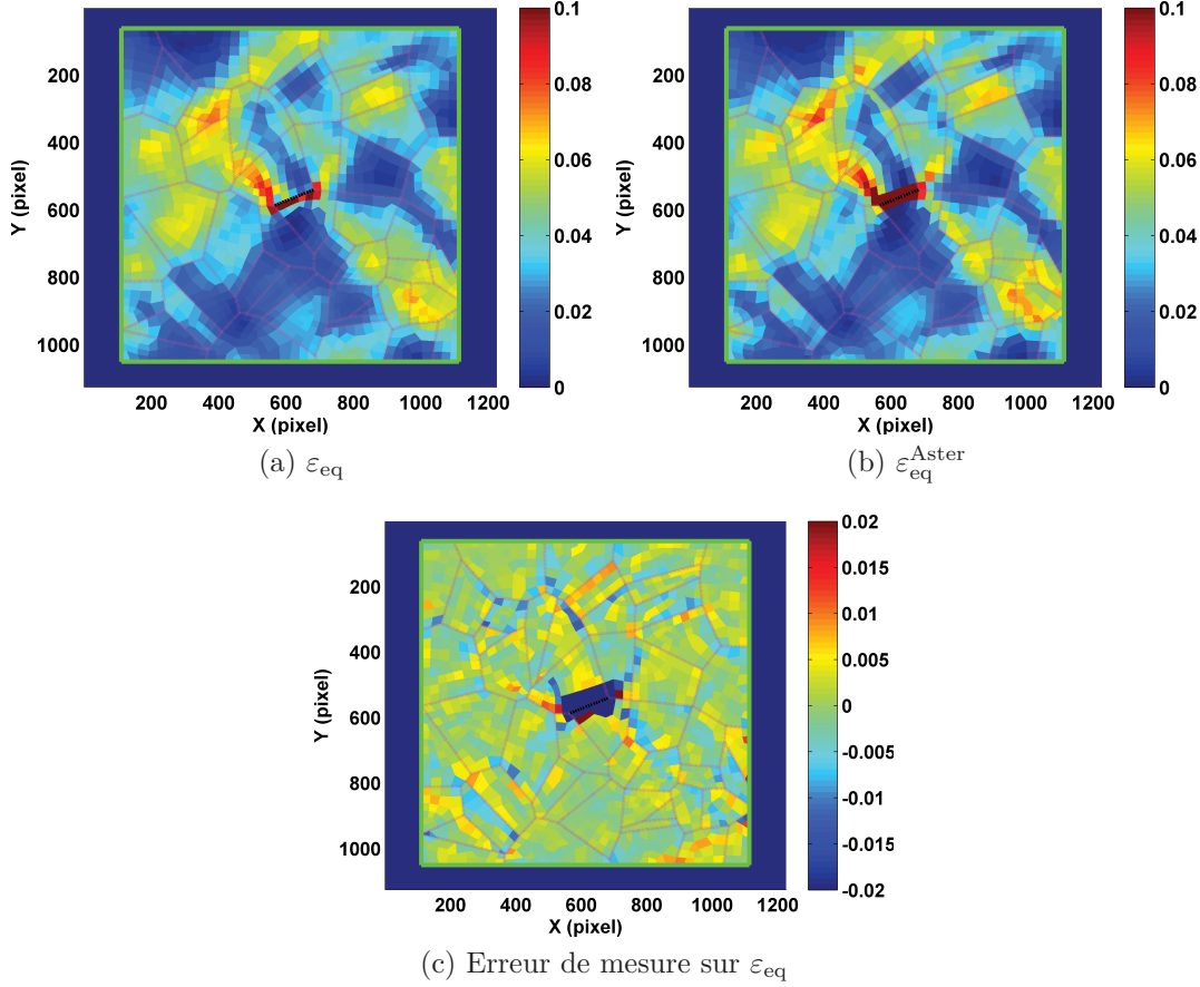
FIGURE 4.26 – Traitement Cinématique IV-F ( Cas 2 ) : Champs de déformation équivalente moyen par élément \varepsilon_{eq} et \varepsilon_{eq}^{\text{Aster}} ainsi que l'erreur de calcul en déformation équivalente
