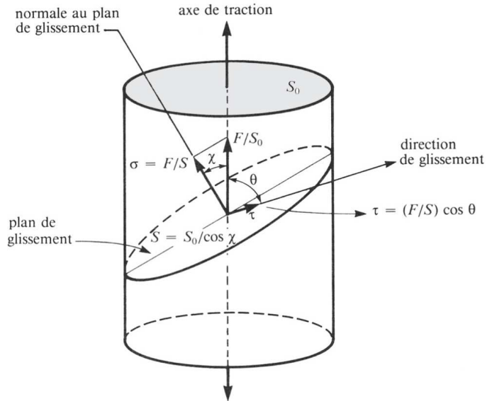
FIGURE 2.15 – Loi de Schmid. Projection de l'effort appliqué sur un plan de glissement et cisaillement résolue \tau dans une direction de glissement.
