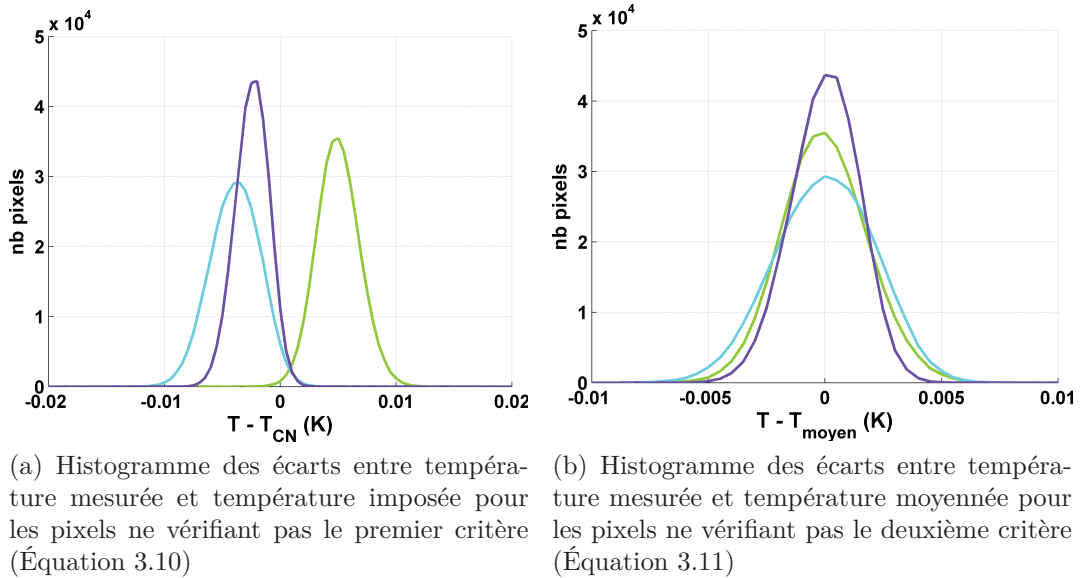
FIGURE 3.5 – Illustration des critères de qualité lors de la procédure d'étalonnage
