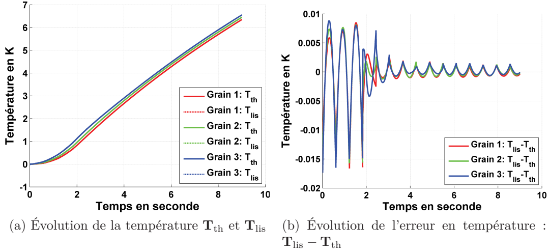
FIGURE 5.11 – Traitement Thermique I : Évolution temporelle de la température moyennée par grain, T_{th} et T_{lis} , ainsi que leurs différences pour les grains 1, 2 et 3
