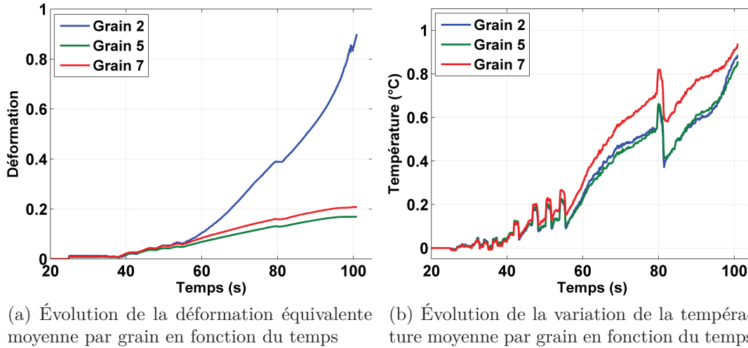
FIGURE 3.11 – Évolutions temporelles de la déformation équivalente par grain et de la variation de la température moyenne par grain [Li et al. , 2013]
