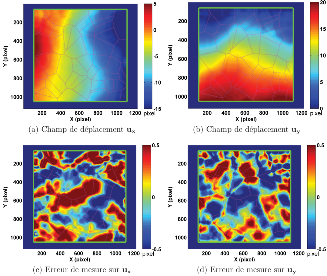
FIGURE 4.12 – Traitement Cinématique II : Champs de déplacements u_x et u_y obtenus par la CIN-E ainsi que l'erreur de mesure par rapport au champ de déplacements simulé u_x^{\text{Aster}} et u_y^{\text{Aster}}
