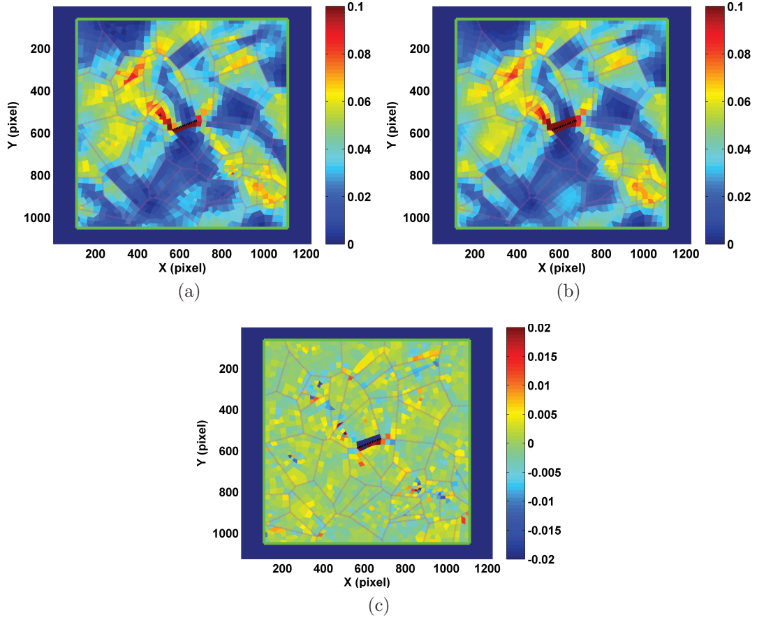
FIGURE 4.19 – Traitement Cinématique II-F : Champs de déformation équivalente moyen par élément \varepsilon_{eq} et \varepsilon_{eq}^{Aster} ainsi que l'erreur de calcul en déformation équivalente
