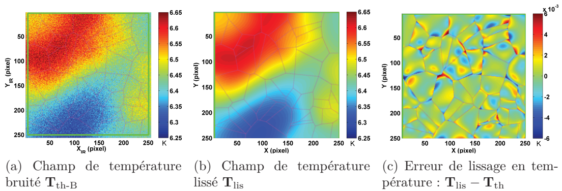
FIGURE 5.13 – Traitement Thermique II : Champ de température obtenu par le traitement d'image thermique ( \mathbf{T}_{lis} ) à partir de l'image bruitée ( \mathbf{T}_{th-B} ) ainsi que la différence par rapport au champ de température théorique ( \mathbf{T}_{th} )
