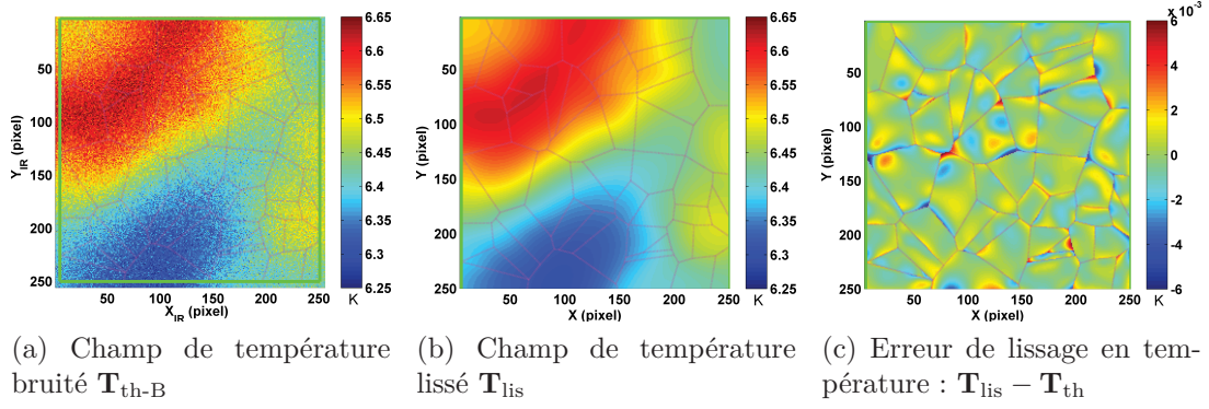
FIGURE 5.19 – Traitement Thermique III : Champ de température obtenu par le traitement d'image thermique ( T_{lis} ) à partir de l'image bruitée ( T_{th-B} ) ainsi que la différence par rapport au champ de température théorique ( T^{th} )
