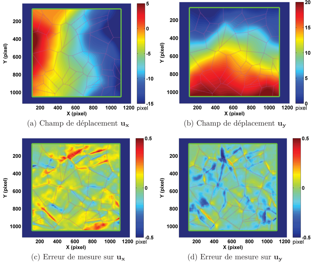
FIGURE 4.14 – Traitement Cinématique III : Champs de déplacements u_x et u_y obtenus par la CIN-E ainsi que l'erreur de mesure par rapport au champ de déplacements simulé u_x^{Aster} et u_y^{Aster}
