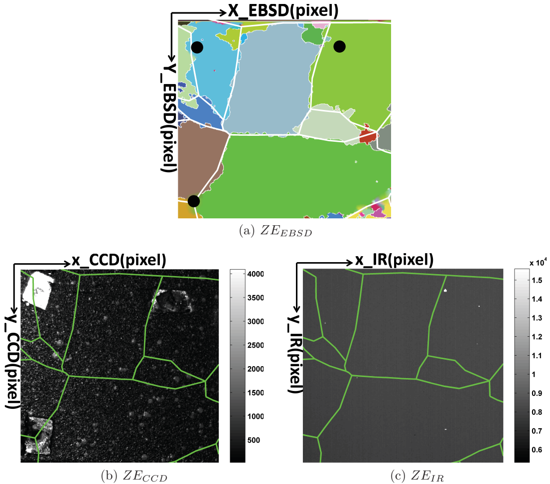
FIGURE 2.27 – Représentation Lagrangienne de la zone d'étude ( ZE ) dans les différents systèmes des coordonnées
