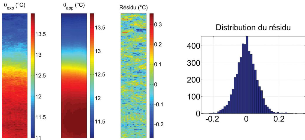
FIGURE 3.9 – Exemple d'un lissage de température avec l'historgramme du résidu (Moyenne \approx 5.10^{-4} °C, Ecart-type \approx 0.06 °C) [Blanche, 2012]
