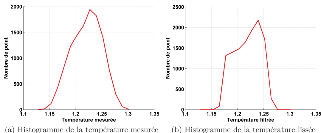
FIGURE 6.32 – Histogramme des grandeurs thermiques pour le grain 1 à l'instant C
