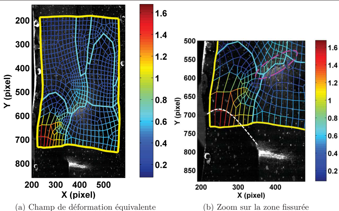
FIGURE 6.19 – Champ de déformation équivalente en utilisant une représentation Eulérienne pour l’instant 2 ainsi que le zoom sur la zone de fissuration
