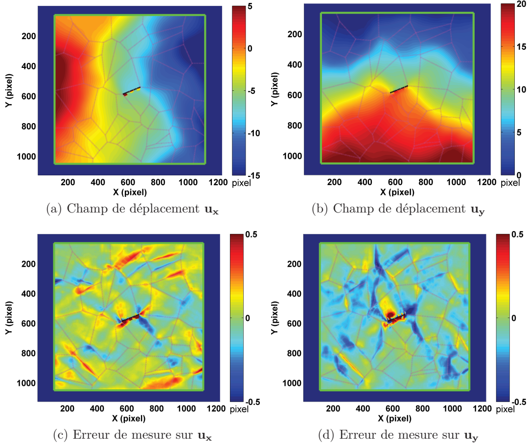
FIGURE 4.24 – Traitement Cinématique IV-F (Cas 2) : Champs de déplacements u_x et u_y obtenus par CIN-E ainsi que l’erreur de mesure par rapport au champ de déplacements simulé u_x^{\text{Aster}} et u_y^{\text{Aster}}
