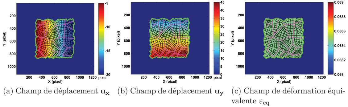
FIGURE 4.33 – Champs cinématiques homogènes imposés pour l'étude de déformation homogène sur l'image réduite
