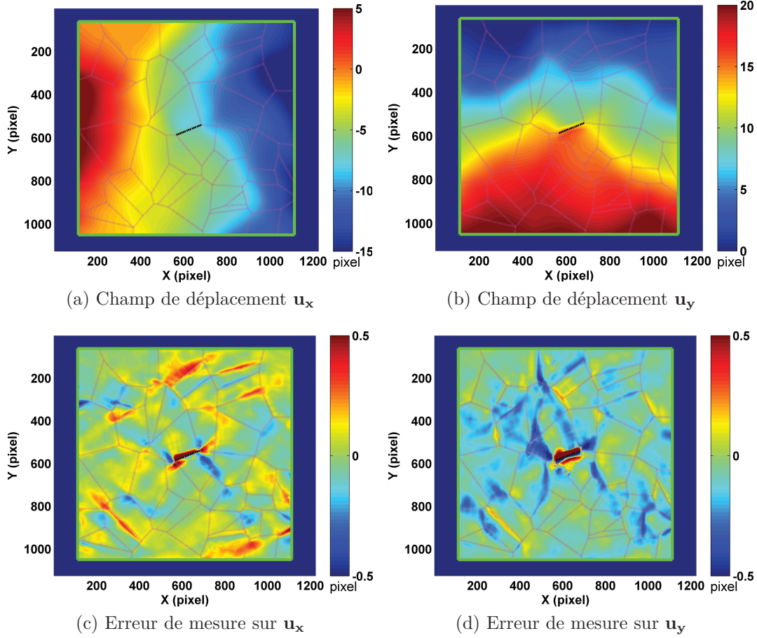
FIGURE 4.23 – Traitement Cinématique IV-F ( Cas 1 ) : Champs de déplacements u_x et u_y obtenus par CIN-E ainsi que l'erreur de mesure par rapport au champ de déplacements simulé u_x^{\text{Aster}} et u_y^{\text{Aster}}
