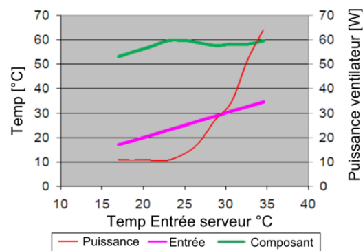
Figure 12 : Consommation d'un ventilateur en fonction d'une rampe de température à l'entrée d'un serveur
