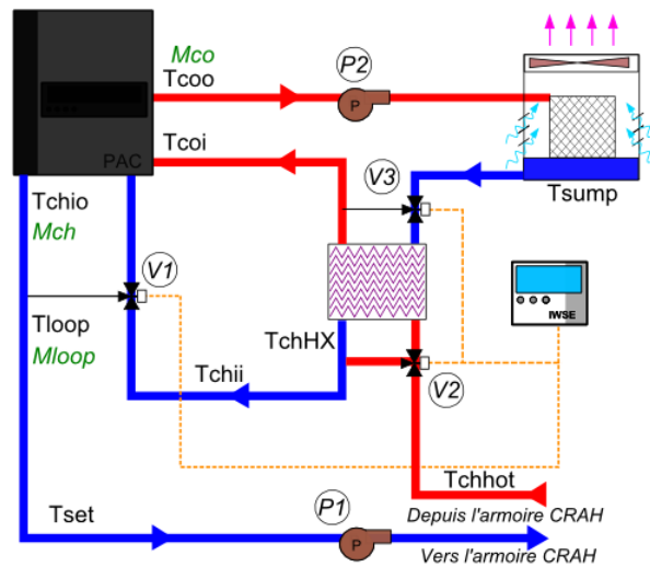
Figure 135 : fonctionnement du système en mode TFC
