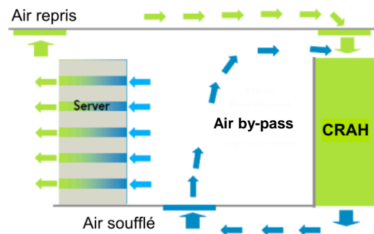
Figure 19 : phénomène de by-pass
