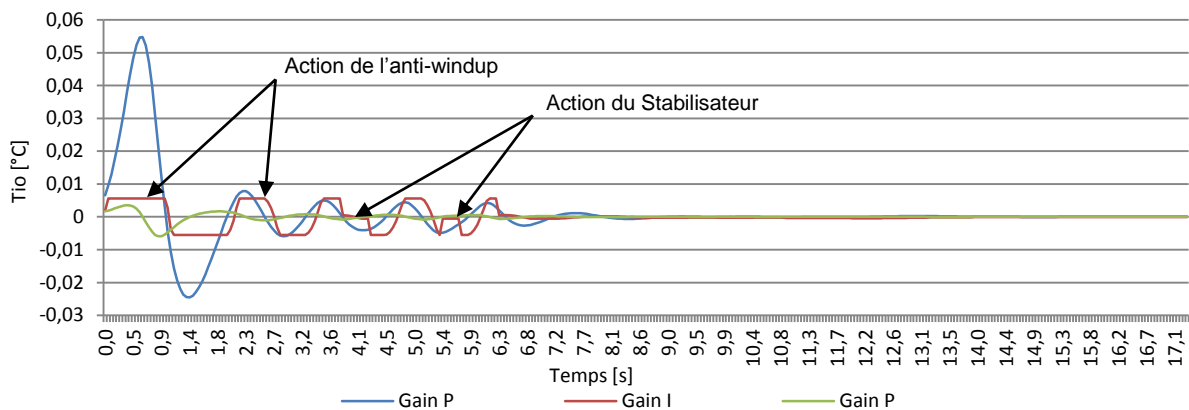
Figure 88 : visualisation des Erreur P_c , I_c , D_c
