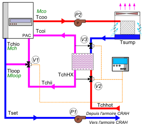
Figure 136 : fonctionnement du système en mode PFC
