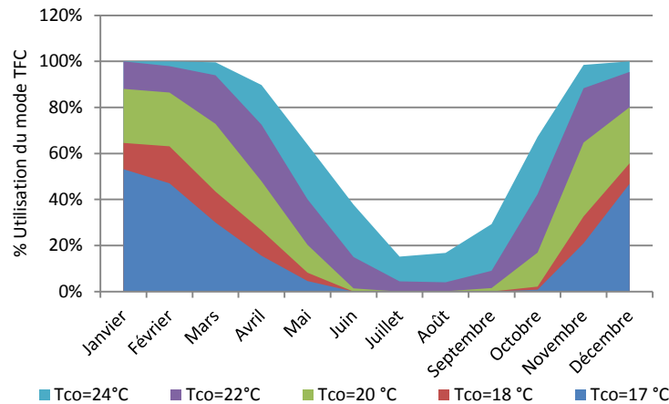
Figure 151 : % utilisation du mode TFC
