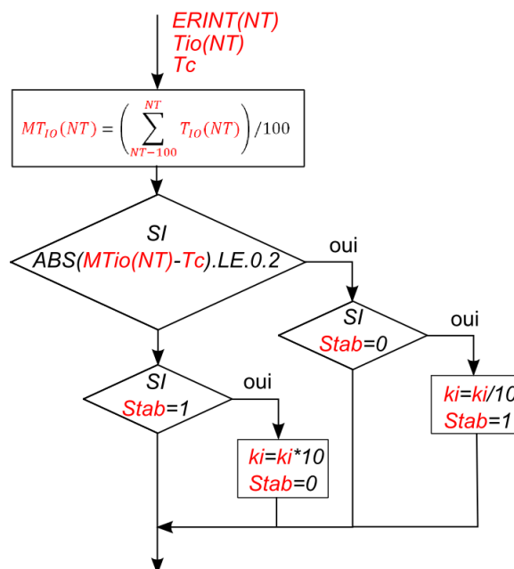
Figure 86 : Algorithme stabilisateur du PID
