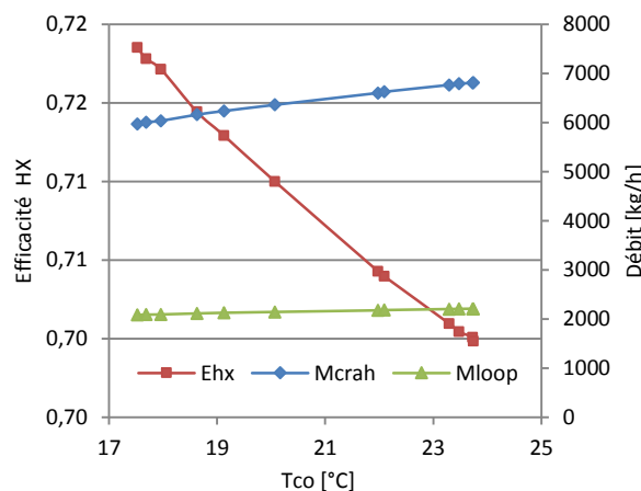
Figure 148 : évolution de \epsilon_{HX} en fonction de T_{CO}
