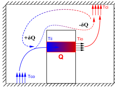
Figure 24 : transfert d'énergie allée chaude allée froide
