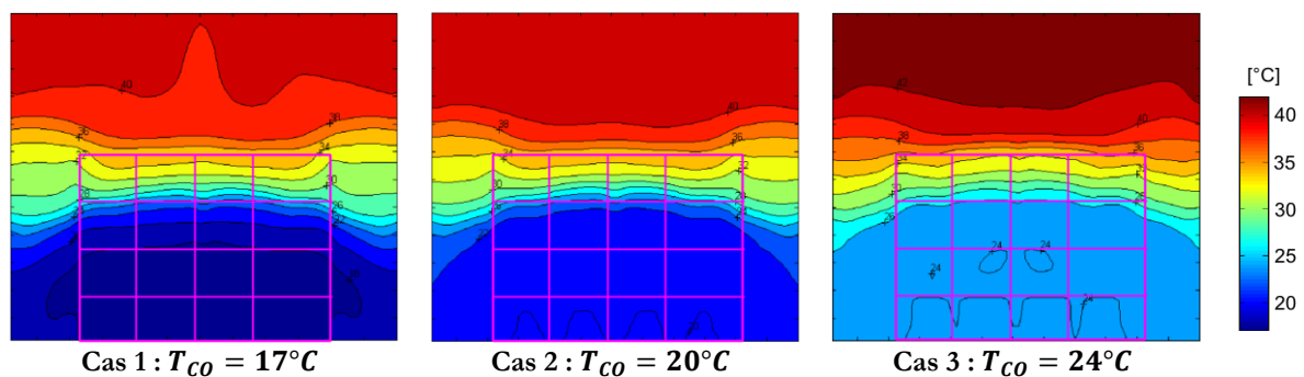
Figure 146 : Champs de température pour 3 valeurs de T_{CO}
