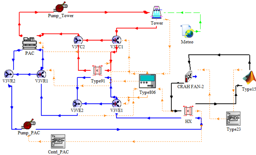
Figure 138 : Implantation du système IWSE dans TRNSYS
