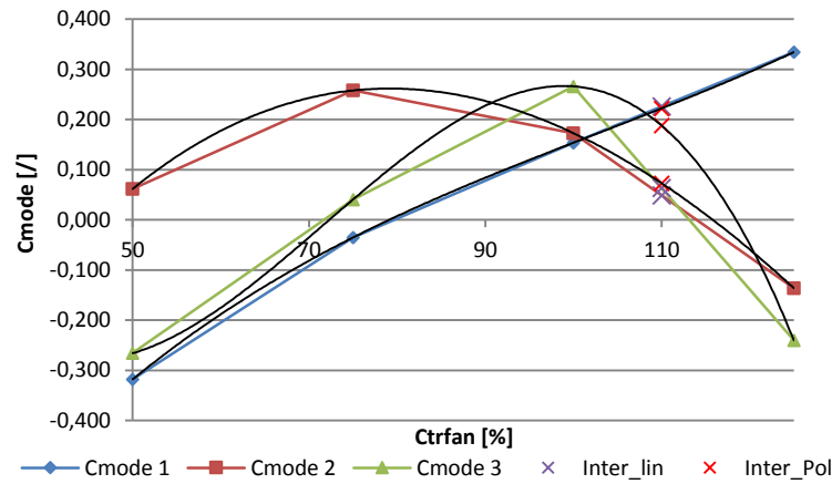
Figure 111 : Evolution de Cmode en fonction de Ctrfan pour T_{co}=18,67^\circ\text{C}
