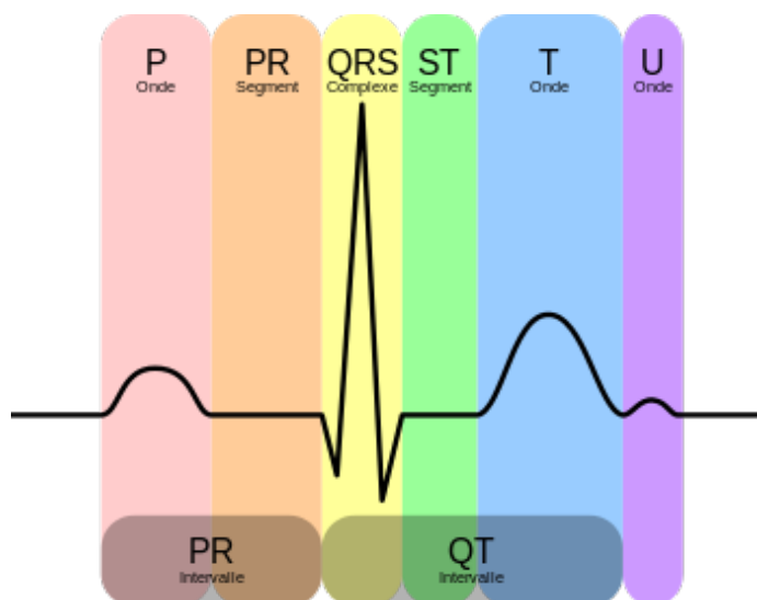
Figure 3 : Représentation d'un ECG normal 1 .
