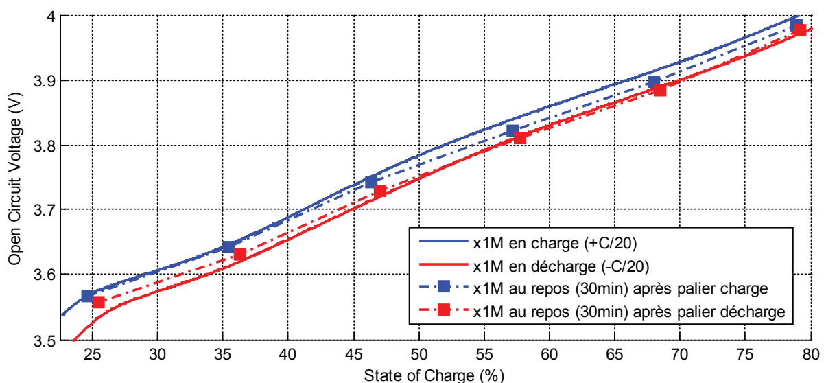
Figure II.8 – Comparaison de tracés OCV à 25\text{ °C} édités à partir de tensions de repos de 30 minutes vs ceux issus de mesures continues à très faible courant
