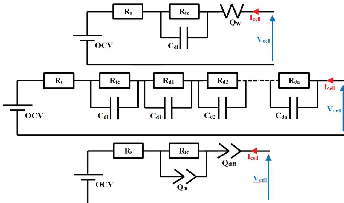
Figure I.19 – Exemples de modèles électriques tenant compte des effets de diffusion
