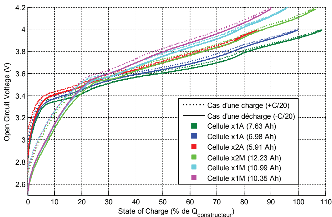
Figure II.13 – Tension à C/20 en fonction du SoC pour deux types de cellules Li-ion à différents états de vieillissement (à 25 °C) – Capacité constructeur considérée comme référence
