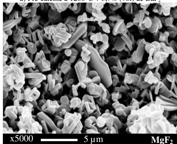
c) Pré-calciné à 1200°C + 4,5% (vol) de MgF 2
