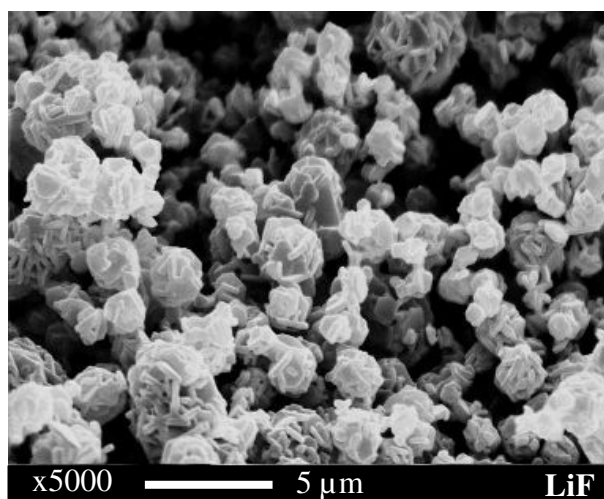
e) Pré-calciné à 1200°C + 4,1% (vol) de LiF
