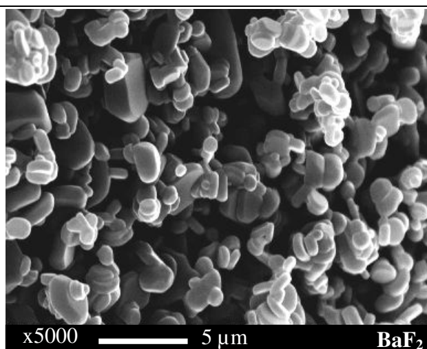
a) Pré-calciné à 1200°C + 3,7% (vol) de BaF 2
