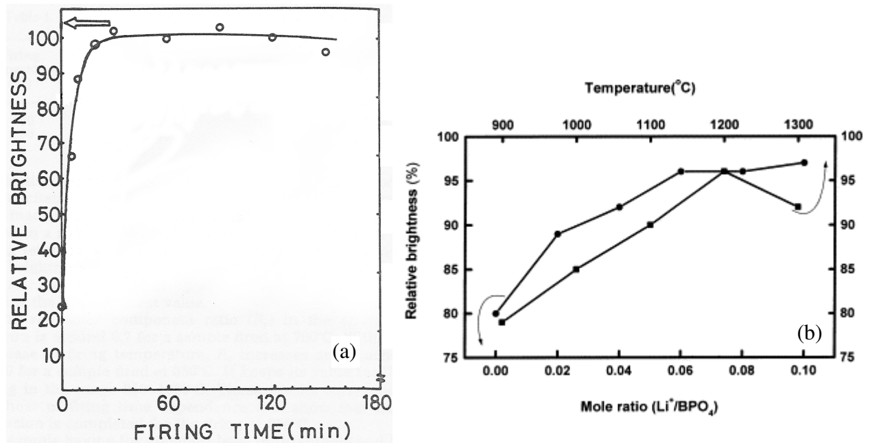
Fig. I.22. (a) Brillance relative d'Y 2 O 2 S :Eu calciné à 1180°C en fonction de la durée de palier [I39] et (b) brillance relative de La(BO 3 ,PO 4 ) : Ce, Tb, Gd en fonction de la température de calcination et de la quantité de fondant ajouté [I40].
