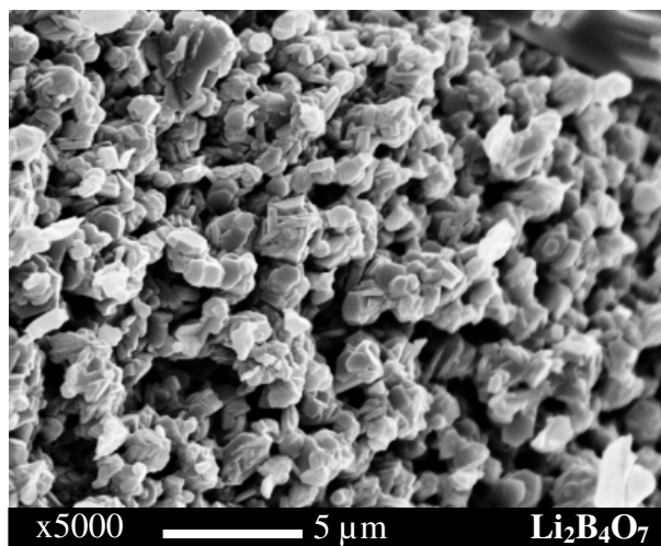
d) Pré-calciné à 1200°C + 2,9% (vol) de Li 2 B 4 O 7
