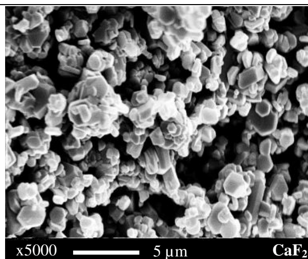
b) Pré-calciné à 1200°C + 4,3% (vol) de CaF 2
