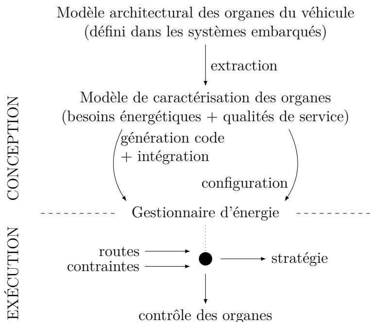
FIGURE 2.1 – Méthodologie du canevas logiciel ORQA.
