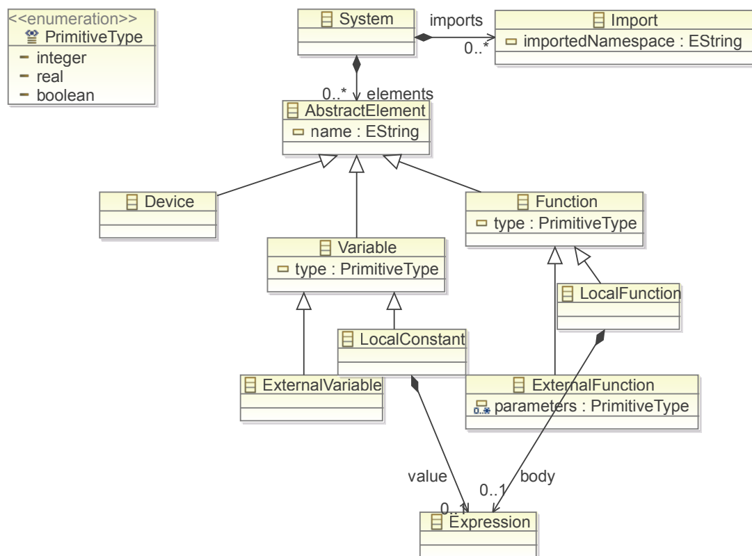
FIGURE 3.1 – Vue graphique du métamodèle Ecore de la caractérisation des organes consommateurs d'un véhicule.
