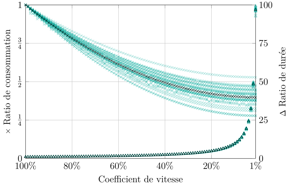
FIGURE 2.8 – Exemple de simplification des ratios des résultats de durée et de consommation. Les ratios approximés sont en noir.
