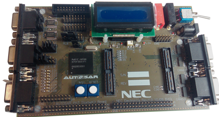
FIGURE 4.3 – La plate-forme d'évaluation NEC V850E/PHO3.
