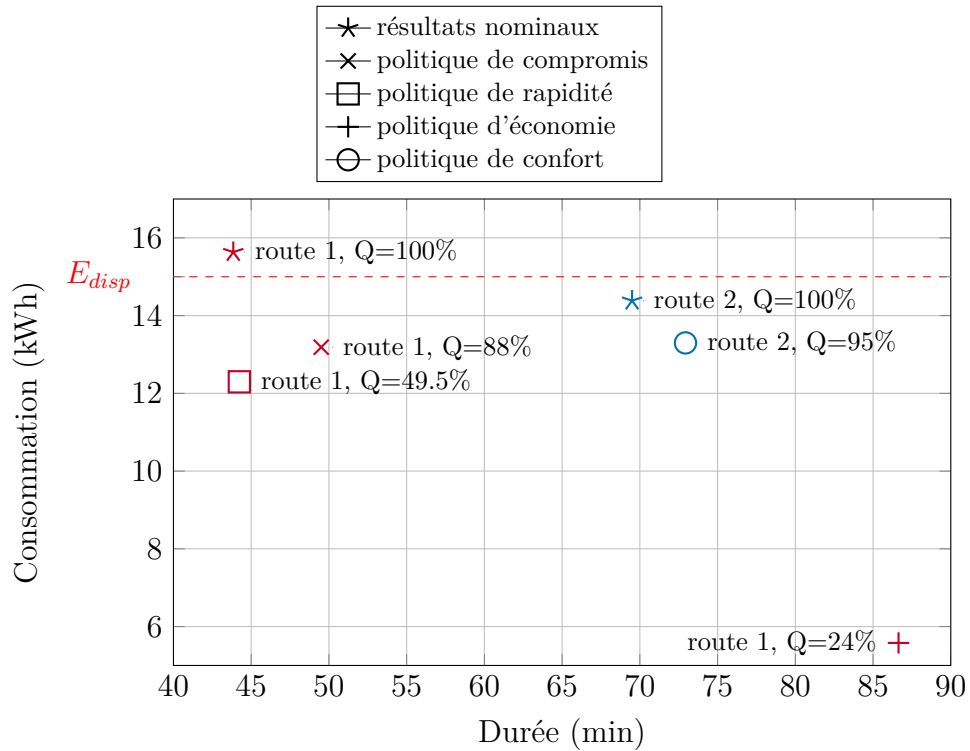
FIGURE 4.6 – Résultats des stratégies de conduite optimales du véhicule polyvalent pour le scénario Sa .
