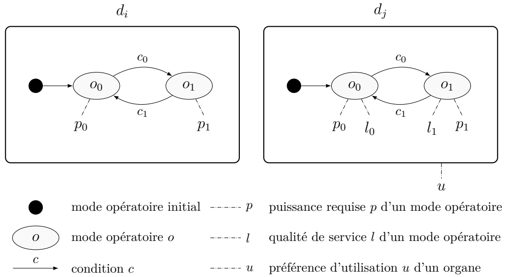
FIGURE 2.4 – Exemple de modélisation de deux organes consommateurs. L'organe d_i est observable et l'organe d_j est contrôlable.
