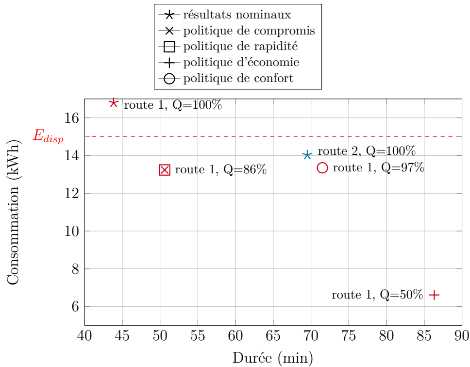
FIGURE B.1 – Résultats des stratégies de conduite optimales du véhicule urbain pour le scénario Sa .
