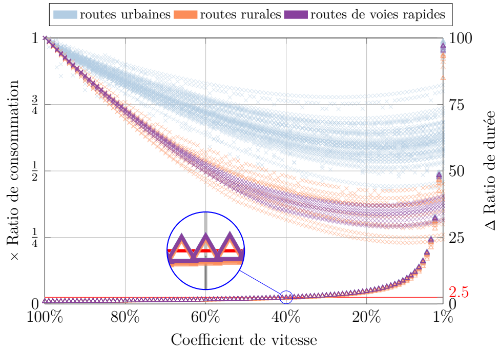
FIGURE 4.4 – Évolution des ratios des résultats de durée et de consommation du véhicule urbain.
