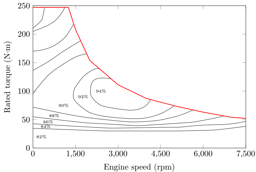
FIGURE 3.2 – Cartographie de l'efficacité d'un moteur électrique de berline en fonction de la vitesse angulaire du moteur et du couple demandé.
