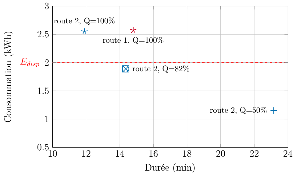
FIGURE 4.7 – Résultats des stratégies de conduite optimales du véhicule urbain pour le scénario Sb .
