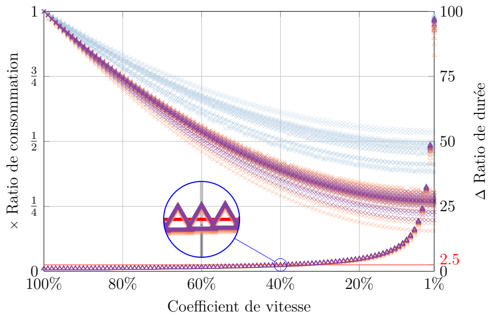
FIGURE 4.5 – Évolution des ratios des résultats de durée et de consommation du véhicule polyvalent.
