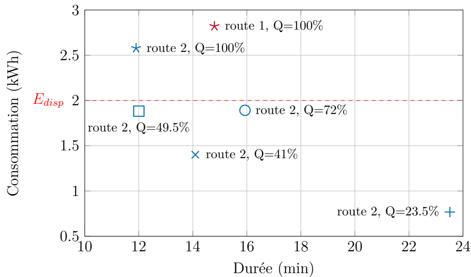
FIGURE B.2 – Résultats des stratégies de conduite optimales du véhicule polyvalent pour le scénario Sb .
