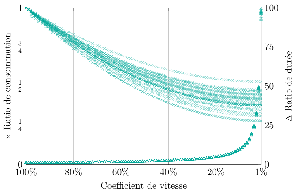
FIGURE 2.6 – Évolution des ratios des résultats de durée (triangles) et de consommation (croix).
