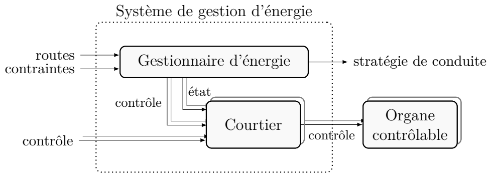
FIGURE 2.9 – Architecture logicielle du système de gestion d'énergie.
