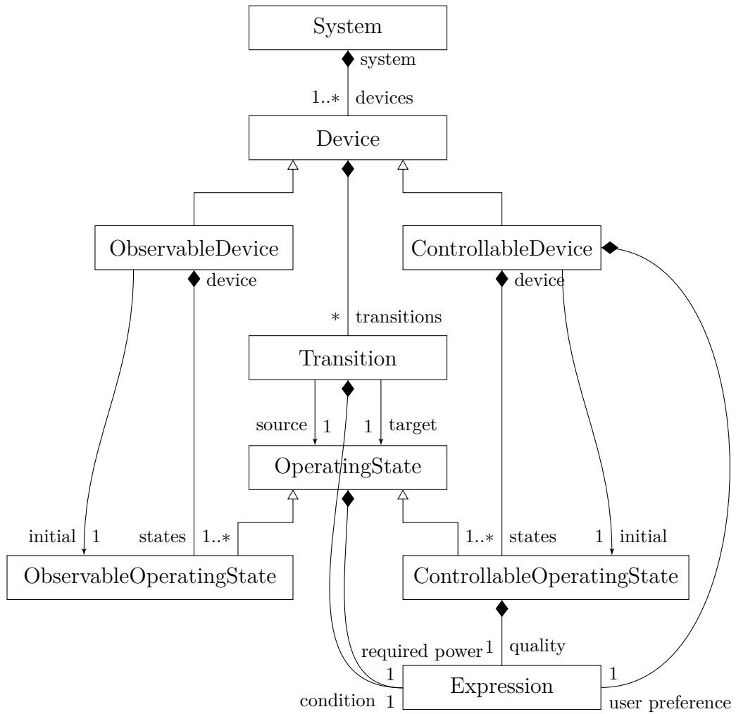
FIGURE 2.2 – Métamodèle de caractérisation des organes consommateurs d’un véhicule.
