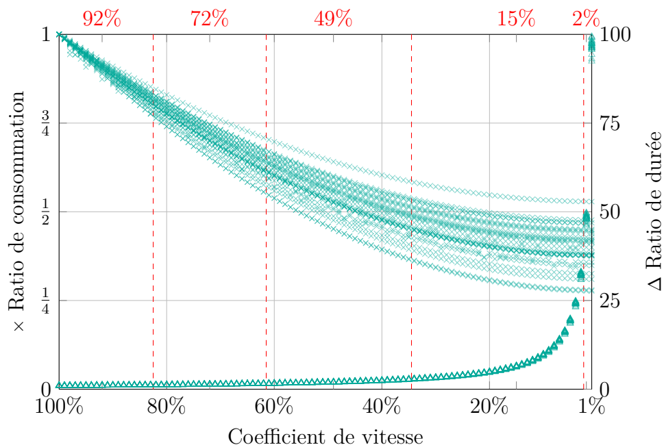
FIGURE 2.7 – Exemple de partitionnement des ratios des résultats de durée et de consommation. Les différentes partitions sont séparées par les lignes verticales pointillées ; les coefficients de vitesse correspondants sont indiqués en partie haute.
