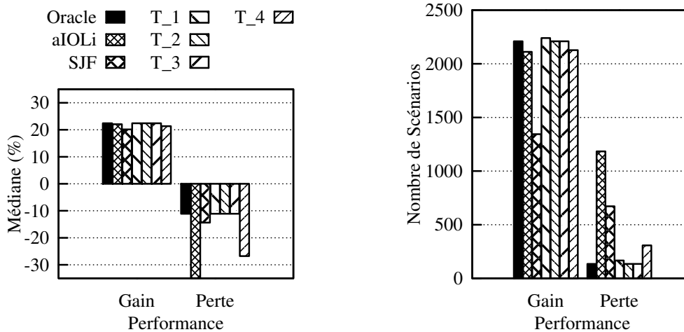
(a) Différences de performance (médiane) (b) Situations avec des différences de performance FIGURE B.5: Résultats de performance pour les arbres de sélection de l'algorithme d'ordonnancement en utilisant la spatialité et la taille des demandes détectées automatiquement.
