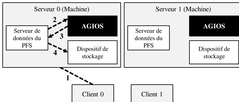
FIGURE B.2: Illustration de l'interface entre AGIOS et un serveur de données d'un système de fichiers parallèle.
