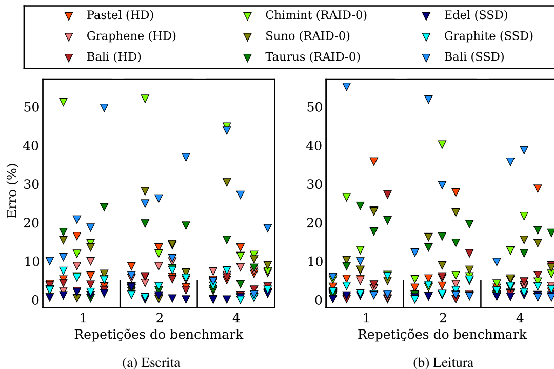
Figura C.4: Erro absoluto induzido pelo uso da SeRRa para obter a razão entre acessar sequencialmente ou aleatoriamente.
