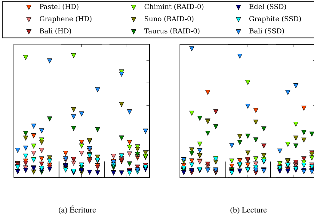
FIGURE B.4: Erreur absolue induite par l'utilisation du SeRRa pour obtenir le ratio de débit séquentiel et aléatoire.
