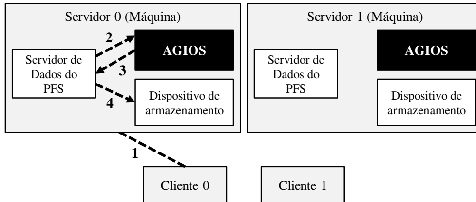
Figura C.2: Ilustração da interface entre AGIOS e um servidor de dados de um sistema de arquivos paralelo.
