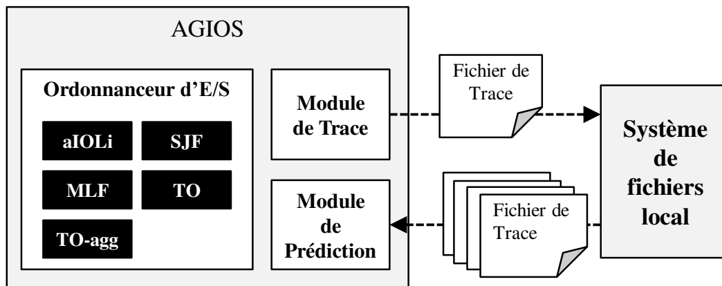
FIGURE B.3: L'architecture de l'outil AGIOS.
