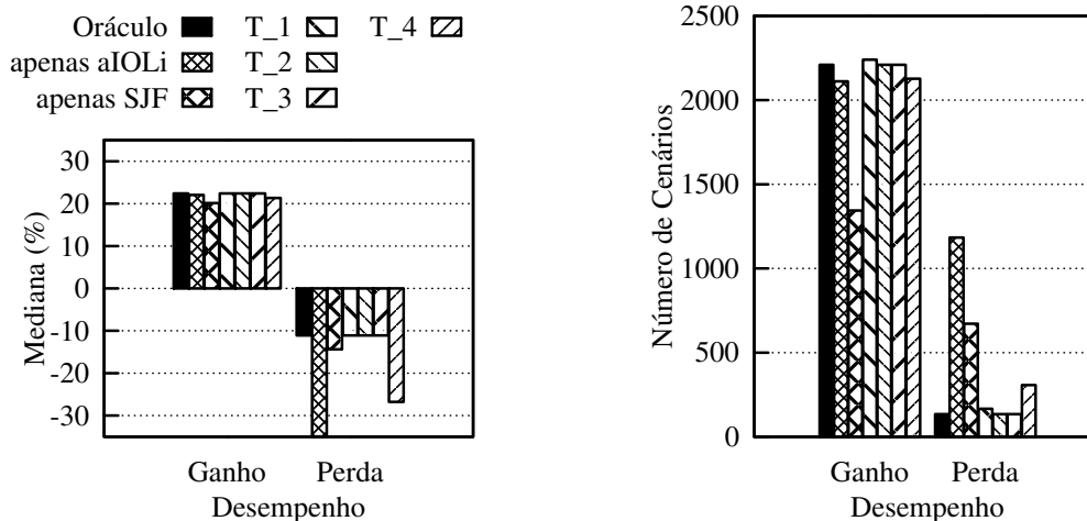
(a) Diferenças medianas de desempenho (b) Situações com diferenças de desempenho Figura C.5: Resultados de desempenho para as árvores de seleção de algoritmo de escalonamento usando espacialidade e tamanho de requisições detectados.
