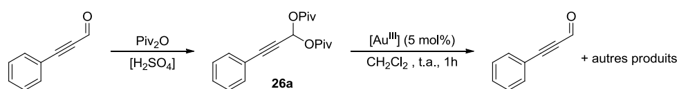
Schéma 165 : Régression à l'aldéhyde initial en catalyse à l'or(III)
