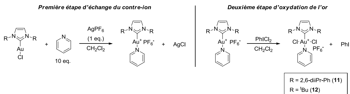
Schéma 145 : Synthèse des complexes NHC-Au III (py) 11 et 12
