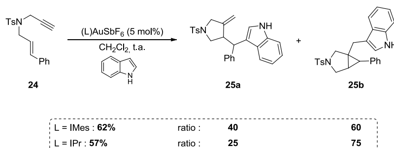
Schéma 162 : Sélectivités de différents carbènes dans l'addition d'indole sur des 1,6-énynes 24
