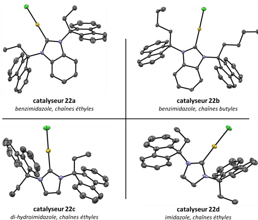
Schéma 157 : Structures DRX correspondants aux complexes NHC(fluorényl)-Au I 22a-d
