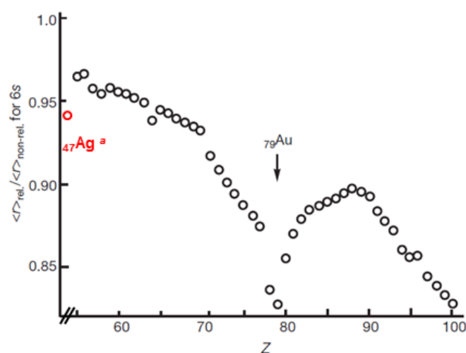
Schéma 6 : Rayon relativiste de l'orbital 6s par rapport au rayon non relativiste en fonction de Z ( a valeur calculée pour l'orbitale 5s dans le cas de l'argent) 12
