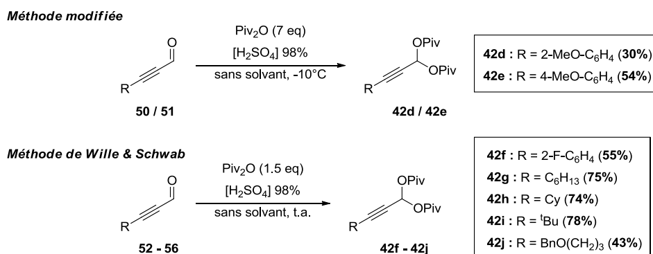
Schéma 102 : Synthèse des différents gem -dipivalates propargyliques
