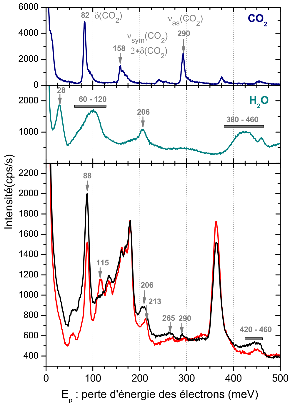
FIGURE 4.3.3 : Spectres de pertes d'énergie ( E_0 = 6 \text{ eV} ; \Delta E_{\text{FWHM}} \approx 6 \text{ meV} ) avant et après une irradiation de 5 heures à 1 eV à 28 K sur un échantillon d'une SAM de MUA acide (dose : N_{e^-} reçus par la surface = 2,1 \times 10^{16} ). Les deux autres spectres en bleu sont respectivement ceux de glaces multicouches d'eau et de dioxyde de carbone pures condensées sur une plaque d'or [45].
