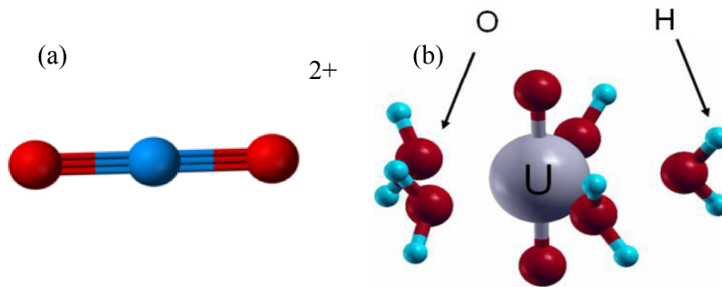
Figure 2 : (a) Ion uranyle et (b) sphère de solvation (Roques et al. , 2009)
