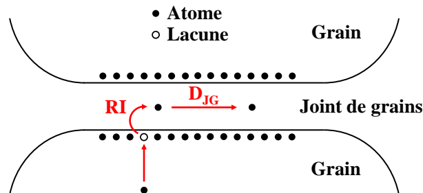
Figure A.9 – Représentation du mécanisme de réaction d'interface (RI) en série avec la diffusion aux joints de grains ( D_{JG} ) au niveau d'un pont entre deux grains
