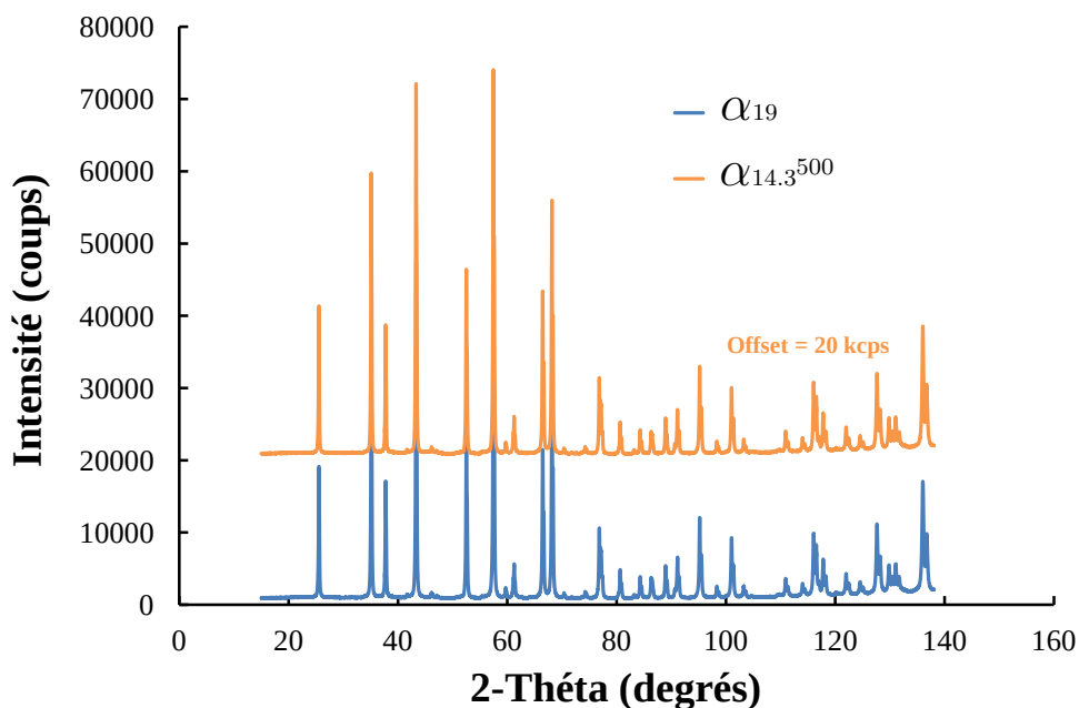
Figure B.7 – Diffractogrammes des poudres principales d'alumine \alpha
