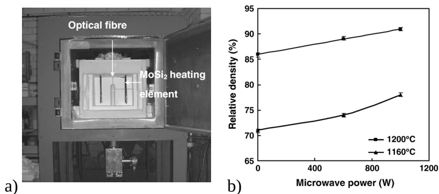
Figure A.40 – a) photographie du four de frittage micro-ondes hybride, b) variation de la densité relative des films à différentes températures en fonction de la puissance des micro-ondes selon Wang et al. [65]
