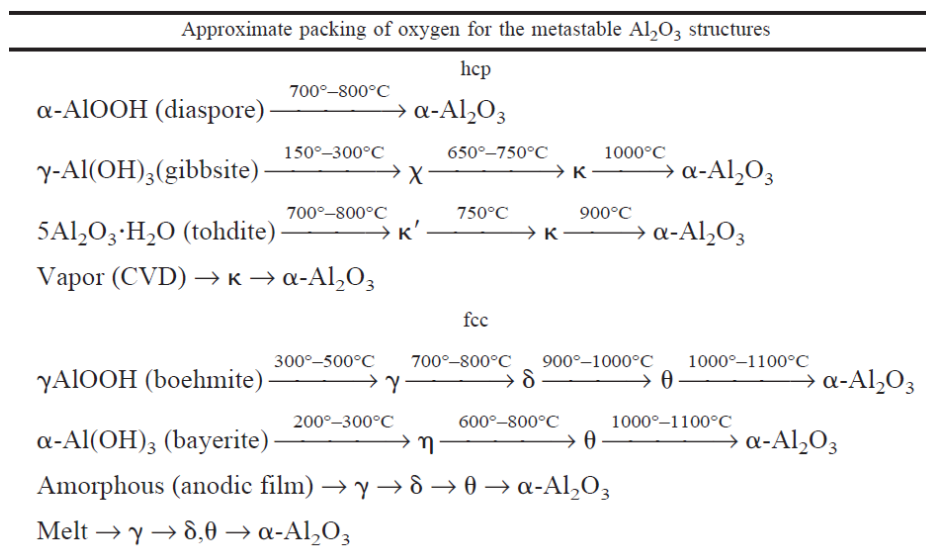
Figure A.23 – Séquences de transformation des alumines de transition cristallisant dans un empilement hexagonal compact (hcp) et cubique faces centrées (fcc) [33]
