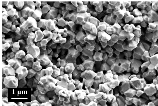
Figure D.24 – Fractographie au cœur de l'échantillon d'alumine \alpha_{6^{500}} fritté par FMD à 25°C/min avec un palier de 5 min à 1550°C, de densité relative 0,8 (la taille des grains correspond à la taille moyenne mesurée sur les différentes zones analysées)
