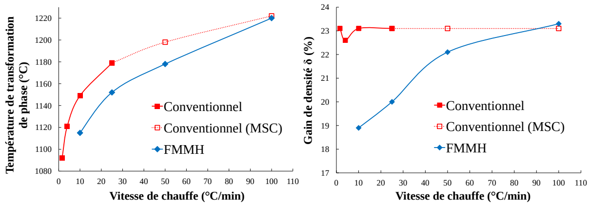
Figure D.36 – Comparaison de la température et du gain de densité \delta de la transformation de phase de la poudre \gamma_{954}^{500} aux vitesses de chauffe de 10, 25, 50 et 100°C/min en frittage conventionnel et FMMH
