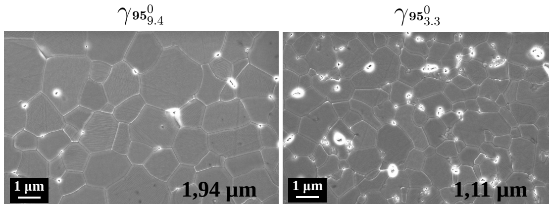
Figure B.41 – Micrographies au cœur des échantillons d'alumine \gamma_{953.3} et \gamma_{959.4} frittés à 25°C/min jusqu'à 1550°C pendant 5 min (la taille des grains correspond à la taille moyenne mesurée sur les différentes zones de l'échantillon)
