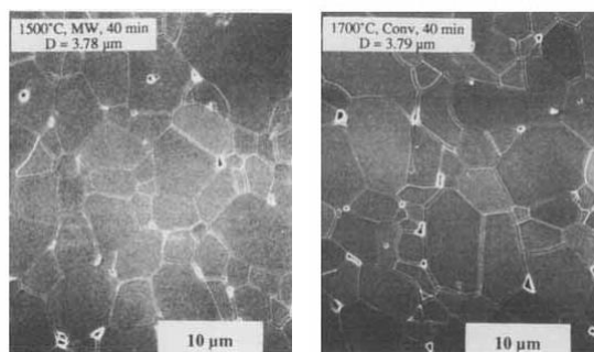
Figure A.42 – Comparaison des microstructures MEB des échantillons d'alumine de Janney et al. [69] après un recuit de 40 min à 1500°C en micro-ondes et 1700°C en conventionnel
