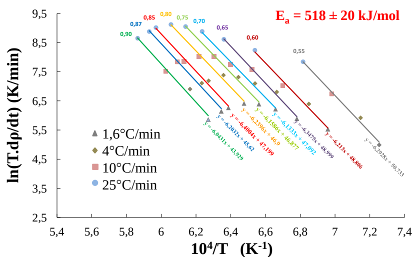
Figure B.24 – Diagramme d'Arrhénius des vitesses de densification à différentes densités à partir des courbes de retrait à quatre vitesses de chauffe pour l'alumine \alpha_{19}
