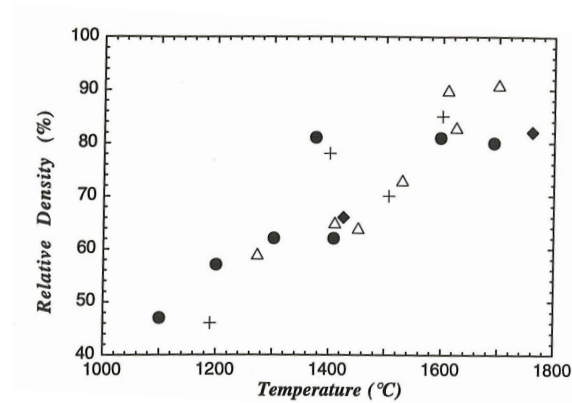
Figure A.50 – Densité en fonction de la température pour une alumine dopée avec : + 1 wt% d'Y 2 O 3 ajouté en solution, Δ 1 wt% d'Y 2 O 3 en poudre ; • 1 wt% de CaO en poudre ; ♦ 1 wt% de MgO en poudre [83]
