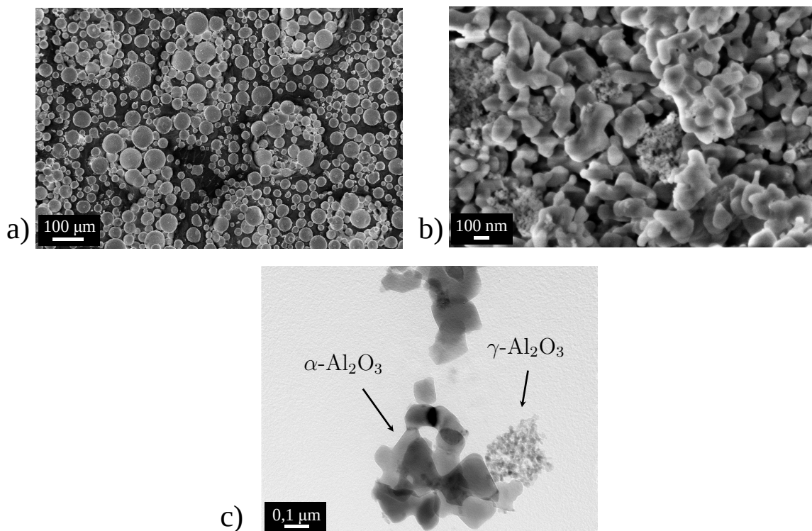
Figure B.3 – Images de la poudre \alpha_{14.3}^{500} : a) image MEB des agglomérats, b) image MEB des grains, c) image MET en champ clair des grains d' \alpha\text{-Al}_2\text{O}_3 et de \gamma\text{-Al}_2\text{O}_3
