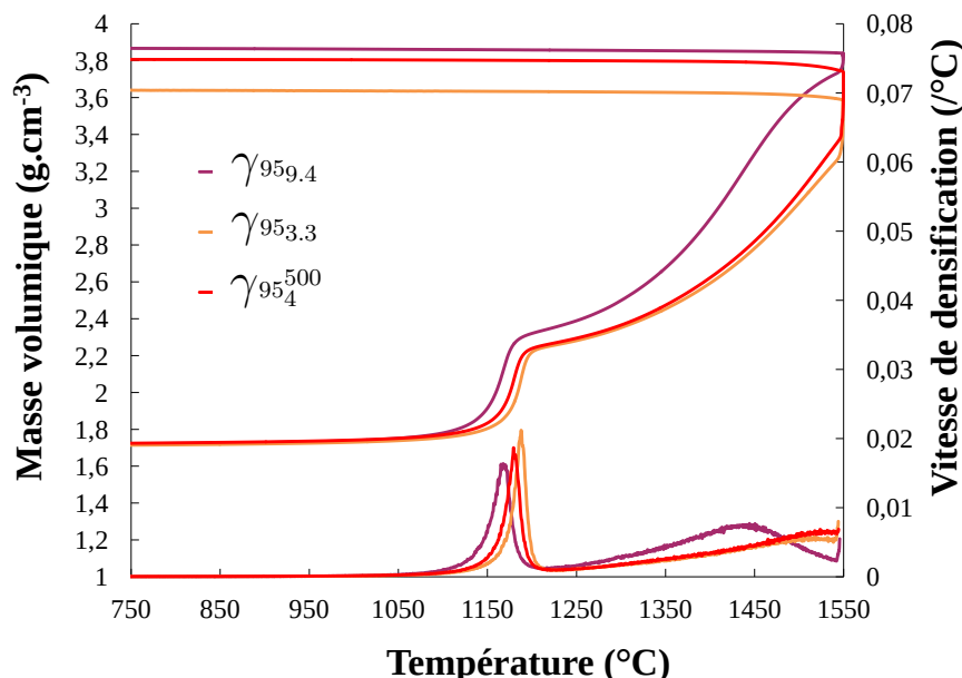
Figure B.45 – Evolution de la masse volumique et de la vitesse de densification en fonction de la température des poudres \gamma_{953,3} , \gamma_{959,4} et \gamma_{954}^{500} frittée à 25^{\circ}\text{C}/\text{min} avec un palier de 5 min à 1550^{\circ}\text{C}
