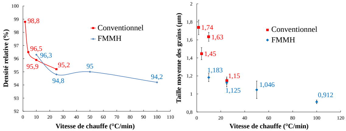
Figure D.37 – Variation de la densité relative finale et de la taille des grains en fonction de la vitesse de chauffe des échantillons de \gamma_{954}^{500} frittés en conventionnel et FMMH avec un palier de 5 min à 1550°C
