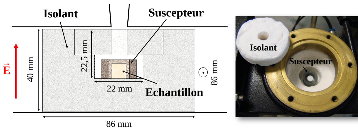
Figure C.23 – Représentation schématique (coupe médiane) et photographie de la cellule de frittage hybride disposée dans la cavité micro-ondes
