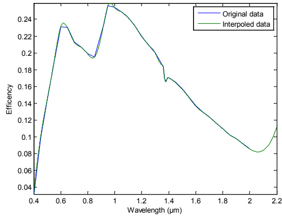
Figure 1-31 Transmission spectrale de l'ensemble des optiques de VIHI
