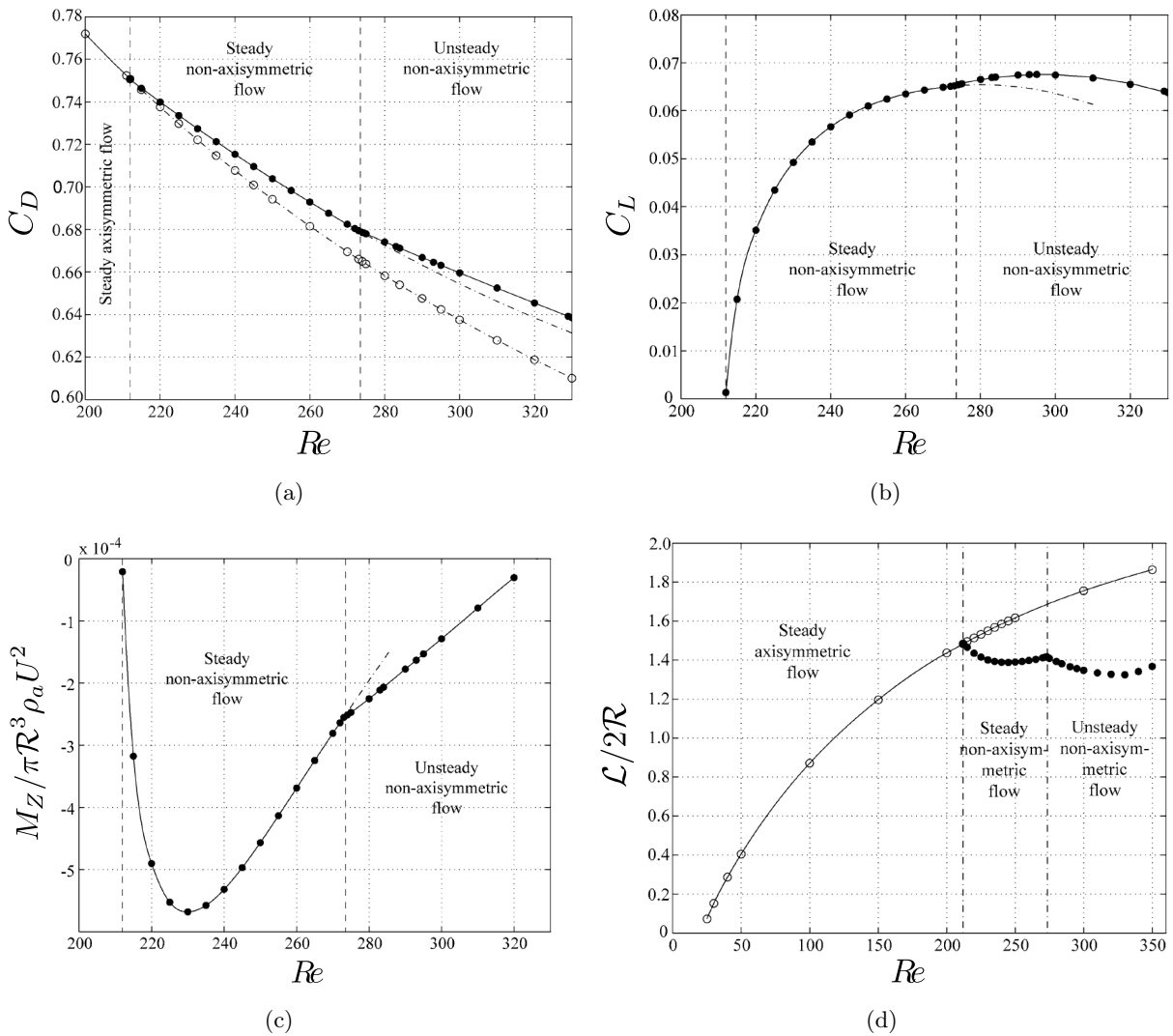
FIGURE 4.26 – Prédictions numériques, en fonction du nombre de Reynolds, (a) du coefficient de traînée, (b) du coefficient de portance, (c) du moment hydrodynamique adimensionné (avec la convention de signe de la figure 4.25) et (d) de la longueur de recirculation adimensionnée d’une sphère solide ; les cercles vides correspondent au flux axisymétrique forcé, alors que les cercles pleins représentent le flux total ; les pointillés traduisent une extrapolation des résultats subcritiques. Les résultats en régime instationnaire correspondent à des grandeurs moyennées temporellement. (Images issues de [16].)
