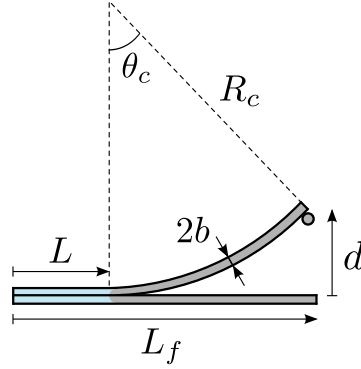
FIGURE 2.28 – Schéma de la géométrie étudiée : deux fibres de rayon b et de longueur L_f sont en contact sur une longueur L grâce à la force d'adhésion capillaire due au liquide étalé. La présence d'une troisième fibre dans un plan transverse, et à une distance d de leur axe initial, impose à la fibre supérieure une déflexion définie par l'angle \theta_c et le rayon de courbure R_c .
