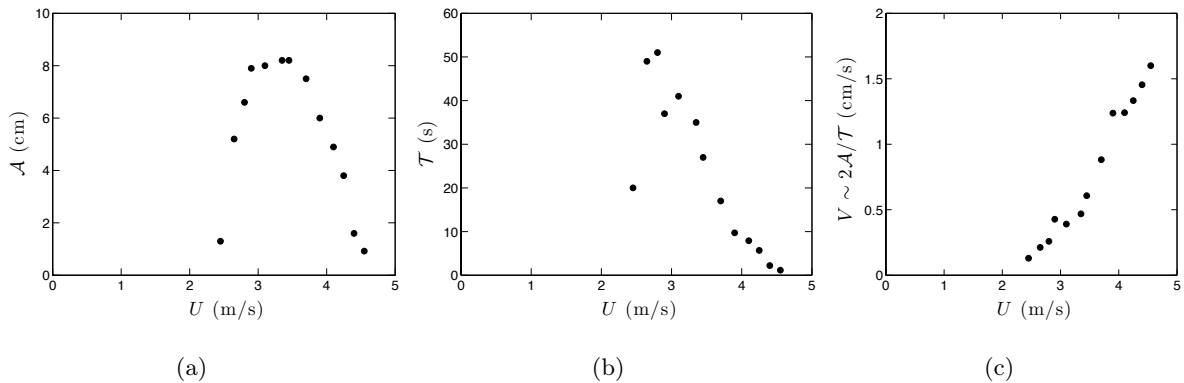
FIGURE 4.58 – Tracés de (a) l'amplitude, (b) la période et (c) la vitesse de la goutte en fonction de la vitesse du vent ; ces mesures sont issues des signaux quasi triangulaires de la figure 4.57. La dernière figure indique que la relation V(U) est sensiblement identique à celle tracée sur la figure 4.12(b), obtenue avec une soufflerie plus "propre", où de telles oscillations ne sont pas observées.
