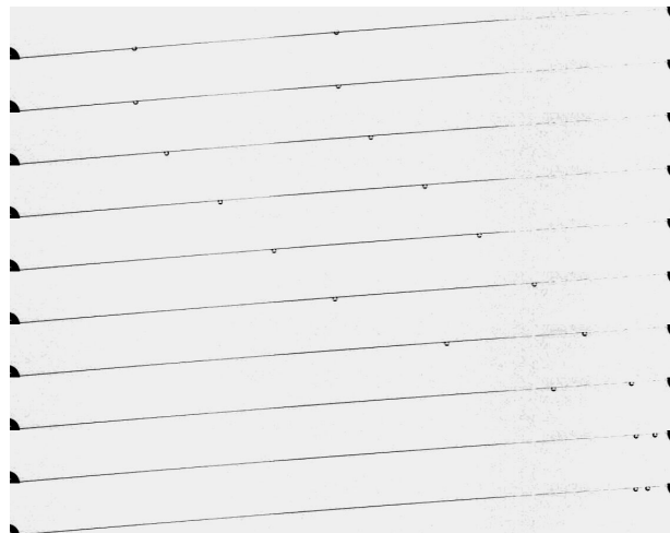
FIGURE 4.51 – Succession de photographies ( \Delta t = 2 s) montrant le déplacement de deux gouttes funambules ( \eta = 5 mPa.s, \Omega = 1 \mu L, b = 75 \mu m) placées sur un fil incliné d’un angle \delta = 4^\circ par rapport à la perpendiculaire au flux d’air, de vitesse U = 5 m/s. Une fois cette vitesse établie, les gouttes ont un mouvement déterministe, elles remontent toujours le vent et ne rebrousse jamais chemin ; elles ne rebondissent plus sur des obstacles mais s’arrêtent à proximité (en oscillant légèrement sur place).
