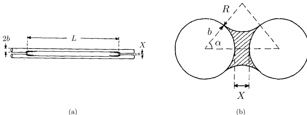
FIGURE 1.4 – Schémas de la forme de "colonne" adoptée par un volume de liquide mouillant étalé entre deux fibres proches, et notations associées : (a) vue latérale ; les fibres sont de rayon b , espacées de X , et le liquide est étalé sur une longueur L ; (b) vue en coupe loin des bords ; la section liquide hachurée est d'aire A , définie par le rayon de courbure R et l'angle \alpha entre la droite joignant le centre des fibres et celle joignant le centre d'une fibre et l'intersection de la ligne triple avec le plan de la figure. (Figures issues de [112] et [113].)
