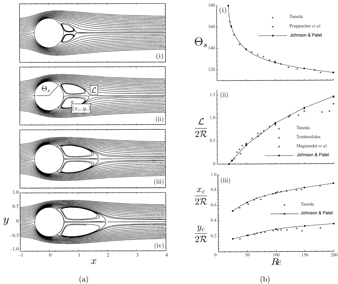
FIGURE 4.22 – (a) Tracé numérique des lignes de courant axisymétriques autour d’une sphère, pour un nombre de Reynolds valant : (i) 50, (ii) 100, (iii) 150 et (iv) 200. (b) Tracé numérique de la géométrie du flux (avec les notations de (a)(ii)) en fonction du nombre de Reynolds, et comparaison avec les données expérimentales issues de [146], et numériques issues de [115], [153] et [79] : (i) angle de séparation (entre le point de stagnation et le point de séparation du flux avec la surface de la sphère), (ii) longueur de recirculation et (iii) position du vortex. Les longueurs sont adimensionnées par le diamètre de la sphère. (Images issues de [55].)
