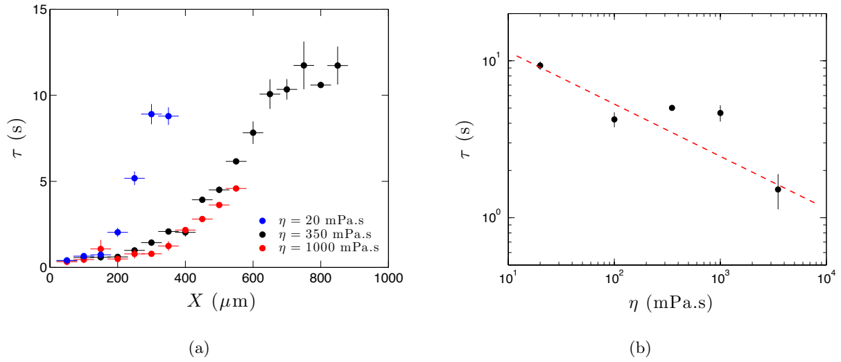
FIGURE 1.36 – (a) Temps d’amortissement \tau des oscillations en fonction de l’espaceur X , pour un volume \Omega = 1.6 \mu\text{L} d’huiles silicones de 3 viscosités différentes. (b) Tracé en coordonnées logarithmiques de \tau en fonction de la viscosité \eta , pour \Omega = 1.6 \mu\text{L} et un espaceur fixé X \approx 500 \mu\text{m} . La droite en pointillés rouges est de pente -1/3 .
