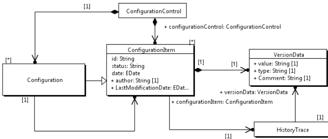
Figure 83 : diagramme de gestion en configuration
