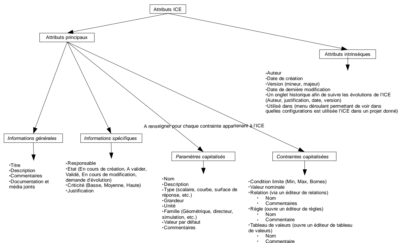
Figure 37 : attributs des ICEs
