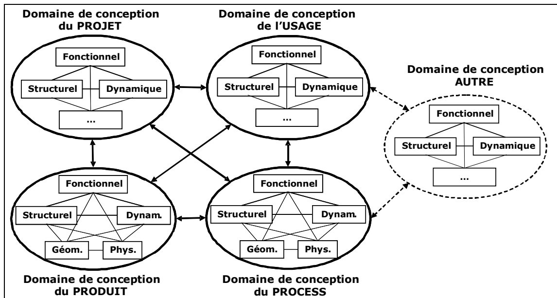
Figure 19 : modèle de données systémique "multi-domaines et multi-vues" comprenant plusieurs aspects appliqués à plusieurs domaines de conception [Gomes, 2002]
