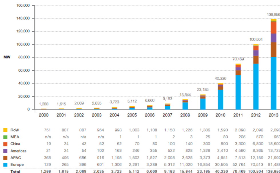
Figure 1. 1 : Évolution de la puissance mondiale cumulée de modules photovoltaïques installés [10]
