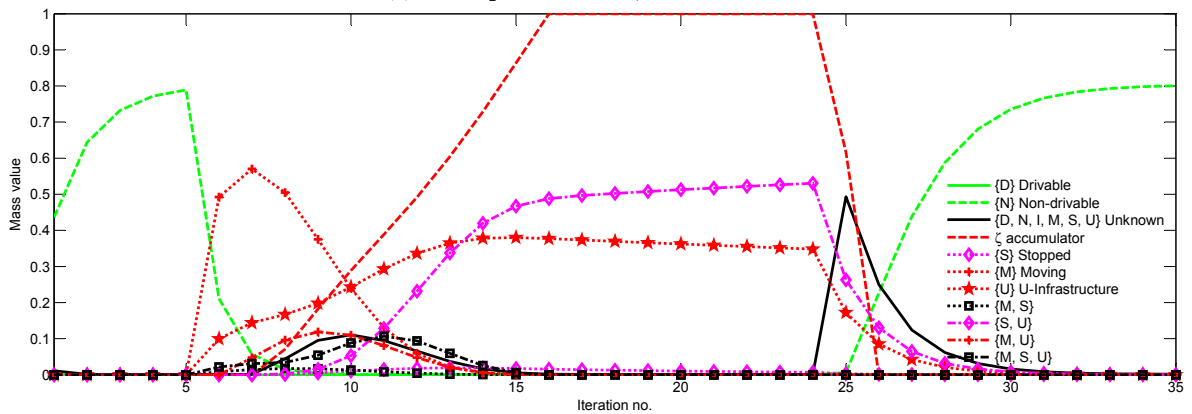
(d) PerceptionGrid. \gamma = 6, \delta = 0.15
