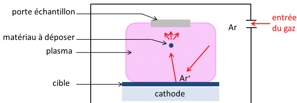
Figure 3.1 : Schéma du fonctionnement du pulvérisateur cathodique.
