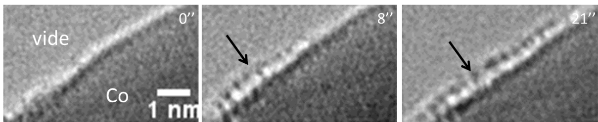
Figure 4.8 : Croissance de la structure de silice sur le bord d'une nanoparticule de Co. Les premières cellules commencent à se voir 8 s après l'irradiation et continuent à croître sur toute la région irradiée.
