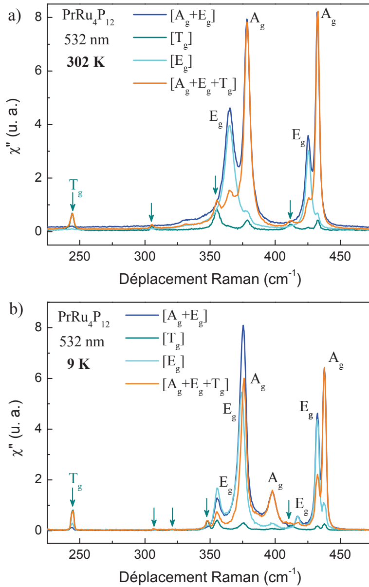
FIGURE 3.11 – Spectres Raman des phonons au-dessus de 200 \text{ cm}^{-1} dans \text{PrRu}_4\text{P}_{12} dans différentes symétries à 302 K a) et 9 K b). Les flèches vertes indiquent la position des phonons T_g . Tous ces spectres ont été réalisés avec l'échantillon #1.
