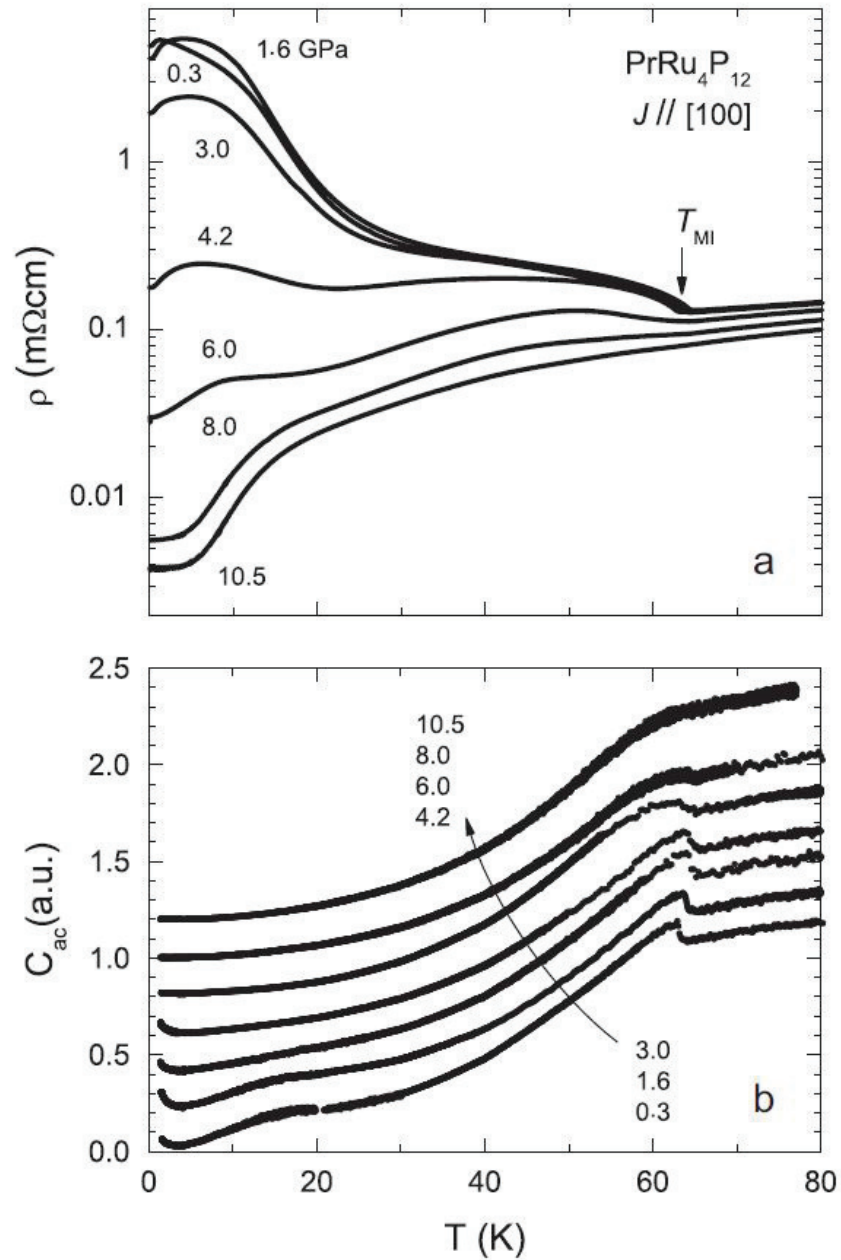
FIGURE 3.8 – Dépendance en température de la résistivité (a) et de la chaleur spécifique (b) à différentes pressions dans \text{PrRu}_4\text{P}_{12} . Ces mesures sont extraites de la Réf. [Miyake, 2008].
