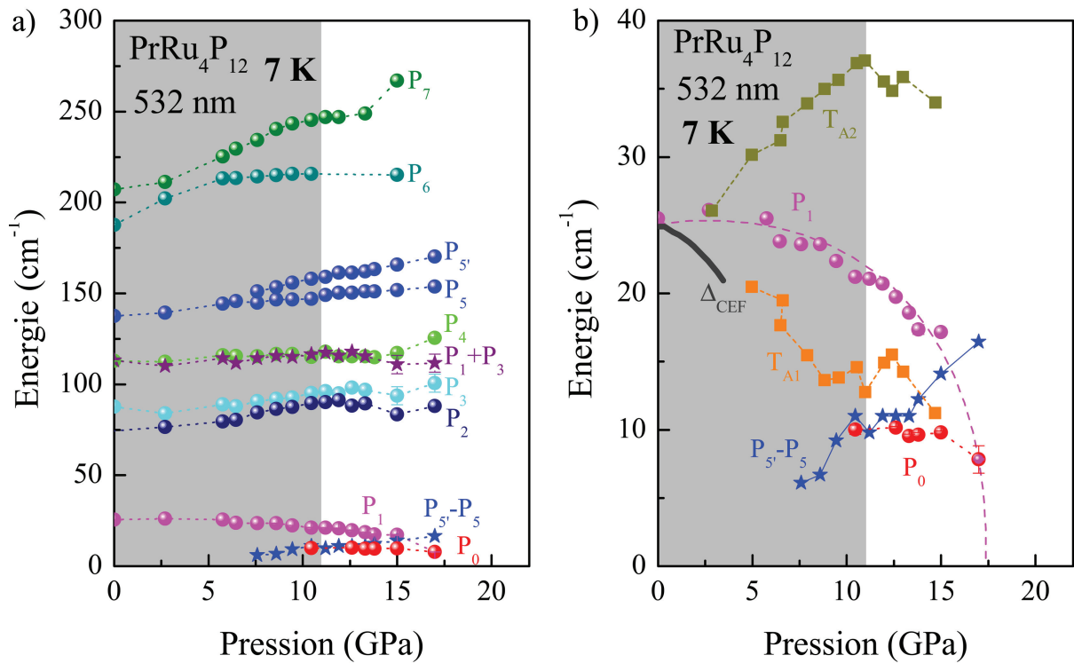
FIGURE 3.21 – a) Dépendance en pression de l'énergie des excitations de champ cristallin de \text{PrRu}_4\text{P}_{12} . b) Agrandissement à basse énergie de la dépendance en pression de l'énergie des excitations de champ cristallin P_0 et P_1 . La courbe marron correspond à la dépendance en pression de l'énergie de la transition \Gamma_4^{(2)} \rightarrow \Gamma_1 ( \Delta_{\text{CEF}} \equiv P_1 ) extraite des mesures de chaleur spécifique [Miyake, 2008]. T_{A1} et T_{A2} correspondent aux anomalies relevées en résistivité sous pression [Miyake, 2008].
