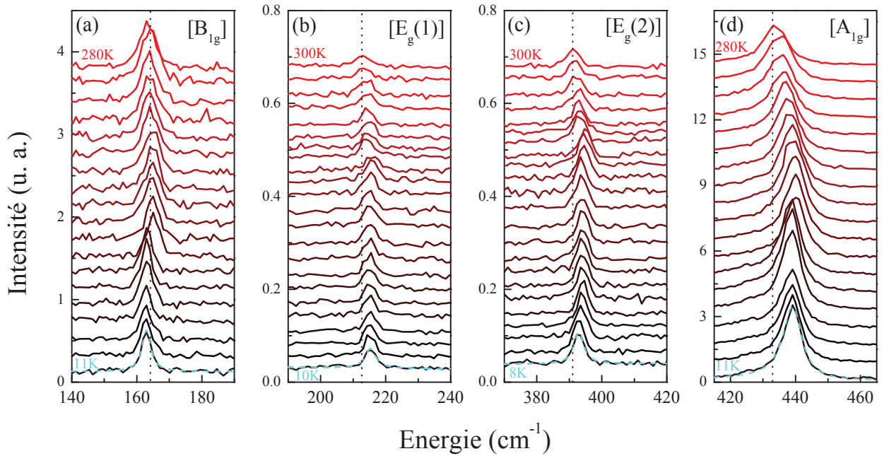
FIGURE 4.33 – Dépendance en température des spectres Raman des modes de phonons B 1g (a), E g (1) (b), E g (2) (c) et A 1g (d). Les lignes discontinues bleues aux basses températures sont des fits Lorentziens.
