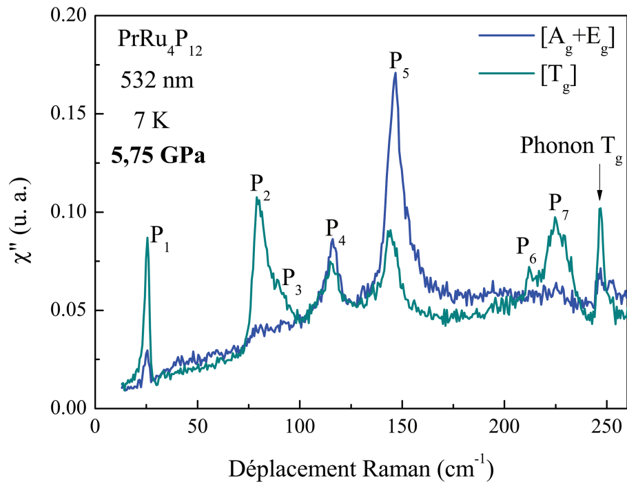
FIGURE 3.18 – Spectres Raman des excitations de champ cristallin de \text{PrRu}_4\text{P}_{12} , à 7 K et 5,75 GPa, dans les symétries [A_g + E_g] a) et [T_g] .
