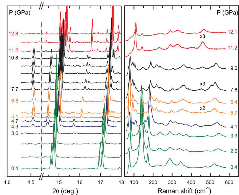
FIGURE 5.6 – Spectres de diffraction X (à gauche) et spectres Raman (à droite) de BiFeO 3 sous pression d'après [Guennou, 2011]. Trois phases orthorhombiques complexes (O 1 , O 2 et O 3 ) sont observées sous pression entre les phases R3c (en vert) et Pnma (en rouge).
