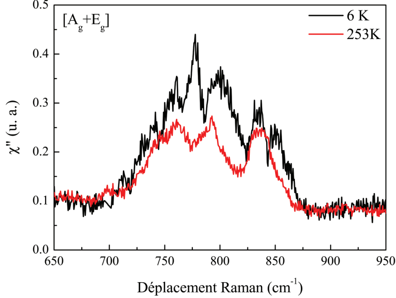
FIGURE 3.13 – Spectres Raman de \text{PrRu}_4\text{P}_{12} à haute énergie dans la symétrie [A_g+E_g] à 6 K et 253 K. Les excitations observées correspondent à des processus phononiques doubles (Cf. texte). Ces mesures ont été faites avec l'échantillon #2.
