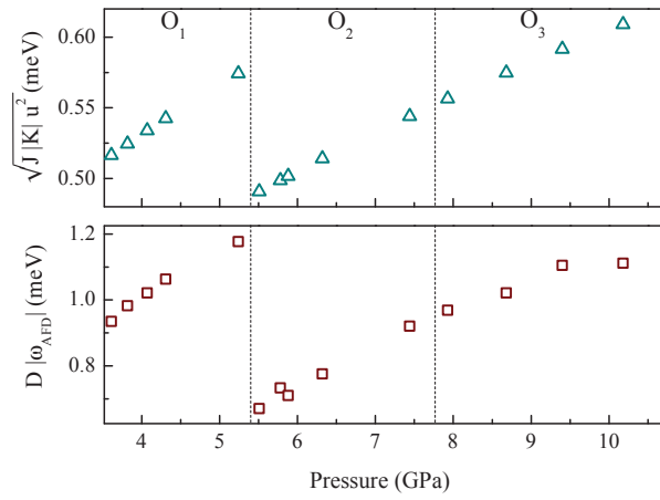
FIGURE 5.12 – Dépendance en pression des paramètres \sqrt{|J|K|u^2} et |D| à travers les phases O 1 , O 2 et O 3 .
