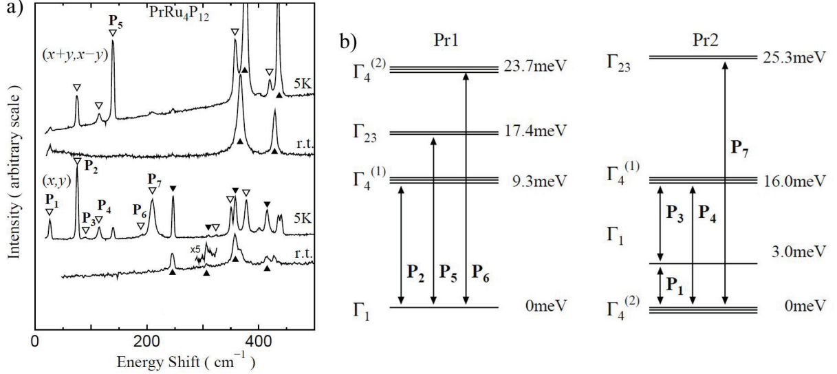
FIGURE 3.7 – a) Spectres Raman de \text{PrRu}_4\text{P}_{12} mesurés par Ogita et al. [Ogita, 2009] à température ambiante (r.t.) et dans la phase isolante (5 K). Les triangles pleins indiquent les phonons dans la phase métallique et les triangles vides les nouveaux phonons dans la phase isolante. Les pics nommés de \text{P}_1 à \text{P}_6 sont des excitations de champ cristallin. b) Schémas de champ cristallin de \text{PrRu}_4\text{P}_{12} proposés par Ogita et al. [Ogita, 2009].
