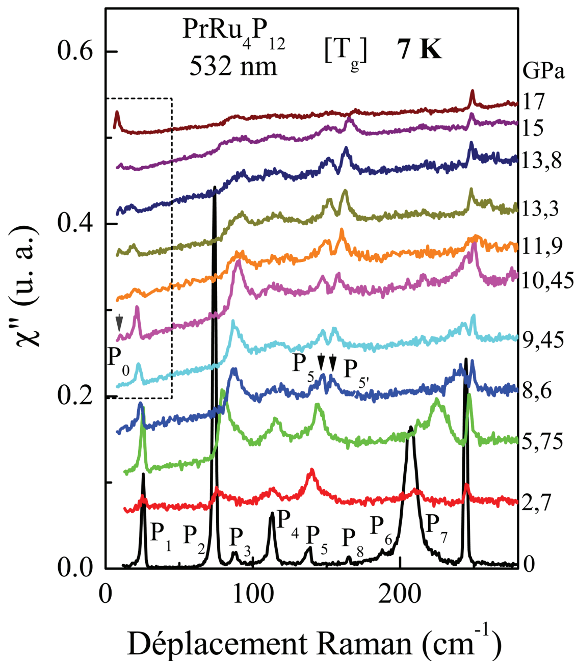
FIGURE 3.19 – a) Spectres Raman des excitations de champ cristallin dans \text{PrRu}_4\text{P}_{12} à 7 K, de 0 à 17 GPa. Tous ces spectres ont été réalisés avec l'échantillon #1. Les excitations P_0 et P_1 de 9.45 à 17 GPa à l'intérieur du cadre pointillé ont été agrandies pour plus de clarté en FIG. 3.20 a).
