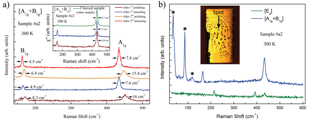
FIGURE 4.11 – a) Spectres Raman dans la configuration a(ab)\bar{a} ( A_{1g} + B_{1g} ) pour l'échantillon #a2 après le premier polissage (en marron), le premier recuit (en bleu), le second polissage (en orange) et le second recuit (en rouge). L'insert montre les spectres Raman dans la configuration c(aa)\bar{c} ( A_{1g} + B_{1g} ) pour l'échantillon #c2 après le premier polissage (en marron), le premier recuit (en bleu) et pour un échantillon clivé (en vert) b) Spectres Raman de l'échantillon 1 obtenu avec le spot laser focalisé sur les taches sombres, dans les configurations a(aa)\bar{a} ( A_{1g} + B_{1g} ) et a(ac)\bar{a} ( E_g ), après le premier recuit. Le symbole * indique les raies parasites du laser.
