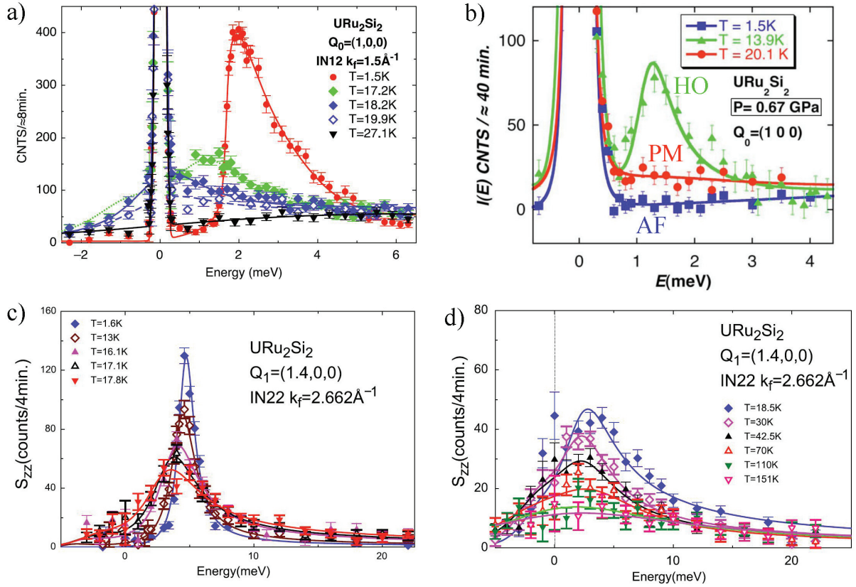
FIGURE 4.7 – a) Spectres en énergie à Q_0 pour différentes températures à travers la transition d'ordre caché [Bourdarot, 2010]. b) Spectres en énergie à Q_0 dans les phases antiferromagnétique (AF), d'ordre caché (HO) et paramagnétique (PM) [Villaume, 2008]. c) et d) Spectres en énergie à Q_1 pour différentes températures à travers la transition d'ordre caché [Bourdarot, 2014].
