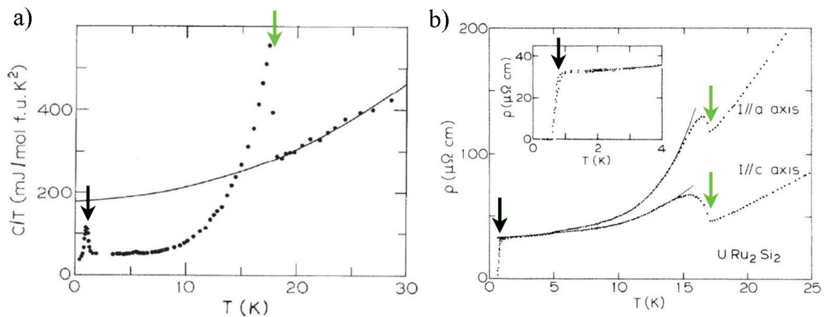
FIGURE 4.4 – a) Chaleur spécifique divisée par la température en fonction de la température [Palstra, 1985] b) Résistivité selon l'axe a et l'axe c en fonction de la température [Palstra, 1985]. L'insert est un agrandissement autour de la température de transition supraconductrice. Les flèches vertes et noires indiquent respectivement les transitions d'ordre caché et supraconductrice.
