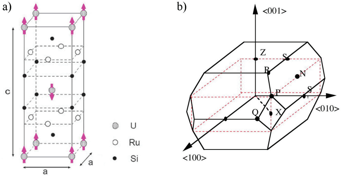
FIGURE 4.5 – a) Structure cristallographique de URu 2 Si 2 avec les moments des atomes d'uranium orientés selon l'axe c dans la phase antiferromagnétique. Dans ce cas, la structure est tétragonale simple mais si on néglige les moments magnétiques des uraniums, ces derniers deviennent tous équivalents, la structure est alors tréragonale centrée, ce qui est le cas dans la phase paramagnétique. b) En noir : zone de brillouin tréragonale centrée dans la phase paramagnétique. En rouge : zone de brillouin tréragonale simple dans la phase antiferromagnétique.
