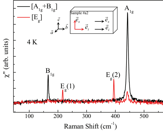
FIGURE 4.32 – Spectres Raman des phonons de URu 2 Si 2 mesurés à 4 K dans l'échantillon 1 (Cf. section 4.2.1). Le schéma représente l'échantillon 1 avec les orientations des polarisations incidentes \vec{e}_i et diffusées \vec{e}_s (Cf. section 4.2.2).
