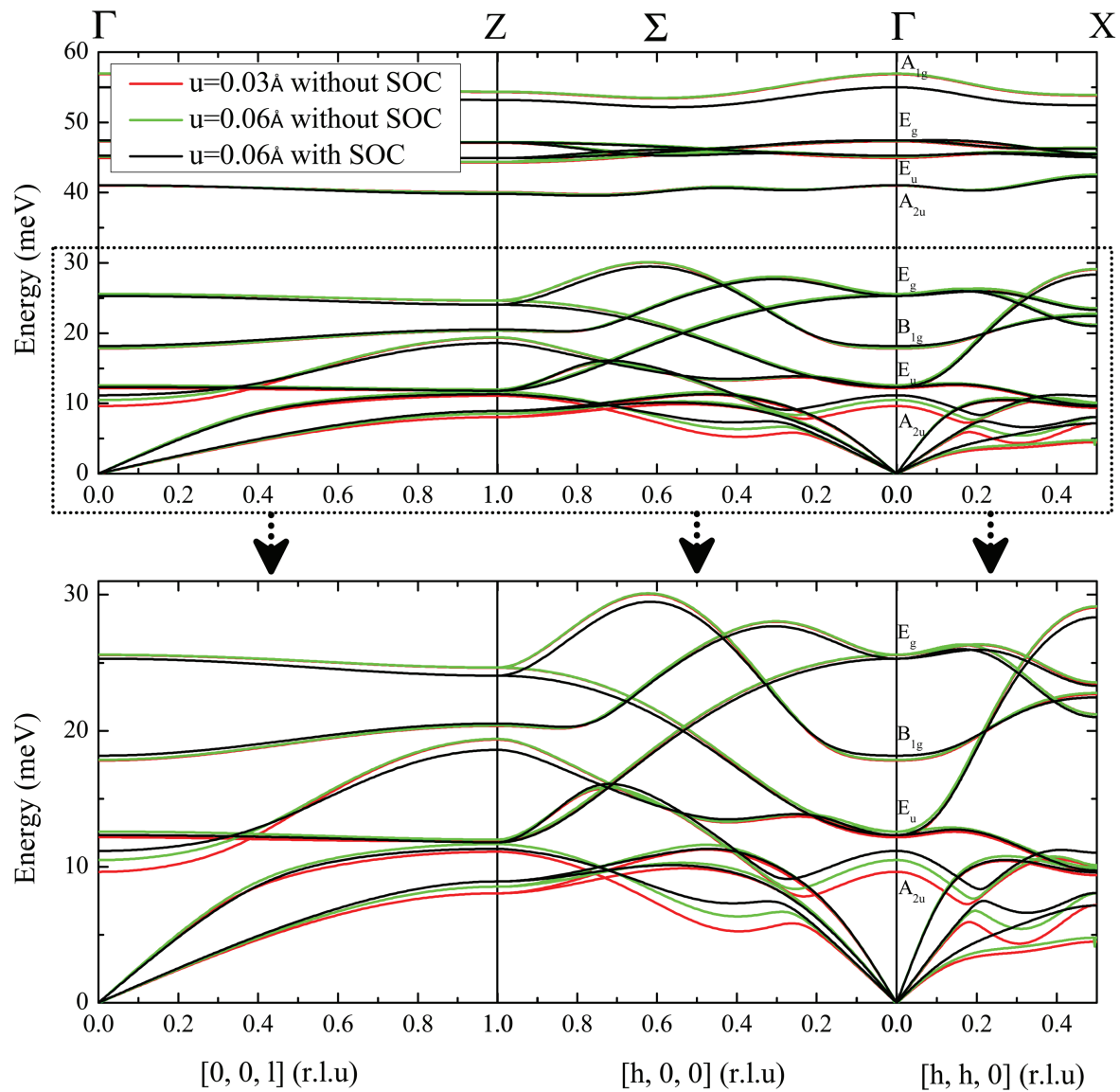
FIGURE 4.50 – Calcul Ab initio de la dispersion des phonons dans les directions \Gamma Z , \Gamma\Sigma Z et \Gamma X à 0 K. Le paramètre u fixe le déplacement des atomes. L'augmentation du paramètre u de 0.03 \text{ \AA} (ligne rouge) à 0.06 \text{ \AA} (ligne verte) est utilisée pour sonder les effets d'anharmonicité. La courbe noire montre le calcul avec le couplage spin-orbite (SOC).
