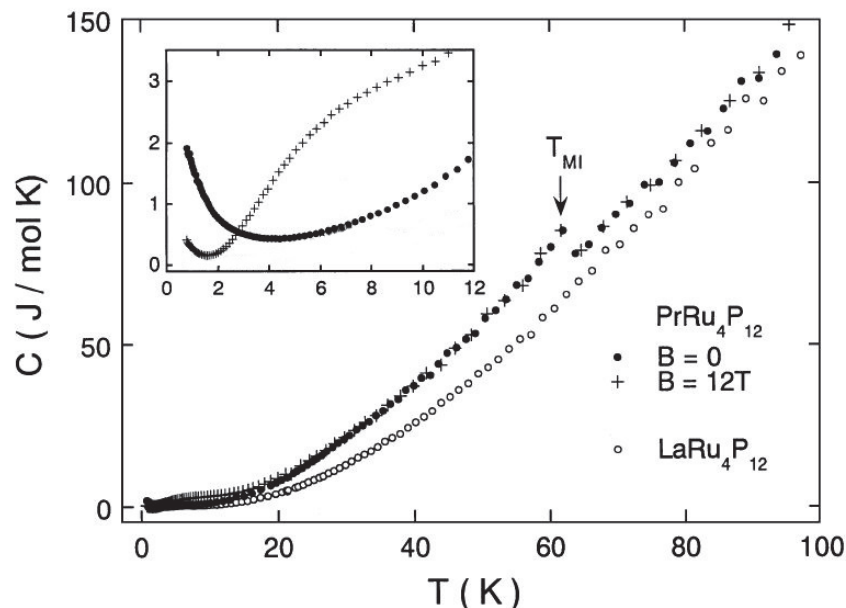
FIGURE 3.3 – a) Dépendance en température de la chaleur spécifique de \text{PrRu}_4\text{P}_{12} à 0 T et 12 T et de \text{LaRu}_4\text{P}_{12} à 0 T. L'insert montre la chaleur spécifique à basse température de \text{PrRu}_4\text{P}_{12} à 0 T et 12 T. Ces mesures sont extraites de la Ref. [Sekine, 2000].
