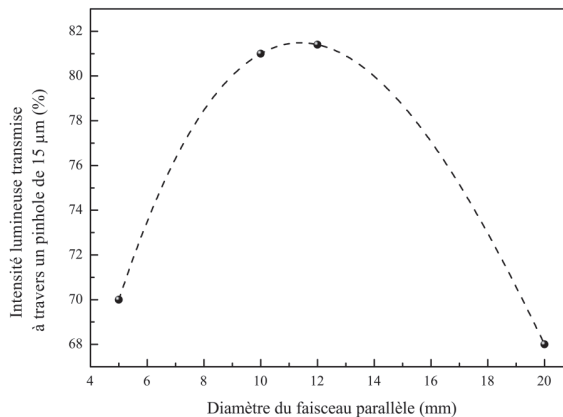
FIGURE 2.5 – Intensité lumineuse relative à la sortie d'un pinhole test de 15 \mu m pour différents diamètres d de faisceau parallèle.
