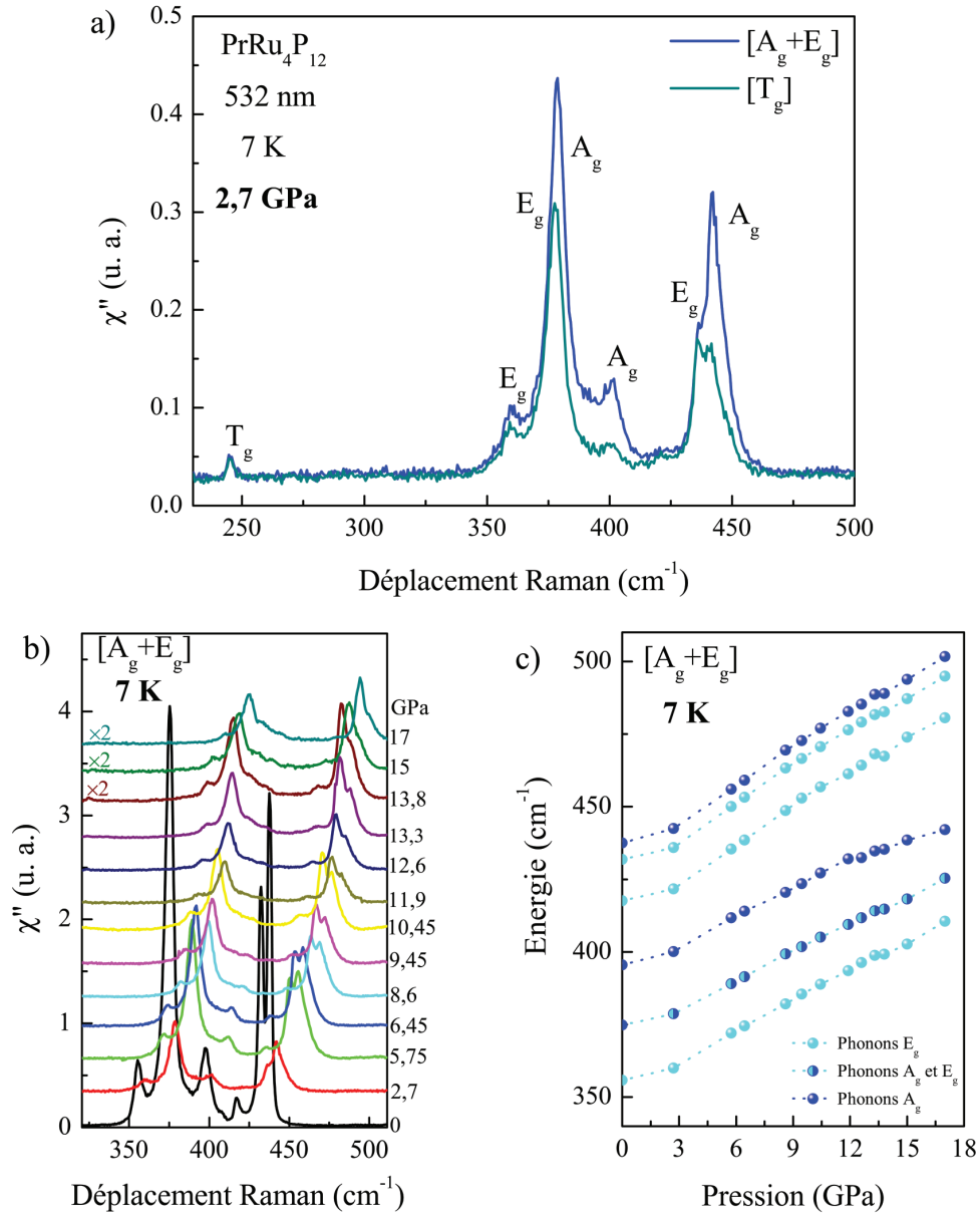
FIGURE 3.16 – a) Spectres Raman des phonons de \text{PrRu}_4\text{P}_{12} dans différentes symétries à 7 K et 2,7 GPa. b) Spectres Raman des phonons de \text{PrRu}_4\text{P}_{12} à 7 K de 0 à 17 GPa. Tous ces spectres ont été réalisés avec l'échantillon #1. c) Evolution en pression de l'énergie des phonons dans \text{PrRu}_4\text{P}_{12} .
