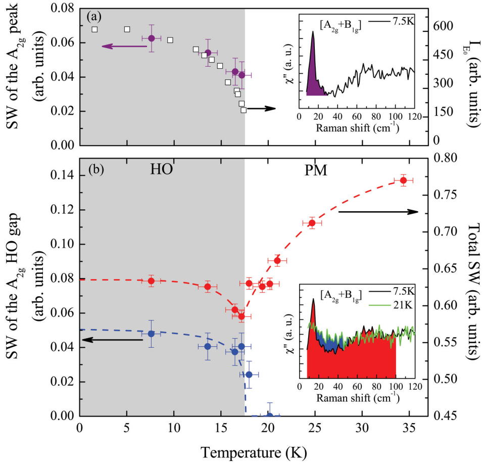
FIGURE 4.25 – (a) Poids spectral du pic Raman A_{2g} et intégrale de la partie imaginaire la susceptibilité dynamique de spin neutronique à \mathbf{Q}_0 , I_{E_0} [Bourdarot, 2010] en fonction de la température. Insert : Illustration de l’intégration du poids spectral du pic Raman A_{2g} . (b) Poids spectral du gap d’ordre caché juste au dessus du pic d’ordre caché et poids spectral total dans la symétrie A_{2g} . Insert : Illustration de l’intégration des différents poids spectraux dans la symétrie A_{2g} .
