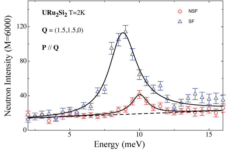
FIGURE 4.48 – Spectres de diffusion inélastique de neutrons polarisés pour \mathbf{Q}=(1.5, 1.5, 0) dans les canaux Non Spin Flip (NSF) et Spin Flip (SF) à T = 2 K. Les lignes continues sont des fits de nos données avec un profil d'oscillateur harmonique amorti pour le phonon et avec un profil \omega -Lorentzien pour l'excitation magnétique (pour plus de détails sur ce type de profil Cf. [Panarin, 2011]). La ligne discontinue indique le fond. L'intensité neutronique est donnée pour un flux incident normalisé (M) qui correspond à un temps de comptage d'environ 25min.
