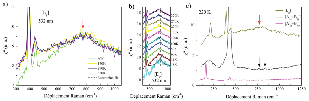
FIGURE 4.29 – a) Spectres Raman à haute énergie dans la symétrie E_g à différentes températures. La flèche rouge indique une large excitation possiblement due à une transition de champ cristallin. b) Dépendance en température de cette excitation. Les deux courbes noires à 300K et 15K sont des fits Lorentziens. Pour plus de clarté les spectres ont été décalés en ordonnée. b) Spectres Raman à haute énergie dans les symétries E_g , [A_{1g}+B_{2g}] et [A_{2g}+B_{1g}] à 200K. La flèche rouge indique la large excitation dans la symétrie E_g présentée en a) et les flèches noires les pointent les doubles phonons observés dans la symétrie A_{1g} . Toutes les températures pour a), b) et c) ont été corrigées de l'échauffement laser à \pm 1K .
