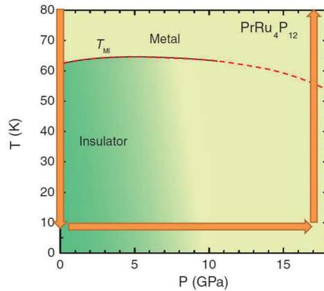
FIGURE 3.23 – Diagramme de phase pression-température de \text{PrRu}_4\text{P}_{12} . Les flèches orange représentent les zones du diagramme de phase que nous avons sondé par spectroscopie Raman. La ligne rouge discontinue indique la transition structurale Im\bar{3} - Pm\bar{3} et la ligne noire continue jusqu'à 10 GPa indique la transition métal-isolant.
