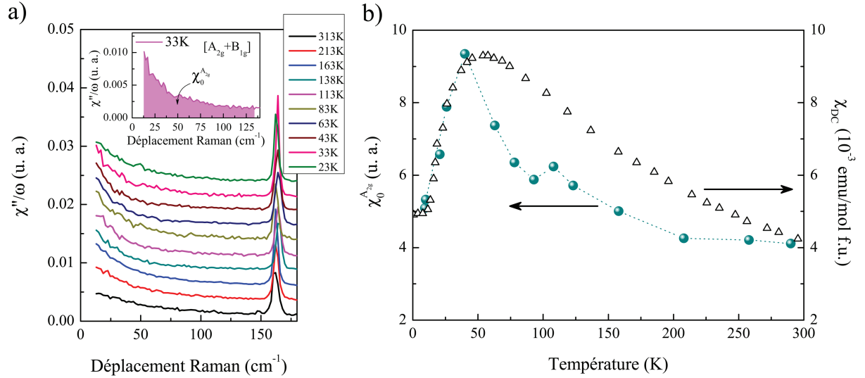
FIGURE 4.26 – a) Spectres Raman divisés par \omega à différentes températures dans la symétrie [A_{2g}+B_{1g}] . L'insert montre un exemple à 33K de l'intégrale nous permettant d'extraire la susceptibilité Raman statique A_{2g} b) Susceptibilité Raman statique A_{2g} en fonction de la température (échelle de gauche) et susceptibilité magnétique DC [Palstra, 1986b] (échelle de droite). La ligne pointillée est un guide pour les yeux.
