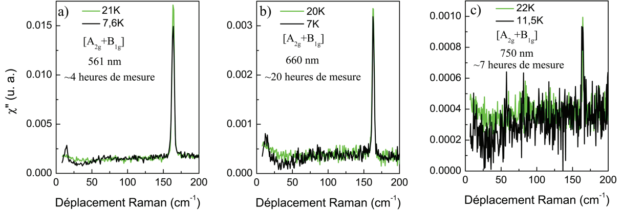
FIGURE 4.18 – Spectres Raman de \text{URu}_2\text{Si}_2 dans la phase d'ordre caché et la phase paramagnétique dans la symétrie [A_{2g}+A_{1g}] à 561 nm a), 660 nm b), 750 nm c). Les données pour chaque longueur d'onde ont été normalisées à une puissance laser de 1 mW. Le temps d'acquisition a été reporté sur chaque graphique.
