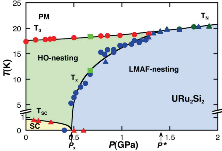
FIGURE 4.6 – Diagramme de phases de URu_2Si_2 en fonction de la température et de la pression [Villaume, 2008]. Les sigles PM, LMAF, SC et HO signifient respectivement Para-Magnetic, Large-Moment-Antiferromagnetic, SuperConductor et Hidden-Order.
