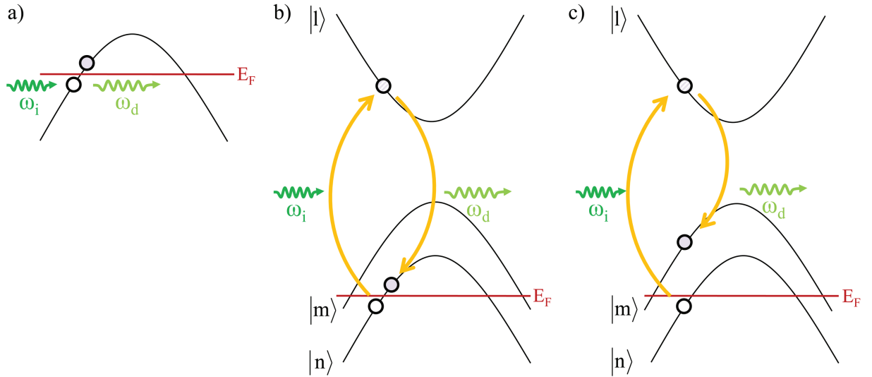
FIGURE 1.4 – a) Diffusion Raman électronique du premier ordre en perturbation (intrabande) b) Diffusion Raman électronique du second ordre en perturbation (intrabande) c) Diffusion Raman électronique du second ordre en perturbation (interbande).
