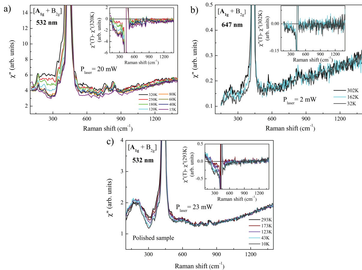
FIGURE 4.52 – Spectres Raman dans la symétrie A_{1g} + B_{2g} à différentes températures réalisés à 532 nm a) et 647 nm b) avec des échantillons d' \text{URu}_2\text{Si}_2 fraîchement clivés et à 532 nm c) avec un échantillon poli. Les inserts montrent les réponses Raman à chaque température auxquelles ont été soustraites les réponses à température ambiante. Les spectres à 15 K et 10 K à 532 nm sont normalisés, ils ont été réalisés avec une puissance laser de 2 mW. Toutes les températures reportées sont corrigées de l'échauffement laser.
