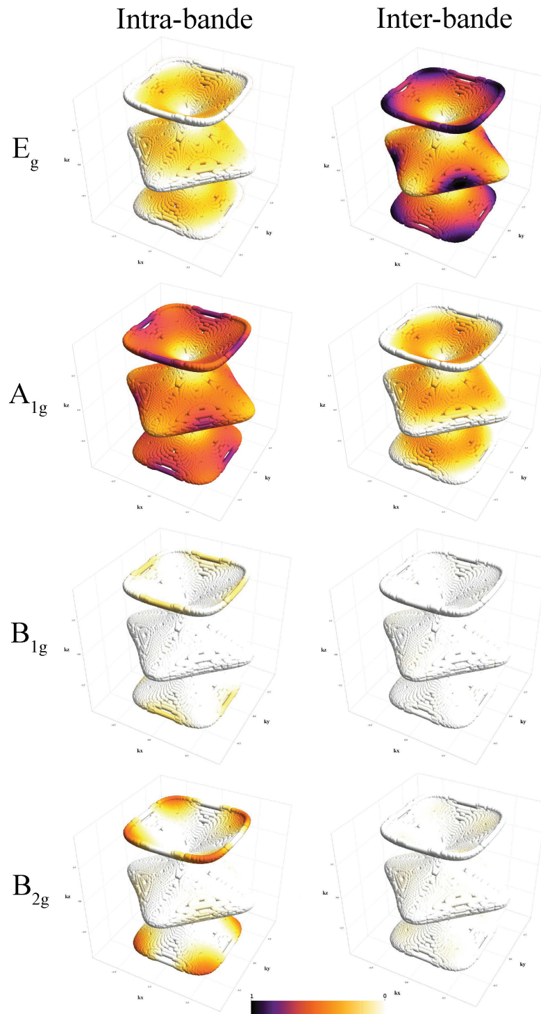
FIGURE 4.57 – Vertex Raman intra et inter-bandes calculés par X. Montiel dans l’approximation de la masse effective pour les symétries E_g , A_{1g} , B_{1g} et B_{2g} . Les vertex sont normalisés par le E_g inter-bande qui présente l’intensité absolue la plus grande. Les zones où l’intensité du vertex Raman est maximum sont représentées en noir. Les zones en blanc indiquent que le vertex est nul.
