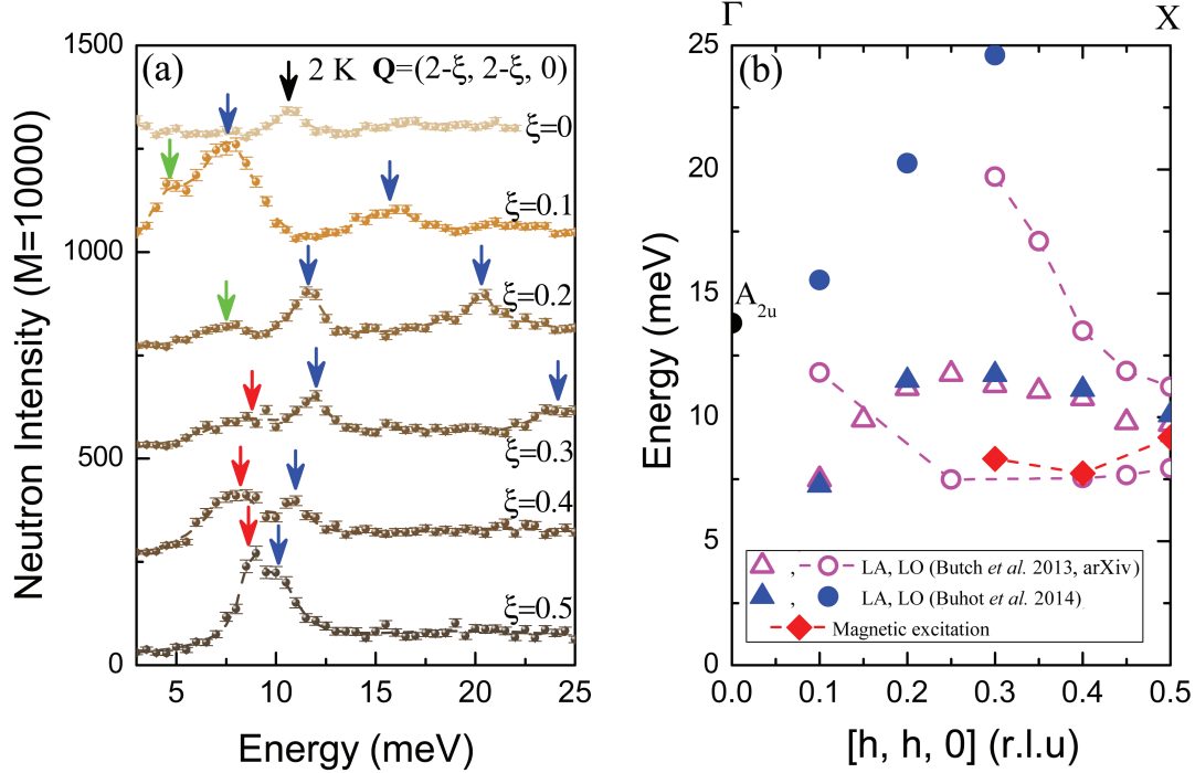
FIGURE 4.47 – (a) Spectres de diffusion inélastique de neutrons mesurés à 2 K sur IN22 dans la direction [h,h,0] pour \mathbf{Q}=(2-\xi, 2-\xi, 0) . Les flèches bleues, rouges, vertes et noires indiquent respectivement des modes de phonon longitudinaux, une excitation magnétique, une fuite d'un mode de phonon transverse et le mode de phonon A_{2u} au point \Gamma . L'intensité neutronique est donnée pour un flux incident normalisé ( M ) qui correspond à un temps de comptage d'environ 80s. (b) Courbe de dispersion des modes longitudinaux obtenus dans la direction [h,h,0] . Nos données sont représentées en bleu (phonons) et rouge (excitation magnétique). Les données en rose correspondent aux modes de phonons longitudinaux rapportés par Butch et al. [Butch, 2012].
