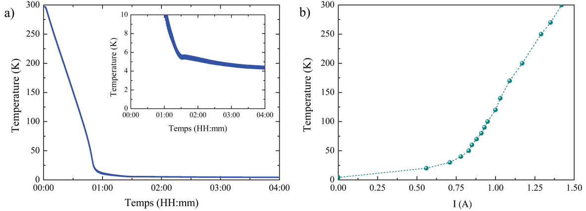
FIGURE 2.20 – a) Évolution au cours du temps de la température de l'étage échantillon de notre cryostat Absolute System. L'insert présente cette évolution en dessous de 10 K. L'origine du temps correspond à la mise en fonctionnement du compresseur. b) Température de l'étage échantillon de notre cryostat Absolute System en fonction du courant appliqué à travers les trois résistances de chauffage de 12 \Omega chacune.
