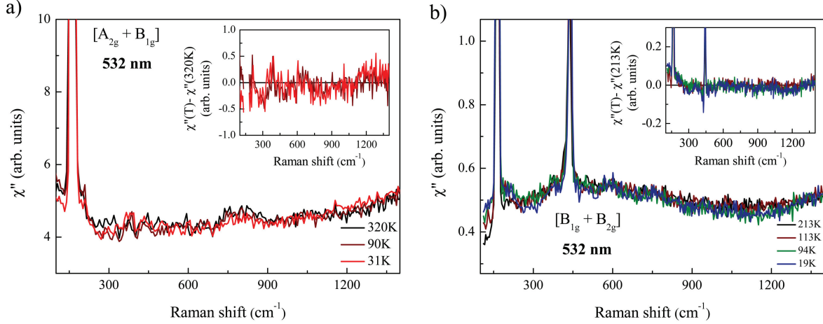
FIGURE 4.53 – Spectres Raman dans les symétries A_{2g} + B_{1g} a) et B_{1g} + B_{2g} b) à différentes températures réalisés à 532 nm avec des échantillons d'URu 2 Si 2 fraîchement clivés. Les insets montrent les réponses Raman à chaque température auxquelles ont été soustraites les réponses à haute température.
