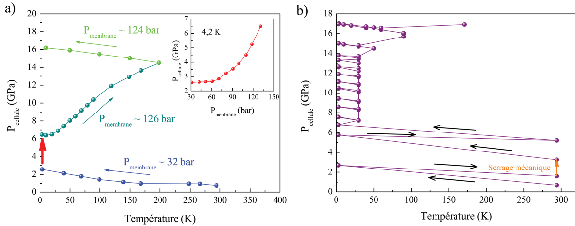
FIGURE 2.10 – a) Évolution de la pression dans la cellule lors d’une mesure test d’un échantillon de silicium à basse température. La cellule a été chargée initialement avec de l’argon gaz. Les flèches indiquent le sens de variation de la température. Les montés et descentes en température ont été faites en maintenant une pression constante dans la membrane. La flèche rouge indique la montée en pression à 4,2 K que nous avons réalisée en faisant croître la pression dans la membrane (insert) b) Évolution de la pression dans la cellule lors de la mesure du composé \text{PrRu}_4\text{P}_{12} à basse température. La cellule avait été chargée initialement avec de l’hélium gaz. Les flèches indiquent le sens de variation de la température. Toutes les augmentations de pression à température constante (à 30 K) ont été faites en faisant croître la pression dans la membrane. La flèche orange indique une augmentation de la pression dans la cellule réalisée par serrage mécanique à température ambiante.
