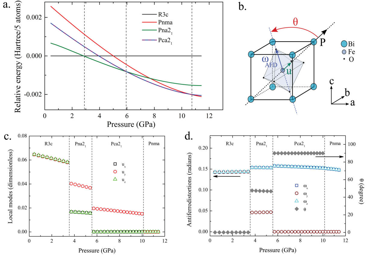
FIGURE 5.9 – a) Energies relatives des différentes structures cristallines en fonction de la pression, calculées avec un Hamiltonien effectif par D. Wang (Cf. texte). b) Schéma représentant le mode local \mathbf{u} (directement proportionnel à \mathbf{P} ), la polarisation \mathbf{P} et le vecteur d'antiferrodistorsion \omega_{AFD} qui décrit le tilt de l'octaèdre des oxygènes de BiFeO 3 dans la représentation pseudo-cubique. Le vecteur de Dzyaloshinskii-Moryia est orienté le long de \omega_{AFD} . c) Valeur moyenne du mode local \langle \mathbf{u} \rangle calculée dans chaque phase structurale en fonction de la pression. d) Vecteur d'antiferrodistorsion \omega_{AFD} calculé dans chaque phase structurale en fonction de la pression (échelle de gauche). Angle \theta entre \langle \mathbf{u} \rangle et \omega_{AFD} en fonction de la pression (échelle de droite).
