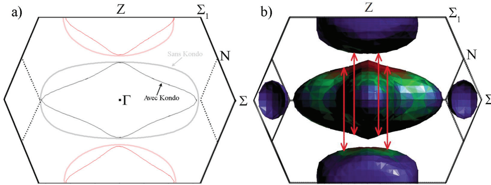
FIGURE 4.55 – a) Coupe dans le plan réciproque ( k_x, k_z ) des surfaces de Fermi \Gamma_7^{(1)} (en noir) et \Gamma_7^{(2)} (en rouge) calculé par X. Montiel grâce au modèle des liaisons fortes développé par Rau [Rau, 2012]. b) Vue de coté de la surface de Fermi de URu 2 Si 2 dans la phase PM le long de l'axe k_x [Oppeneer, 2010]. Les flèches rouges correspondent au vecteur de "nesting" Q_0 qui relie les feuillet principaux.
