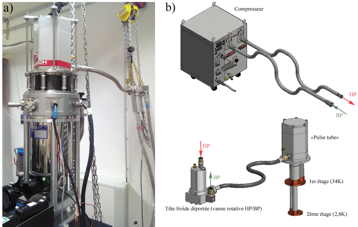
FIGURE 2.17 – a) Photographie du cryostat Absolute System en position de fonctionnement sur la table optique. b) Schéma de la machine Cryomech PT407-RM à tête froide déportée. HP et BP signifient, respectivement, haute pression et basse pression.
