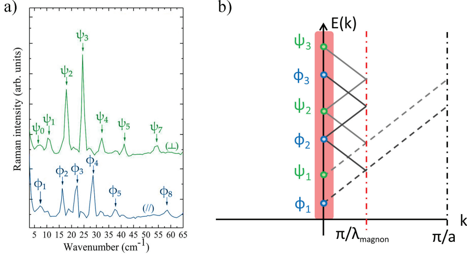
FIGURE 5.4 – a) Spectres Raman des excitations d’onde de spin dans \text{BiFeO}_3 mesurés par Cazayous et al. [Cazayous, 2008]. b) Schéma de la dispersion et du repliement des excitations antiferromagnétiques dans la 1 re zone de Brillouin.
