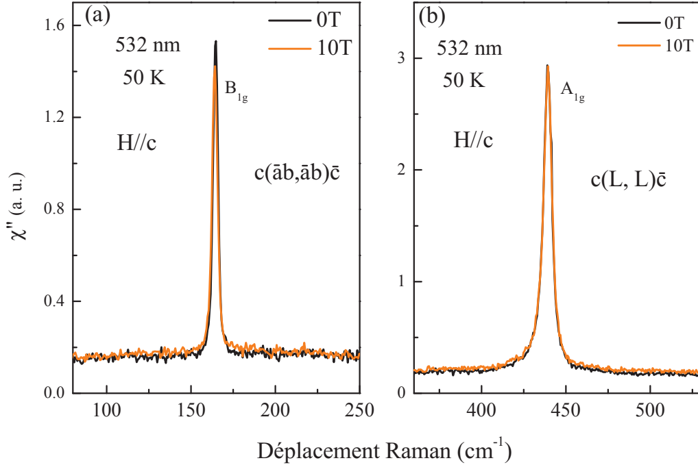
FIGURE 4.39 – Spectres Raman des phonons B_{1g} (a) et A_{1g} (b) dans URu 2 Si 2 à 0T et 10T réalisés sur un échantillon clivé refroidi à 50 K. Le champ magnétique H est orienté selon l’axe c, ainsi seuls les modes B_{1g} et A_{1g} sont accessibles.
