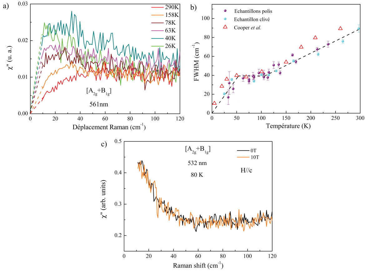
FIGURE 4.12 – a) Susceptibilité Raman dans la symétrie A_{2g}+B_{1g} de 26 K à 290 K. b) Largeur de la réponse quasi-élastique en fonction de la température. La ligne en pointillés est un guide pour les yeux. Les triangles ouverts correspondent aux mesures de Cooper et al. [Cooper, 1986]. c) Spectres Raman de l’excitation quasi-élastique A_{2g} à 0 et 10 T à la température de 80 K.
