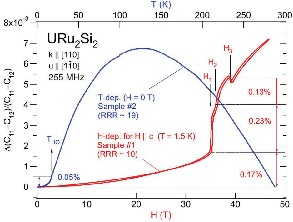
FIGURE 4.8 – Comparaison des dépendances en température (courbe bleue) et en champ magnétique (courbe rouge) de la constante C_{11} - C_{12} dans URu 2 Si 2 , extraite de la Réf. [Yanagisawa, 2013].
