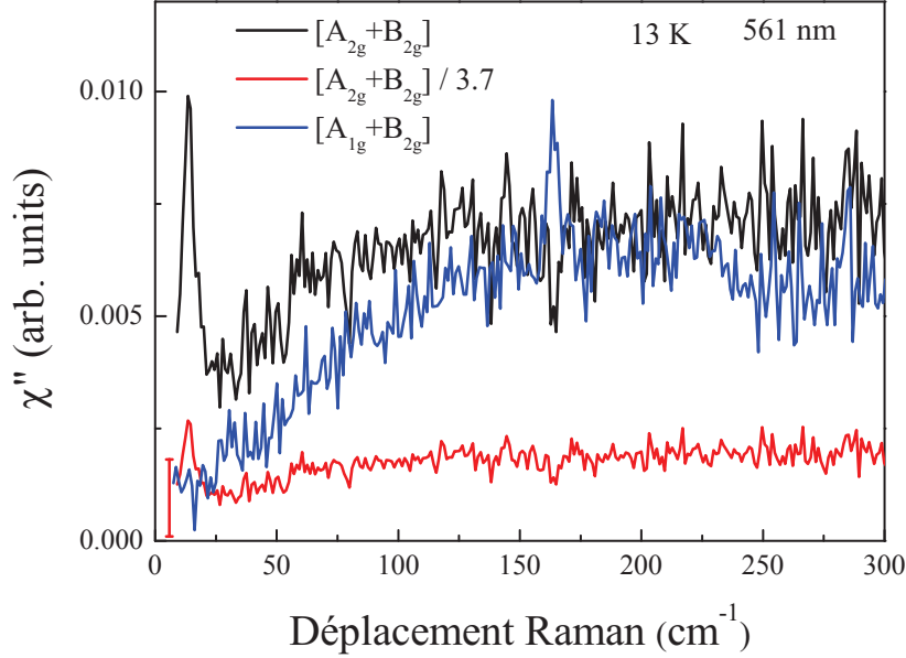
FIGURE 4.24 – Spectres Raman mesurés dans les symétries [A_{2g}+B_{2g}] et [A_{1g}+B_{2g}] . Le spectre [A_{2g}+B_{2g}] est aussi représenté avec son intensité divisée par 3.7 (Cf. texte). Ce spectre nous donne une référence sur l'intensité que devrait avoir le pic A_{1g} vu par Kung et al. [Kung, 2015].
