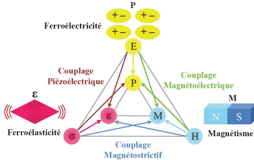
FIGURE 5.1 – Schéma présentant les principaux ordres ferroïques et leurs couplages [Spaldin, 2005]. La polarisation ( P ), l'aimantation ( M ) et la déformation ( \varepsilon ) peuvent être contrôlées respectivement par un champ électrique ( E ), un champ magnétique ( H ) et une contrainte ( \sigma ).
