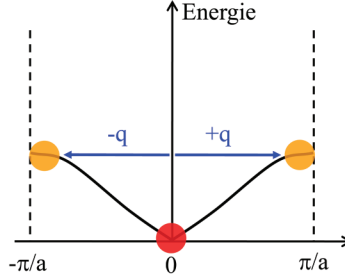
FIGURE 1.3 – Dispersion d’une excitation phononique dans la première zone de Brillouin. En rouge, la portion de la zone de Brillouin sondée pour un processus Raman simple. En orange, la portion de la zone de Brillouin sondée pour un processus Raman double.
