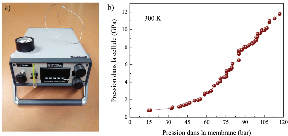
FIGURE 2.9 – a) Photographie de chargeur gaz manuel BETSA PDS 200 b) Évolution de la pression à l'intérieur de la cellule en fonction de la pression appliquée dans la membrane lors d'une mesure à température ambiante.
