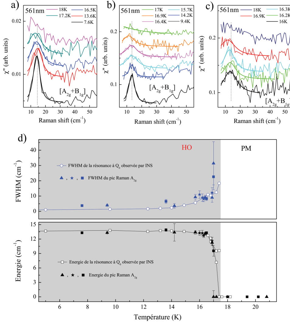
FIGURE 4.15 – Spectres Raman du pic A_{2g} pour différentes températures au dessus et en dessous de la transition vers l'ordre caché réalisés lors de plusieurs campagnes de mesures : a) dans le cryostat Absolut System avec une puissance laser de 5 mW, b) et c) dans le cryostat Oxford avec une puissance laser de 10 mW et 20 mW, respectivement. Les courbes en traits plein correspondent à des fits de Voigt pour lesquels nous fixons la largeur de la contribution Gaussienne par la résolution du spectromètre à 3 \text{ cm}^{-1} . Les spectres ont été décalés pour plus de clarté. Toutes les températures sont corrigées de l'échauffement laser. d) Dépendance en température de l'énergie et de la largeur à mi-hauteur (FWHM) du pic Raman A_{2g} (symboles pleins) et de la résonance mesurée à Q_0=(0,0,1) par diffusion inélastique de neutrons (INS) (symboles vides) [Bourdarot, 2010]. Les symboles pleins carrés, triangles et étoiles correspondent aux valeurs extraites respectivement des spectres a), b) et c). La zone grisée indique la plage de température de l'ordre caché.
