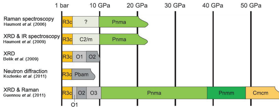
FIGURE 5.5 – Schéma résumant les différentes études expérimentales réalisées sur BiFeO 3 sous pression [Guennou, 2011]. Cet article de Guennou et al. présente une étude aboutie prouvant l'existence de trois phases orthorhombiques complexes (O 1 , O 2 et O 3 ) entre les phases R3c et Pnma.
