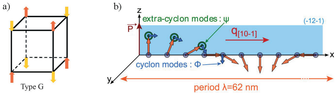
FIGURE 5.3 – a) Structure antiferromagnétique de type G dans BiFeO 3 . b) Spirale cycloïdale antiferromagnétique incommensurable de période 62 nm dans BiFeO 3 . Les excitations d'onde de spin dans le plan et hors du plan de la cycloïde sont appelées respectivement modes "cyclon" ( \phi ) et "extra-cyclon" ( \psi ). La cycloïde antiferromagnétique est contenue dans le plan (-12-1) et se propage dans la direction [10-1]. La polarisation électrique P , de direction [111], appartient au plan de la cycloïde antiferromagnétique (-12-1).
