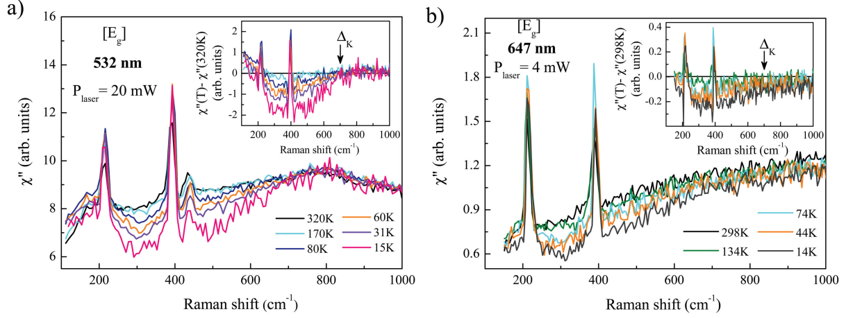
FIGURE 4.51 – Spectres Raman dans la symétrie E_g à différentes températures mesurés à 532 nm a) et 647 nm b). Le spectre à 15 K à 532 nm est normalisé, il a été réalisé avec une puissance laser de 2 mW. Les inserts montrent les réponses Raman à chaque température auxquelles ont été soustraites les réponses à température ambiante. Les flèches noires indiquent approximativement l'énergie de fermeture du gap Kondo \Delta_K . Tous les spectres ont été réalisés avec des échantillons d'URu 2 Si 2 polis. Toutes les températures reportées sont corrigées de l'échauffement laser.
