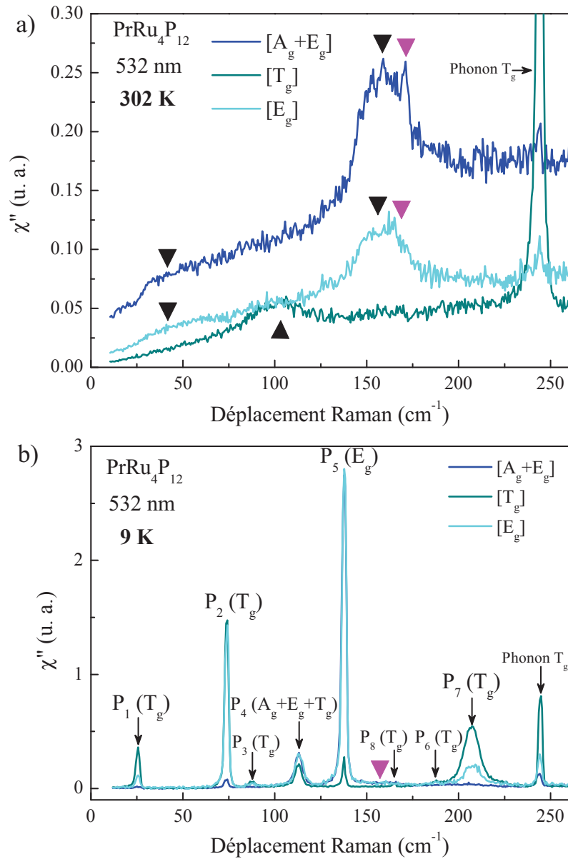
FIGURE 3.14 – a) Spectres Raman à basse énergie de \text{PrRu}_4\text{P}_{12} à température ambiante dans différentes symétries. Les flèches noires indiquent des excitations de champ cristallin. b) Spectres Raman à basse énergie de \text{PrRu}_4\text{P}_{12} à 9 K dans différentes symétries. Les excitations de champ cristallin sont nommées de \text{P}_1 à \text{P}_7 . \text{P}_8 désigne une nouvelle excitation étroite mesurée en [\text{T}_g] et assigné à un phonon (Cf. texte). Les flèches roses pour a) et b) indiquent une excitation qui pourrait être un mode de "rattling" des ions Pr (Cf. texte).
