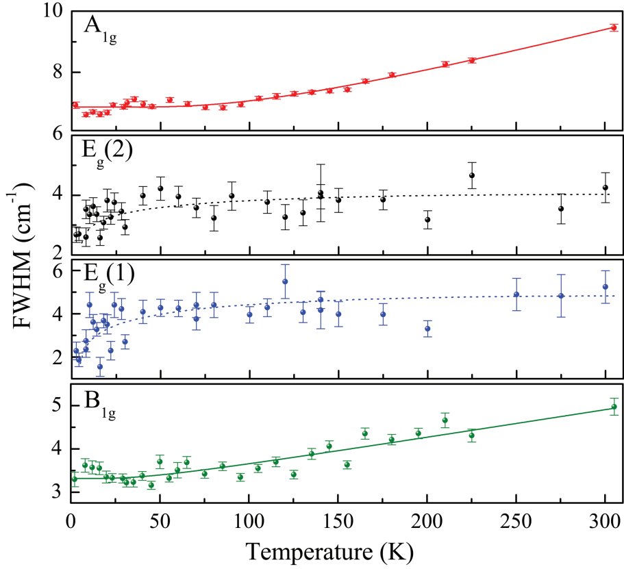
FIGURE 4.35 – Dépendance en température de la largeur à mi-hauteur des modes de phonon A_{1g} , E_g(1) , E_g(2) et B_{1g} . Les lignes continues représentent des ajustements avec un modèle anharmonique simple (Cf. texte). Les lignes en pointillés sont des guides pour les yeux.
