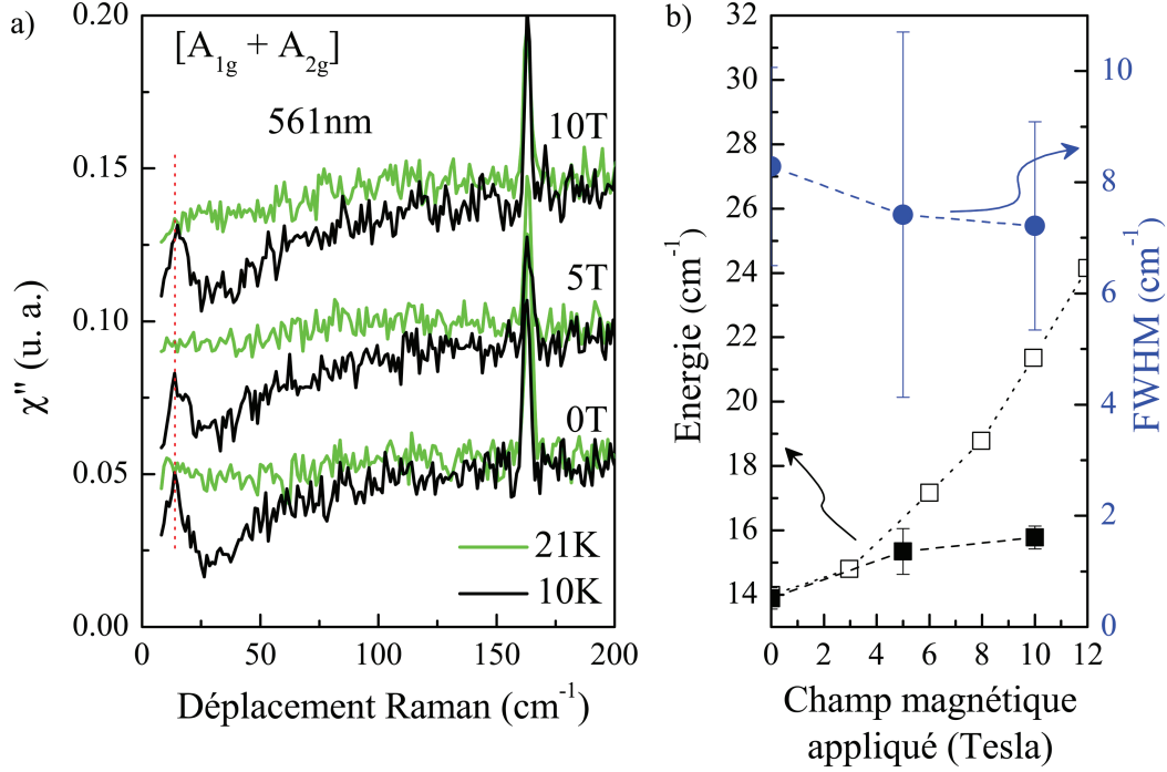
FIGURE 4.22 – a) Spectres Raman de URu 2 Si 2 dans la symétrie A 2g +A 1g , dans la phase d'ordre caché (10 K) et dans la phase paramagnétique (21 K) à 0, 5 et 10 T. Pour plus de clarté, les données ont été décalées en abscisse. b) Energie (échelle de gauche) et largeur (échelle de droite) du pic Raman d'ordre caché en fonction du champ magnétique appliqué. Les carrés vides correspondent à l'énergie de l'excitation Q 0 mesurée sous champ par INS [Bourdarot, 2004].
