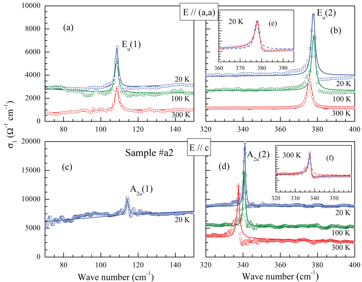
FIGURE 4.41 – Conductivité optique centrée autour de chaque phonon polaire dans URu 2 Si 2 à différentes températures. Pour (a) et (b) la lumière incidente est polarisée dans le plan (a, a) et pour (c) et (d) le long de l'axe c. Les lignes correspondent à un fit Drude-Lorentz. L'insert (e) montre le phonon E u (2) à 20 K décrit par un fit Lorentzien (ligne discontinue) ou un fit Fano (ligne continue). L'insert (f) est équivalent à (e) pour le mode phononique A 2u (2) à 300 K.
