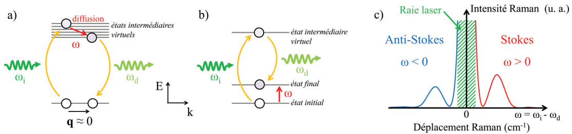
FIGURE 1.2 – a) Processus Raman de création d'un phonon de fréquence \omega . b) Processus Raman de création d'une paire électron-trou de fréquence \omega . c) Spectre Raman typique lors de la création (processus Stokes) ou de l'annihilation (processus Anti-Stokes) d'une excitation de fréquence |\omega| .
