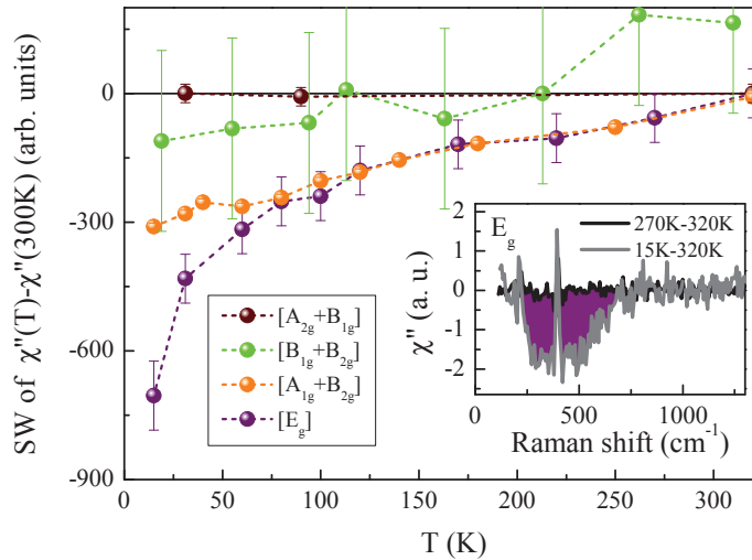
FIGURE 4.54 – Dépendance en température des poids spectraux normalisés des soustractions des réponses Raman \chi''(T) - \chi''(T_{\text{ambiante}}) dans les symétries [A_{2g} + B_{1g}] , [B_{1g} + B_{2g}] , [A_{1g} + B_{2g}] et [E_g] . L'insert montre un exemple : le poids spectral (en violet) extrait dans la symétrie E_g à 15K. Les poids spectraux extraits pour chaque symétrie ont été normalisés par rapport à l'intensité des phonons.
