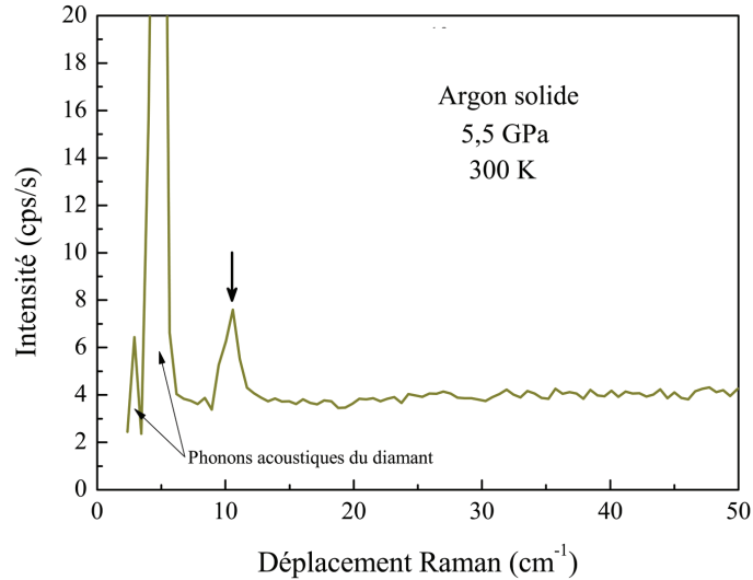
FIGURE 2.16 – Spectre Raman de l'argon réalisé dans la cellule de pression à 5,5 GPa. Le flèche noire pointe une excitation de l'argon solide à \sim 10,5 \text{ cm}^{-1} .
