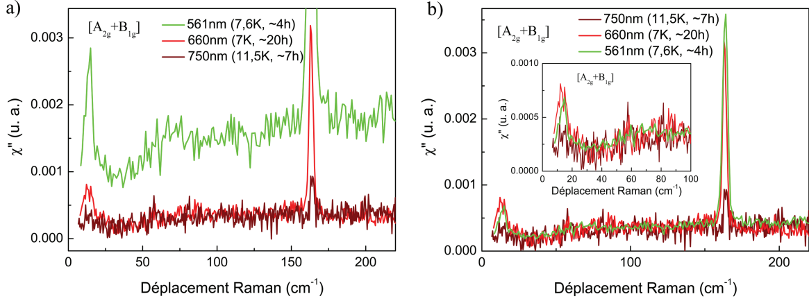
FIGURE 4.19 – a) Spectres Raman de URu 2 Si 2 dans la phase d’ordre caché dans la symétrie [A_{2g}+A_{1g}] à 561 nm, 660 nm et 750 nm. Les spectres sont normalisés à une puissance laser identique de 1 mW. b) Spectres Raman identiques à a) excepté la spectre à 561 nm qui a été normalisé afin que son continuum électronique coïncide avec celui des spectres à 660 nm et 750 nm. L’insert présente ces spectres à basses énergies.
