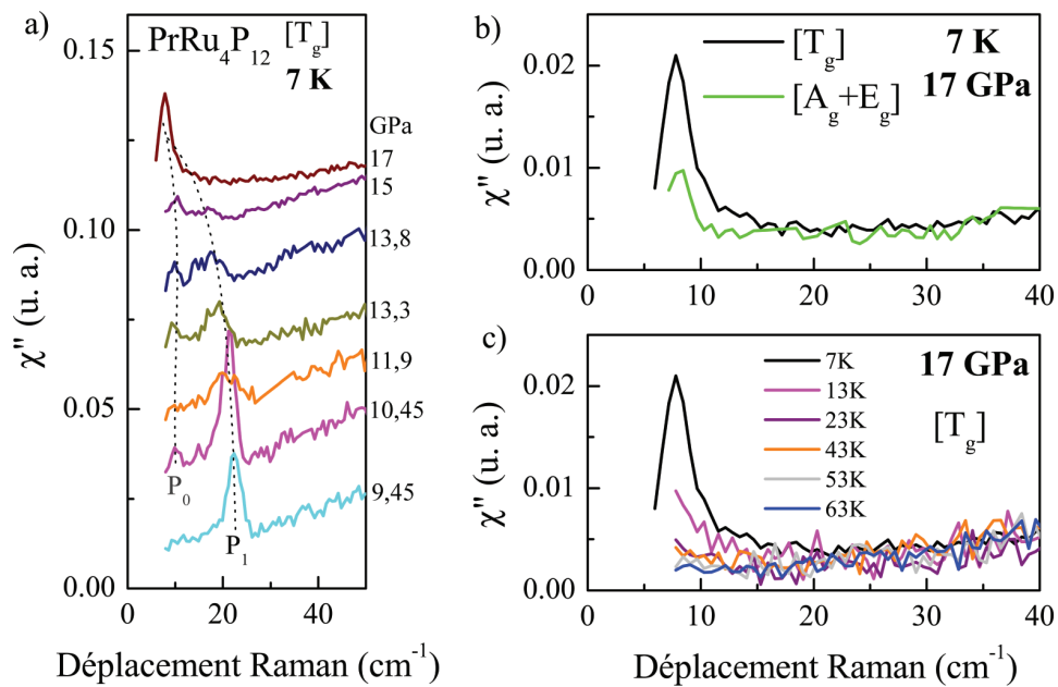
FIGURE 3.20 – a) Évolution sous pression des excitations P_0 et P_1 à 7 K dans la symétrie [T_g] . Les lignes pointillées sont des guides pour les yeux. b) Spectre à 17 GPa et 7 K dans les symétries [T_g] et [A_g + E_g] . c) Spectres Raman de basse énergie de \text{PrRu}_4\text{P}_{12} , à 17 GPa pour différentes températures dans la symétrie [T_g] .
