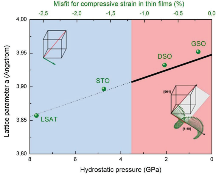
FIGURE 5.11 – Dépendance en pression du paramètre de maille a de BiFeO 3 "bulk" (ligne noire continue) extraite de la Réf. [Guennou, 2011] comparée aux valeurs discrètes (points verts) du paramètre de maille a dans les films minces de BiFeO 3 pour différents substrats [Sando, 2013, Sando, 2014]. La zone en rose indique la plage d'existence de la cycloïde antiferromagnétique et la zone bleue indique la présence de l'ordre antiferromagnétique homogène. Pour les films minces, la structure est R3c sur toute la plage de contrainte; pour les cristaux 3D, la zone rose est R3c et la zone bleue correspond aux phases O 1 , O 2 et O 3 .
