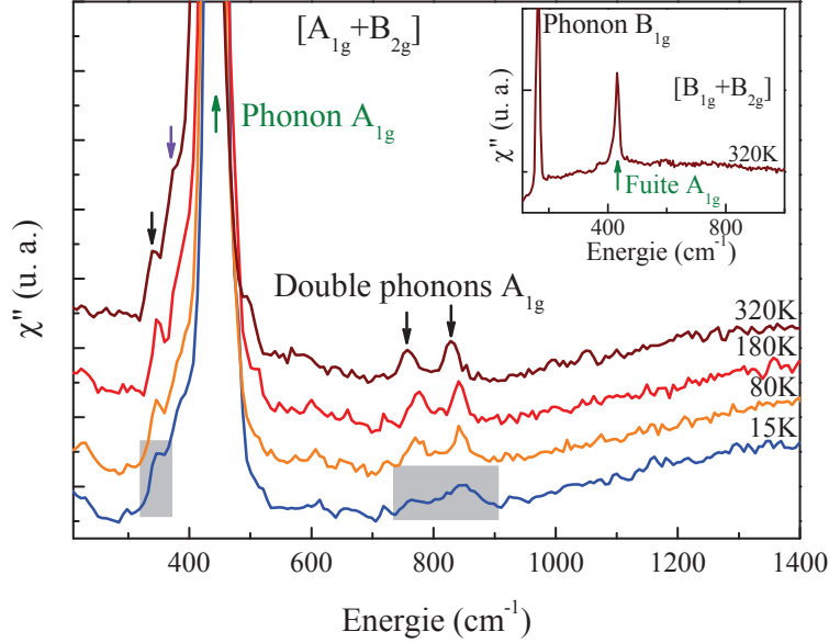
FIGURE 4.40 – Spectre Raman sur une grande plage d'énergie dans la symétrie A_{1g} + B_{2g} à différentes températures. Les spectres ont été décalés en ordonnées pour plus de clarté. La flèche verte indique le centre du phonon A_{1g} . Une fuite du phonon E_g(2) est observée à 394 \text{ cm}^{-1} (flèche violette). Trois nouveaux pics indiqués par des flèches noires, sont observés à environ 350 \text{ cm}^{-1} et 800 \text{ cm}^{-1} . Les aires grisées correspondent aux plages d'énergie possibles pour des processus de diffusion phononiques double d'après les calculs de P. Przemek (Cf. FIG. 4.49). L'insert montre un spectre Raman sur une grande plage d'énergie dans la symétrie B_{1g} + B_{2g} à 310K.
