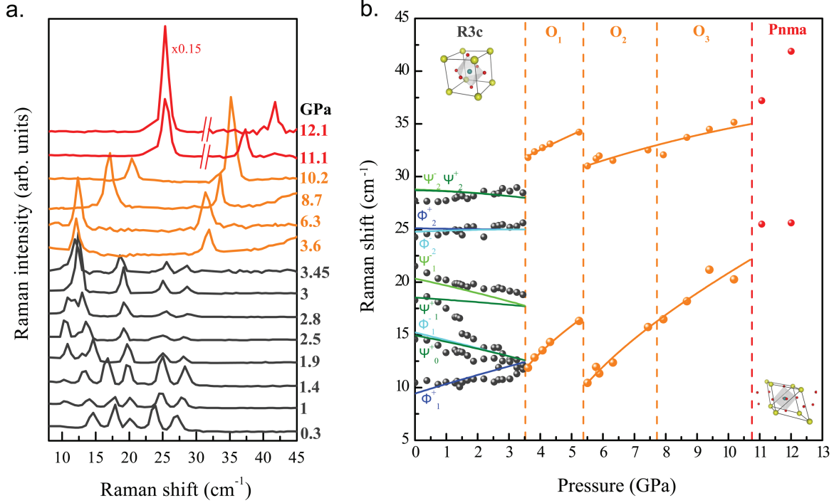
FIGURE 5.10 – a) Spectres Raman des excitations d’onde de spin dans \text{BiFeO}_3 à différentes pression. Les spectres en gris foncé, orange et rouge correspondent respectivement aux excitations d’onde de spin dans les structures R3c, O_{1,2,3} et Pnma. b) Énergies des excitations d’onde de spin dans \text{BiFeO}_3 de 0 à 11 GPa. Les lignes pleines sont des ajustements utilisant le modèle théorique de R. de Sousa et certains paramètres issus du calcul numérique de D. Wang (Cf. texte). Les lignes verticales discontinues indiquent les quatre transitions structurales.
