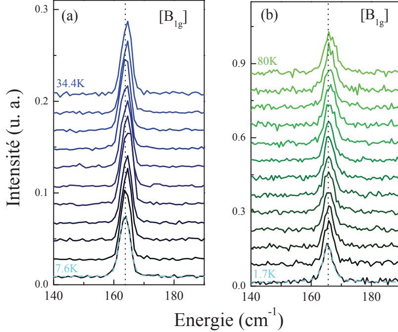
FIGURE 4.37 – Dépendance en température des spectres Raman du phonon B_{1g} mesurés pour un échantillon clivé dans le cryostat Absolute System (a) et pour un échantillon poli dans le cryostat Oxford (b). Les lignes discontinues bleues aux basses températures sont des fits Lorentziens.
