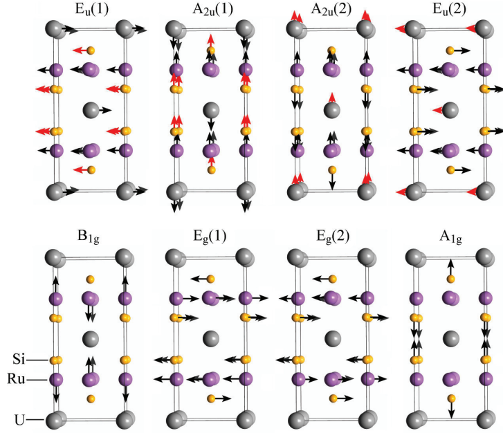
FIGURE 4.31 – Schéma des déplacements atomiques des modes de phonons dans URu 2 Si 2 observés en conductivité optique (haut) et en Raman (bas). Les modes de phonons sont rangés par énergie croissante de la gauche à la droite. Les modes en rouge sont de très faibles intensités selon les calculs ab-initio.
