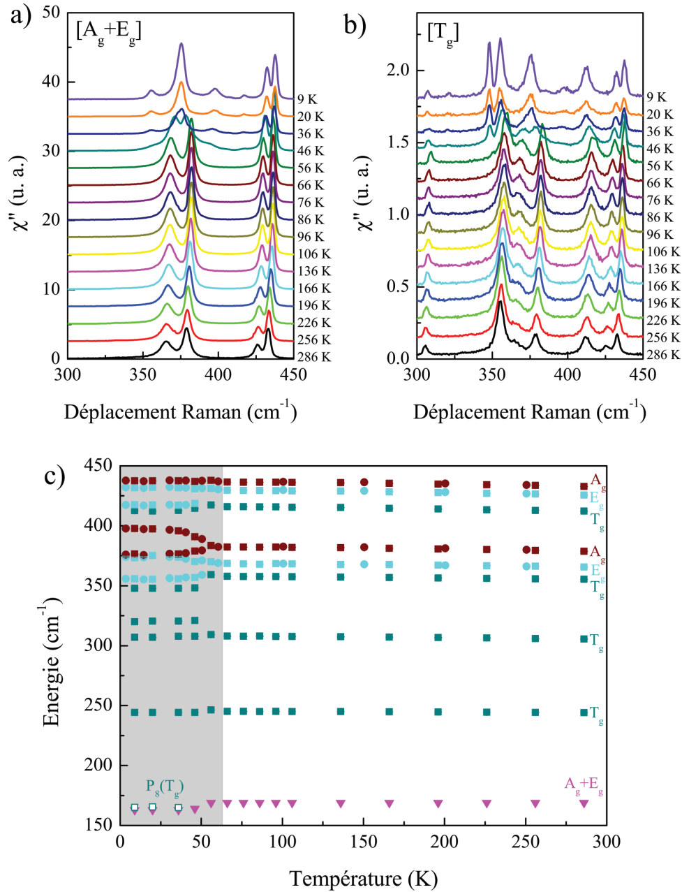
FIGURE 3.12 – a) Spectres Raman des phonons de \text{PrRu}_4\text{P}_{12} de 286 K à 9 K dans la symétrie [A_g + E_g] . b) Spectres Raman des phonons de \text{PrRu}_4\text{P}_{12} de 286 K à 9 K dans la symétrie [T_g] . Ces spectres ont été réalisés avec l'échantillon #1. c) Evolution en température de l'énergie des phonons dans \text{PrRu}_4\text{P}_{12} . La zone grisée en dessous de 63 K correspond à la phase isolante. Les carrés et les ronds correspondent aux mesures faites respectivement sur les échantillons #1 et #2. Les triangles roses correspondent au mode [A_g + E_g] interprété comme provenant du mouvement de "rattling" des ions Pr dans les cages de P. Le mode P_8 , assigné à un phonon, est reporté par les carrés vides. Ces deux modes de plus basses énergies sont visibles dans la section concernant les excitations de champ cristallin et ont été mesurés sur l'échantillon #1.
