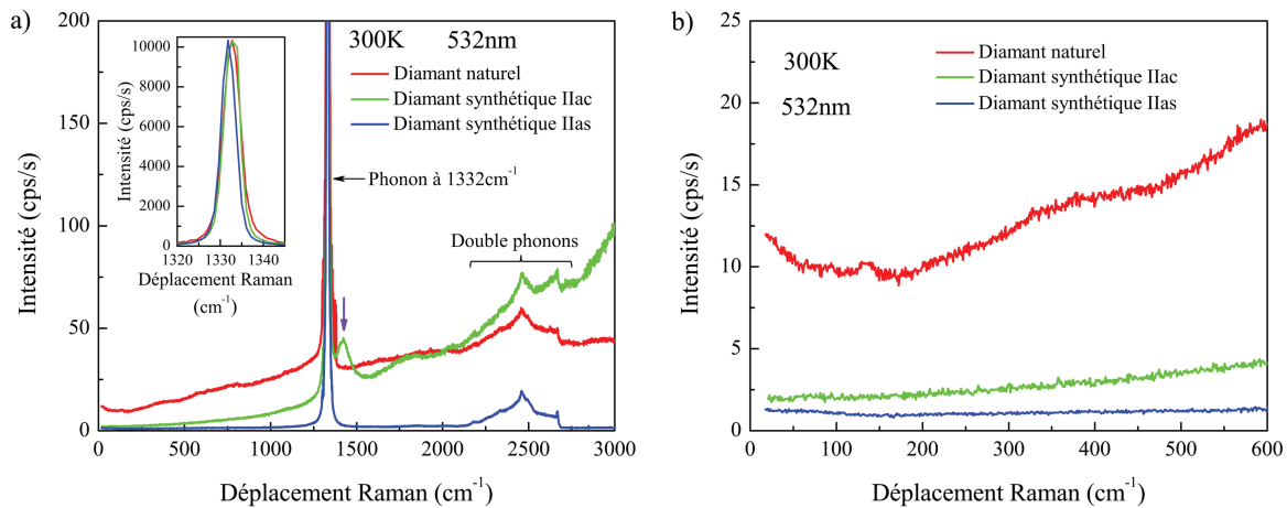
FIGURE 2.13 – a) Spectres Raman de trois diamants différents : un diamant naturel et deux diamants synthétiques (type IIas et IIac, achetés chez almax-easylab). L'insert montre le phonon du diamant à 1332\text{ cm}^{-1} . Les spectres ont été normalisés entre eux via l'intensité du phonon à 1332\text{ cm}^{-1} . La flèche mauve pointe un pic observé uniquement dans le spectre du diamant synthétique IIac. b) Spectres Raman des trois diamants à basse fréquence.
