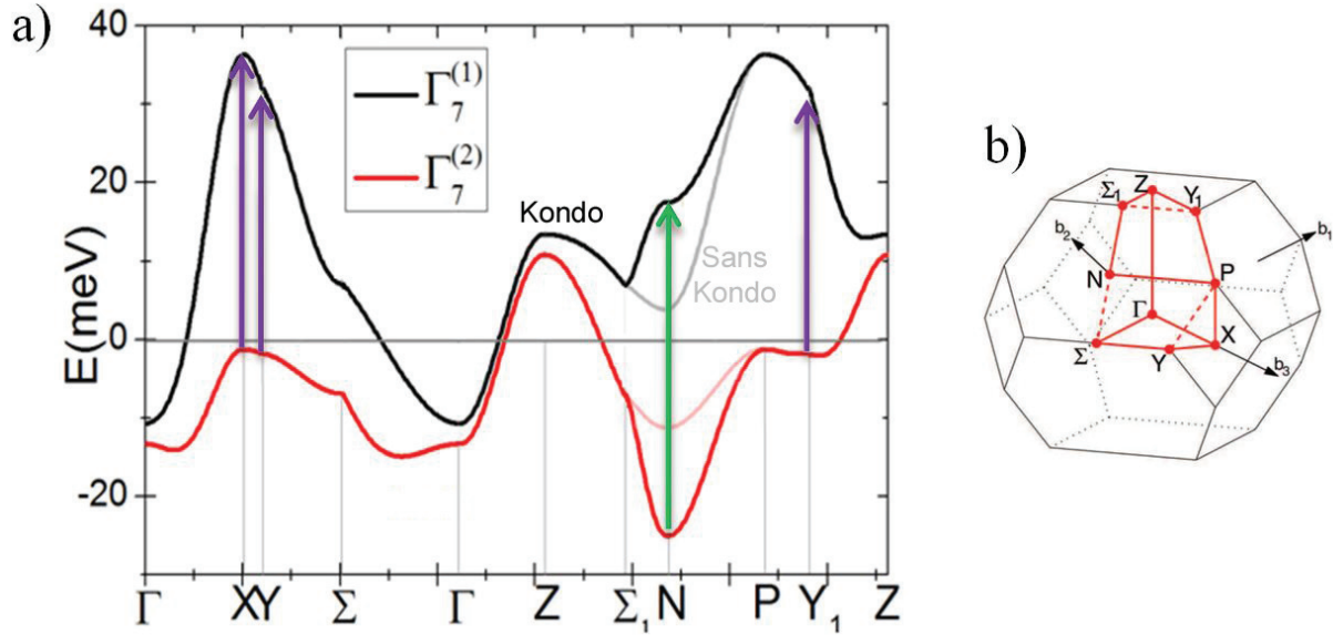
FIGURE 4.56 – a) Dispersion des bandes électronique \Gamma_7^{(1)} et \Gamma_7^{(2)} calculée par X. Montiel grâce au modèle des liaisons fortes développé par Rau [Rau, 2012]. En foncé, la dispersion électronique dans la phase Kondo (terme de saut entre les atomes d’uranium premiers voisins t_{12} = 0.7 ). En clair, la dispersion électronique dans la phase paramagnétique sans hybridation Kondo (terme de saut t_{12} = 0 ). Les flèches violettes et vertes indiquent respectivement les transitions inter-bandes E_g et A_{1g} aux endroits de l’espace réciproque où elles fournissent les vertex Raman les plus intenses. b) Zone de Brillouin de la phase paramagnétique.
