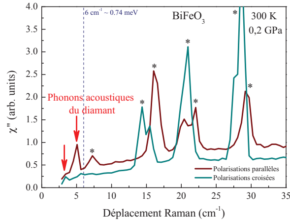
FIGURE 2.15 – a) Spectres Raman à 0,2 GPa des excitations d’onde de spin (*) du composé multiferroïque \text{BiFeO}_3 . Les flèches rouges pointent les phonons acoustiques du diamant supérieur de la cellule de pression à \sim 3 \text{ cm}^{-1} et \sim 5 \text{ cm}^{-1} .
