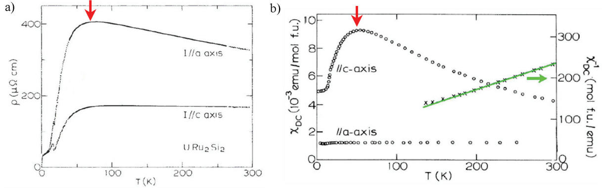
FIGURE 4.2 – a) Dépendance en température de la résistivité dans URu 2 Si 2 [Palstra, 1986a] b) Susceptibilité magnétique DC (échelle de gauche) et susceptibilité inverse (échelle de droite) obtenues à 2T dans URu 2 Si 2 [Palstra, 1985]. Les flèches rouges indiquent les maxima de ces deux quantités correspondant à la température de cohérence T_{coh} .
