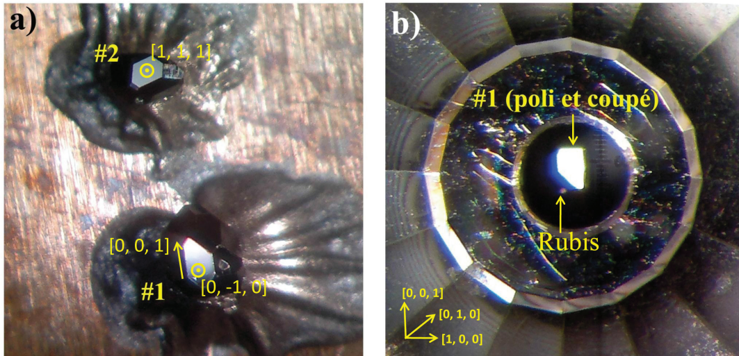
FIGURE 3.10 – a) Photographie des deux monocristaux de PrRu 4 P 12 (nommés #1 et #2) utilisés pour notre étude Raman. b) Photographie de l'échantillon de PrRu 4 P 12 à l'intérieur de la cellule de pression. Celui-ci provient de l'échantillon #1 après polissage et découpage. Un rubis ball à l'intérieur de la cellule est utilisé comme manomètre.
