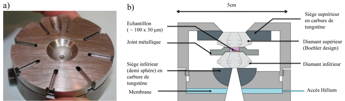
FIGURE 2.8 – a) Photographie de la cellule de pression. b) Schéma de la cellule de pression.
