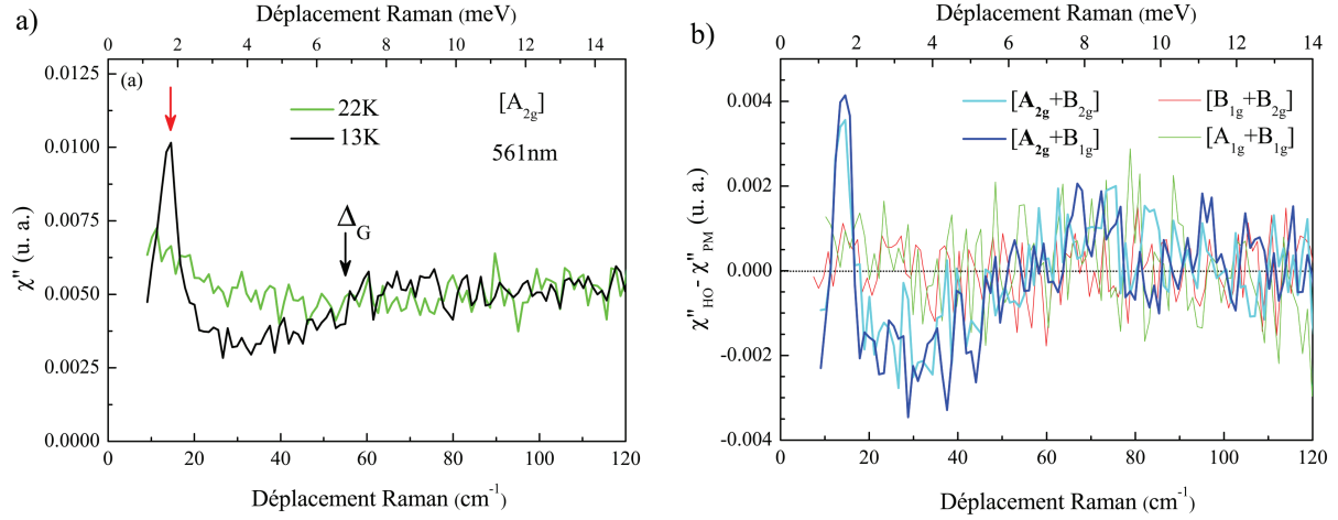
FIGURE 4.13 – a) Spectres Raman de URu 2 Si 2 en symétrie A 2g pure (Cf. Annexe A.3) dans la phase d'ordre caché (13 K) et dans la phase paramagnétique (22 K). b) Soustractions des réponses Raman dans la phase d'ordre caché et la phase paramagnétique pour toutes les symétries sondées. Tous les spectres ont été mesurés à la même puissance laser. Les spectres contenant la réponse B 1g ont été normalisés par rapport à l'intensité du phonon B 1g .
