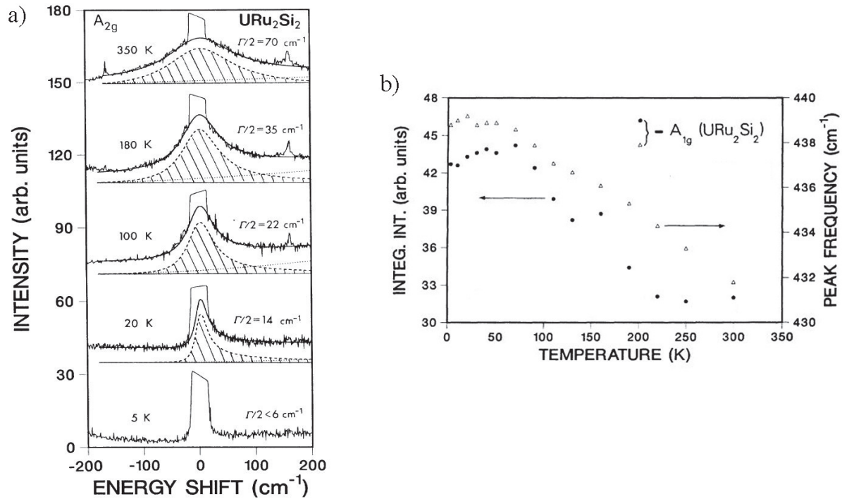
FIGURE 4.9 – a) Excitation quasi-élastique observée par Cooper et al. par spectroscopie Raman [Cooper, 1987] dans la symétrie A 2g . b) Intensité intégrée et énergie du phonon A 1g en fonction de la température, extraites de [Cooper, 1987].
