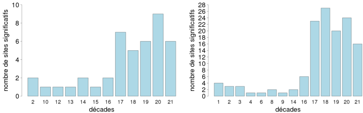
Figure 41: Histogrammes représentant le nombre de sites par décade où le meilleur R^2 significatif au seuil de 1% ( p -value < 0,01) est obtenu entre le wg_2 décadaire, simulé avec le jeu de simulations DIF1-NRT et le LAI décadaire GEOV1. A gauche, les cultures de type C3 et à droite les prairies naturelles.
