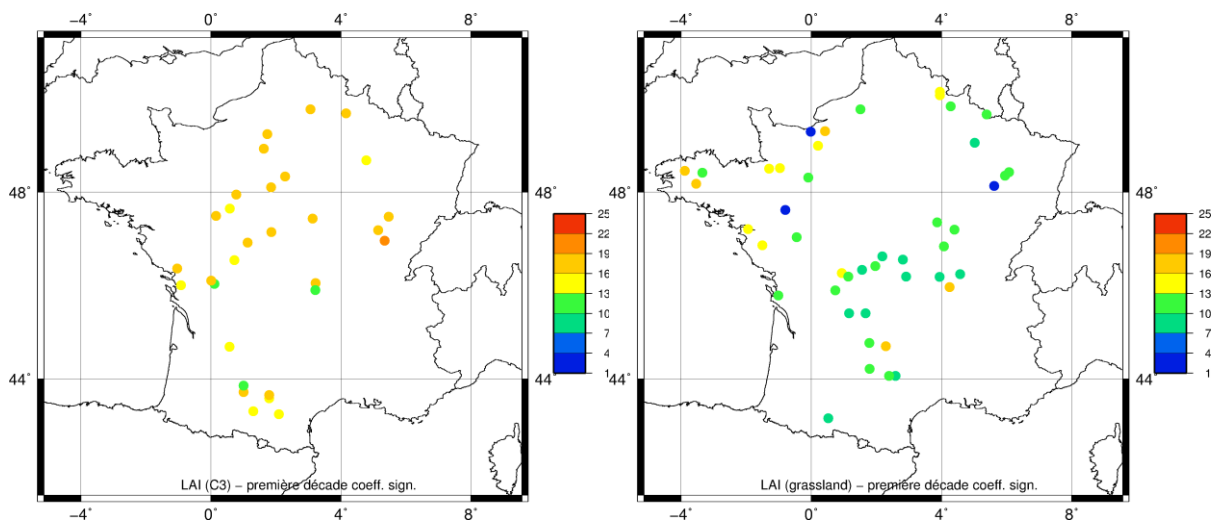
Figure 17: Cartes illustrant les premières décades pour lesquelles on obtient un R^2 significatif ( p -value < 0,01) entre le wg_2 décadaire et le LAI décadaire simulés avec le jeu de simulations DIF1-NRT, pour les cultures de type C3 (à gauche) et pour les prairies naturelles (à droite).
