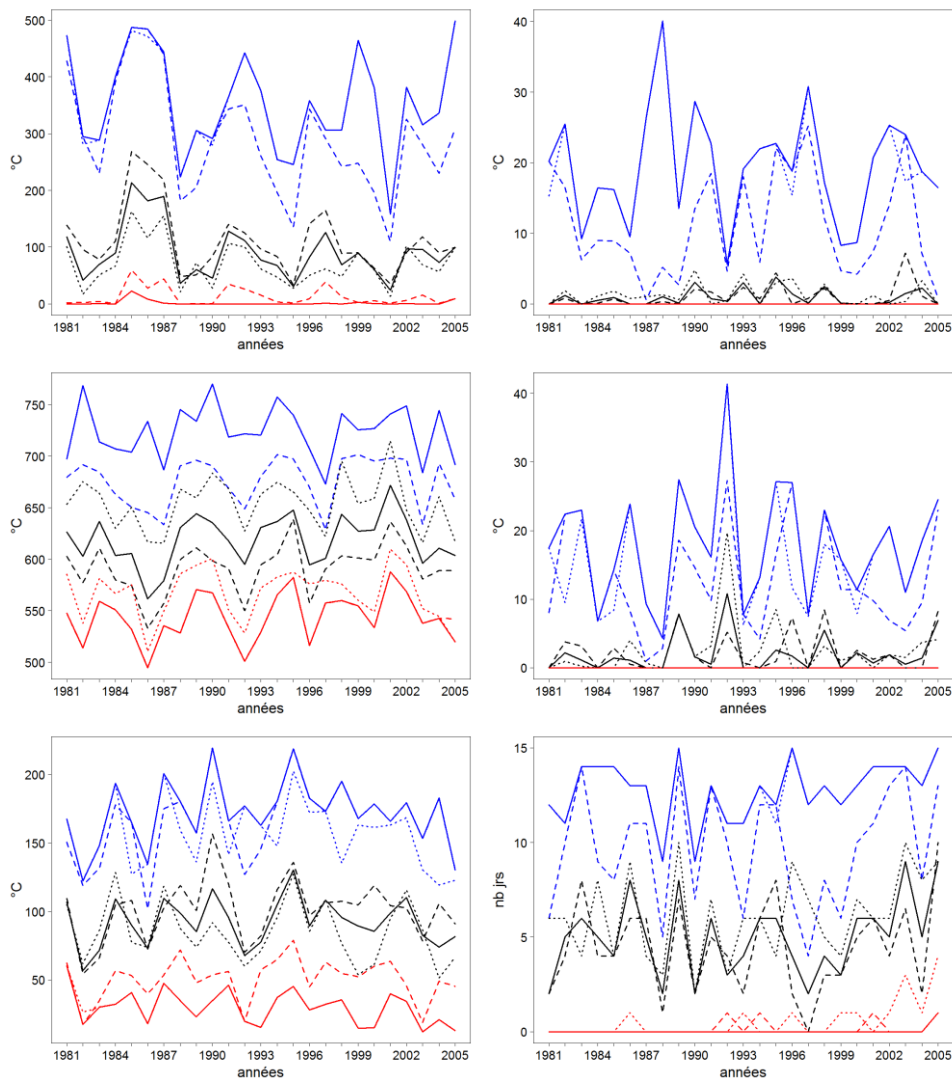
Figure 68: Évolution temporelle des variables thermiques sur la période 1981-2005, obtenues avec le jeu de simulations de référence. En partant de haut à gauche jusqu'en bas à droite, sont représentées les variables : « somme des températures minimales inférieures à 0°C entre la date de semis et le stade épi à 1 cm », « somme des températures minimales inférieures à 0°C entre les stades épi à 1 cm et 2 nœuds », « somme des températures moyennes supérieures à 0°C entre les stades épi à 1 cm et épiaison », « somme des températures maximales supérieures à 25°C entre les stades méiose et floraison », « somme des températures minimales inférieures à 14°C entre les stades épiaison et maturité » et « nombre de jours où la température maximale est supérieure à 25°C ». La médiane de l'ensemble des sites est représentée en trait plein, celle de la région nord en tirets, en pointillés pour la région sud. La valeur médiane est en noir, la valeur minimale en rouge et la valeur maximale en bleu.
