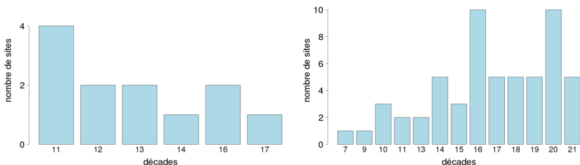
Figure 26: Histogrammes représentant le nombre de sites par décade où le meilleur R^2 significatif au seuil de 1% ( p -value < 0,01) est obtenu entre le wg_2 décadaire, simulé avec le jeu de simulations DIF1-NRT, et le rendement final issu d'Agreste. A gauche, les cultures de type C3 et à droite les prairies naturelles.
