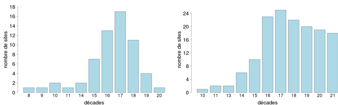
Figure 23: Histogrammes représentant le nombre de sites par décade où le meilleur R^2 significatif au seuil de 1% ( p -value < 0,01) est obtenu entre le wg_2 décadaire et le B_{agX} , simulés avec le jeu de simulations DIF1-NRT. A gauche, les cultures de type C3 et à droite les prairies naturelles.
