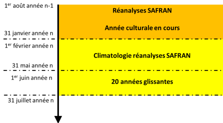
Figure 52: Forçages météorologiques utilisés pour le jeu de simulations de contrôle « clim » jusqu'au 31 juillet de l'année culturelle.
