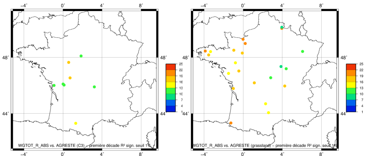
Figure 24: Cartes illustrant les premières décennies pour lesquelles on obtient un coefficient de détermination significatif ( p -value < 0,01) entre le wg_2 décennal, simulé avec le jeu de simulations DIF1-NRT, et le rendement final issu d'Agreste. A gauche, les cultures de type C3 et à droite les prairies naturelles.
