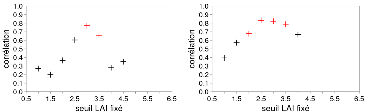
Figure 29: R 2 calculés entre le rendement final issu d'Agreste et la série de wg_2 simulés avec le jeu de simulations DIF1-NRT sur la période 1994-2010. La valeur de wg_2 est obtenue lorsque différents seuils de LAI ont été atteints. Sont représentés en rouge les R 2 significatifs au seuil de 1% (p-value > 0,01). A gauche, le R 2 obtenu pour le rendement de l'orge d'hiver pour le département du Puy-De-Dôme (63). A droite le R 2 obtenu pour le rendement des prairies naturelles pour le département du Maine-et-Loire (49).
