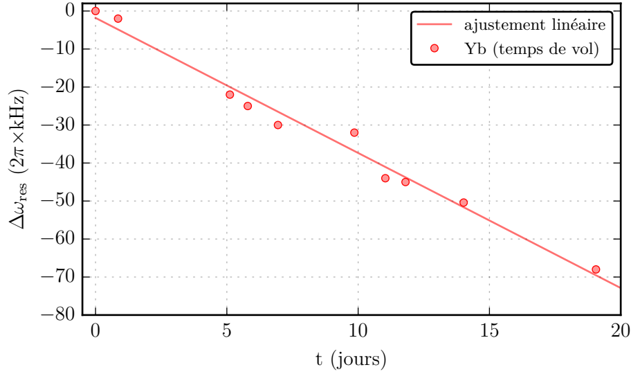
FIGURE 4.6 – Dérive résiduelle de la cavité après optimisation de sa température, mesurée par spectroscopie en temps de vol sur un condensat d'ytterbium.
