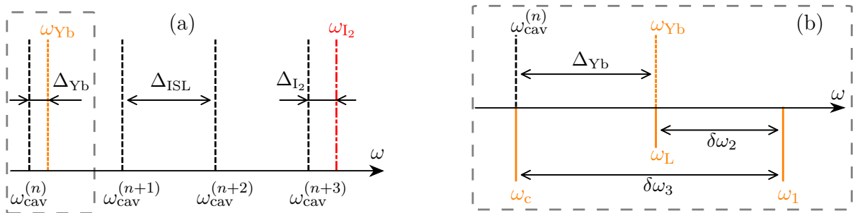
FIGURE 4.1 – Principe de l'asservissement du laser « d'horloge ». (a) Représentation des résonances de l'ytterbium et du diode par rapport à celles de la cavité. (b) Agrandissement autour de la résonance de l'ytterbium. Les différentes composantes spectrales du laser d'horloge sont représentées.
