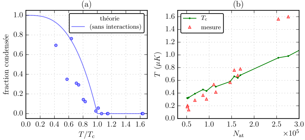
FIGURE 2.29 – (a) Évolution de la fraction condensée en fonction du rapport T/T_c . La température critique T_c est calculée pour chaque point en utilisant le nombre d’atomes total mesuré et les fréquences de piégeages, estimées à partir des mesures effectuées à haute puissance. La courbe théorique correspond au modèle décrit par l’équation (2.37), sans paramètre libre. (b) Évolution jointe de la température de l’échantillon et de la température critique en fonction du nombre d’atomes. La condensation a lieu lorsque les deux courbes se croisent.
