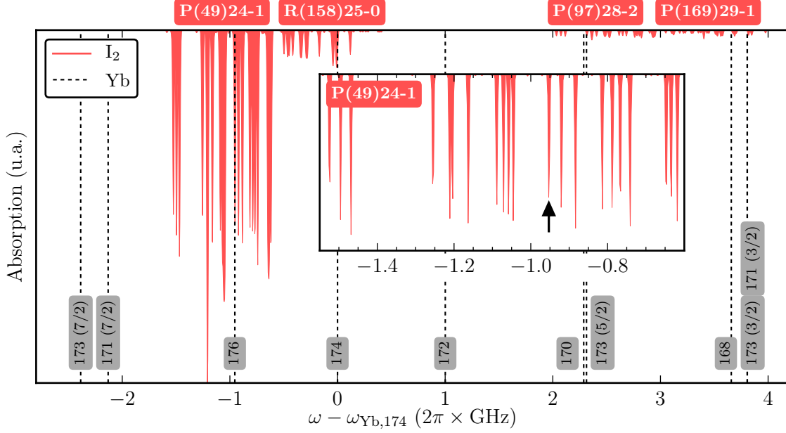
FIGURE 2.4 – Spectre d'absorption théorique du diode (rouge) aux alentours de la transition ^1S_0 \rightarrow ^3P_1 de l'ytterbium. Les transitions des différents isotopes de l'ytterbium sont tracées en pointillés. L'origine de l'axe des fréquences correspond à la transition de l'isotope 174. En insert : détail de la structure hyperfine de la transition P(49)24-1 utilisée pour l'asservissement du laser. La flèche désigne la composante servant de référence (voir aussi figure 2.6). Ce spectre a été calculé à l'aide d'un programme qui nous a été généreusement fourni par l'équipe d'Eberhard Tiemann de l'université de Hanovre.
