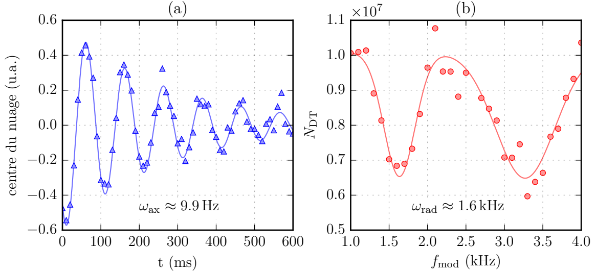
FIGURE 2.21 – (a) Mesure de la fréquence axiale du piège dipolaire à 1070 nm. La position du centre de masse du nuage est mesurée pour différents temps après le déplacement soudain du foyer du laser. (b) Mesure de la fréquence radiale du piège dipolaire à 1070 nm par excitation paramétrique. La profondeur du piège est modulée à f_{mod} (10% de modulation pendant 1 s), puis le nombre d'atome est mesuré. On s'attend à des pertes par chauffage pour f_{mod} = 2f_{rad} . Nous voyons aussi des pertes pour f_{mod} = f_{rad} , pouvant s'expliquer par l'anharmonicité du piège, ou par la présence d'harmoniques d'ordre supérieur dans la modulation. La fonction utilisée pour l'ajustement comprend deux résonances gaussiennes, le rapport entre les fréquences de résonance étant fixé à 2.
