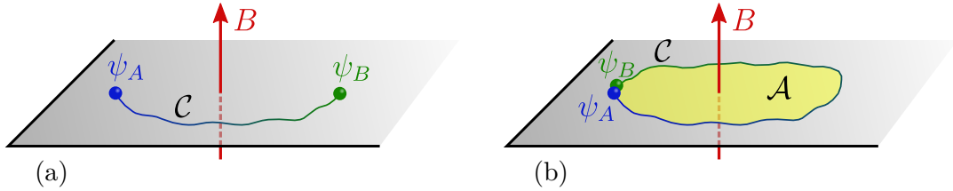
FIGURE 1.1 – Illustration de l'effet Aharonov-Bohm. (a) Exemple de trajectoire ouverte. (b) Trajectoire fermée C définissant une surface A .
