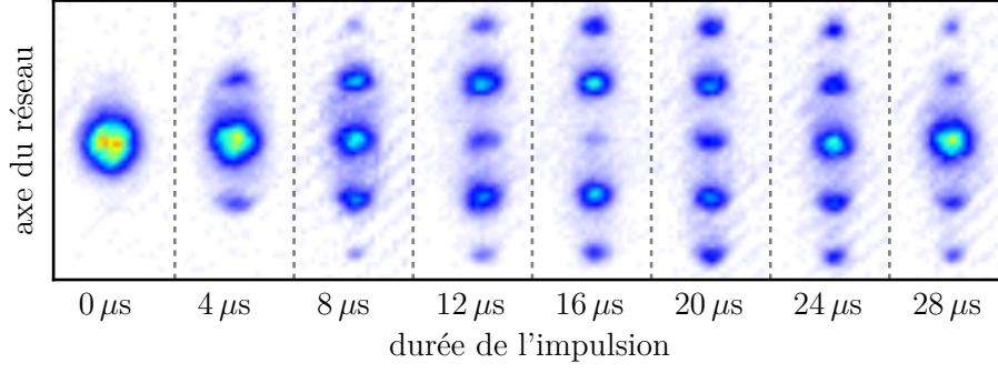
FIGURE 2.31 – Images de diffraction obtenue pour un réseau de profondeur U_0/E_r \approx 21 , pour différentes durées de l'impulsion lumineuse. On observe bien une série de pics équidistants, séparés d'une distance correspondant, après temps de vol, à une différence d'impulsion de 2\hbar k .
