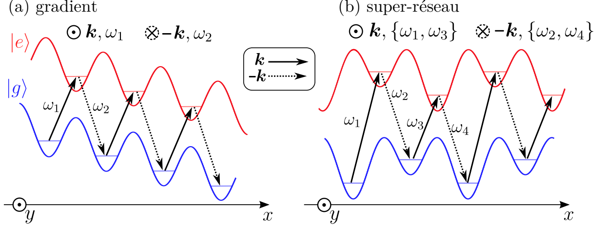
FIGURE 1.8 – Principe de la rectification du flux. Un potentiel est ajouté au réseau suivant x pour désaccorder les fréquences associées à deux effets tunnels successifs, ce qui permet d'utiliser deux lasers contra-propageants – vecteurs d'onde \mathbf{k} et -\mathbf{k} – pour restaurer alternativement l'effet tunnel suivant x . Le potentiel peut être linéaire (a) ou bien consister en un super-réseau (b). Les transitions associées aux lasers de vecteurs d'onde \mathbf{k} et -\mathbf{k} sont respectivement représentées par des flèches en traits pleins et pointillés.
