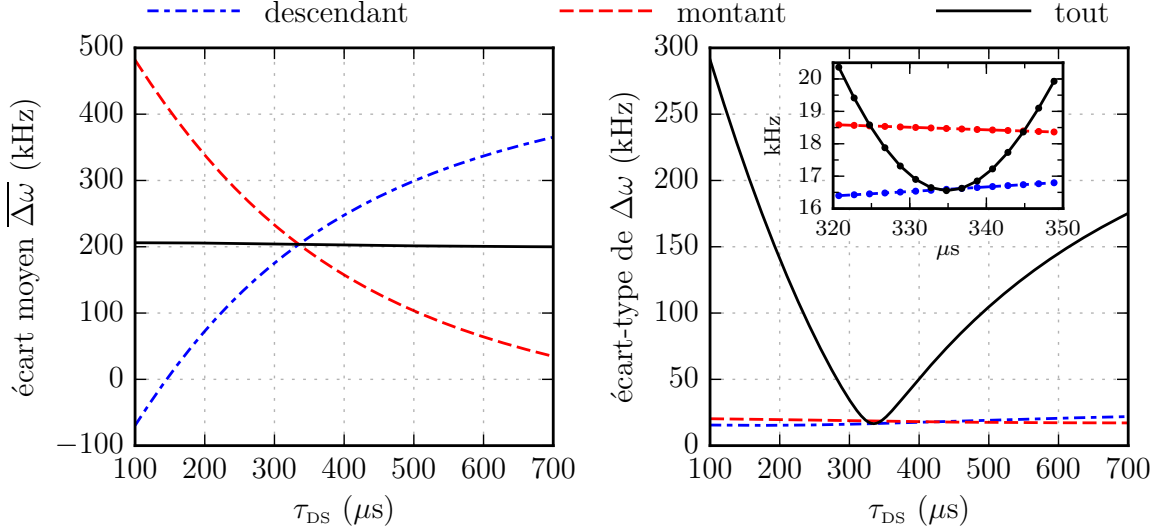
FIGURE 3.16 – Effet du filtre de la détection synchrone sur la mesure. (a) Valeur moyenne de l'écart estimé entre la résonance de la cavité et celle du diode en fonction de la constante de temps \tau_{DS} utilisée pour modéliser le filtre de la détection synchrone. On a distingué les sous-ensembles des balayages de fréquence ascendants (rouge interrompu) et descendants (bleu mixte). La moyenne de l'ensemble des mesures est aussi tracée (noir continu) (b) Écart-type en fonction de \tau , pour les mêmes ensembles que (a). L'insert montre un agrandissement autour du \tau_{DS} optimal.
