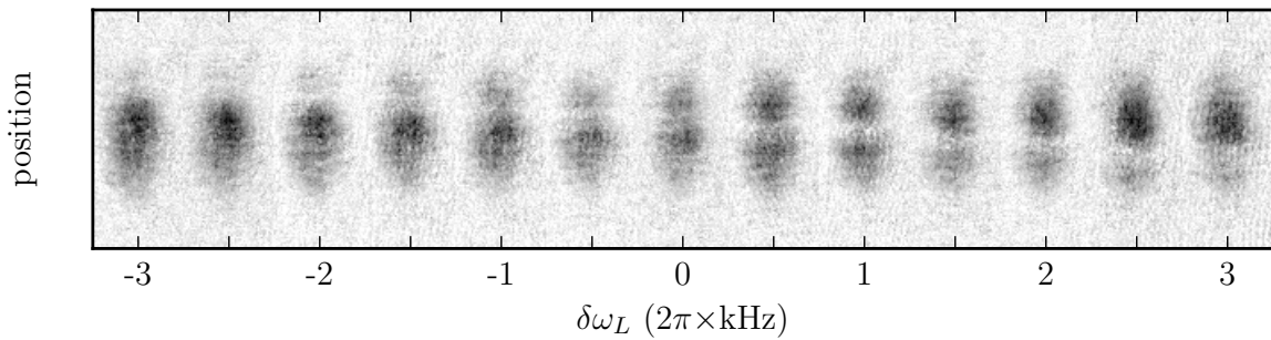
FIGURE 4.14 – Profils de densités observés pour différentes fréquences du laser de spectroscopie avec la séquence illustrée dans la figure 4.13. Le laser se propage du haut vers le bas dans les images. On observe bien une tranche dans le profil, correspondant à la classe de vitesse résonante avec le laser. L’amplification de la largeur Doppler dans la direction du laser se traduit par une plus grande extension spatiale du nuage dans cet axe, visible si l’on compare aux images de la figure 4.12.
