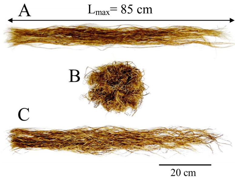
Figure 72 Photographie de la filasse (A), des étoupes brutes (B) et des étoupes démêlée et alignées (C).
