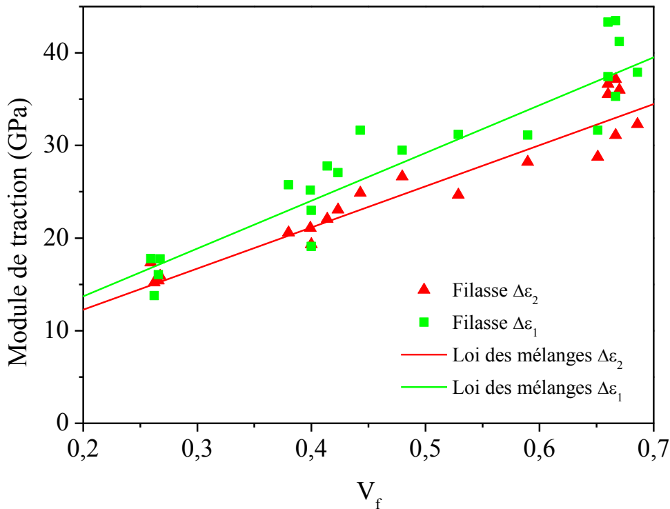
Figure 91 Comparaison des rigidités des composites à renforts UD pour deux gammes de déformation, en fonction de la fraction volumique de fibres. Chaque point représente une éprouvette. Les données sont présentées pour la filasse.
