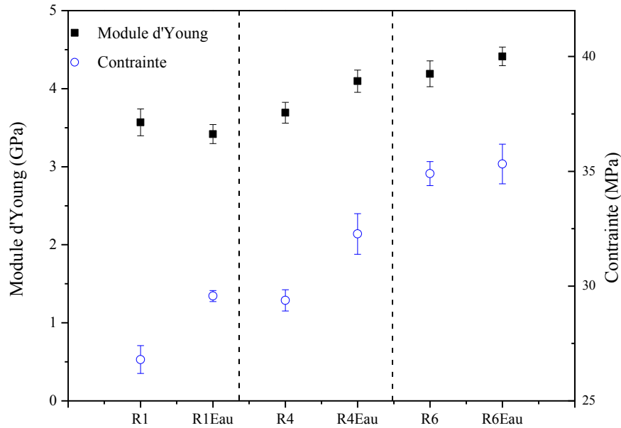
Figure 69 Propriétés mécaniques en traction des matériaux injectés renforcés par les fibres R1, R4 et R6 ainsi que ces mêmes lots traités à l'eau. Module d'Young et contrainte maximale.
