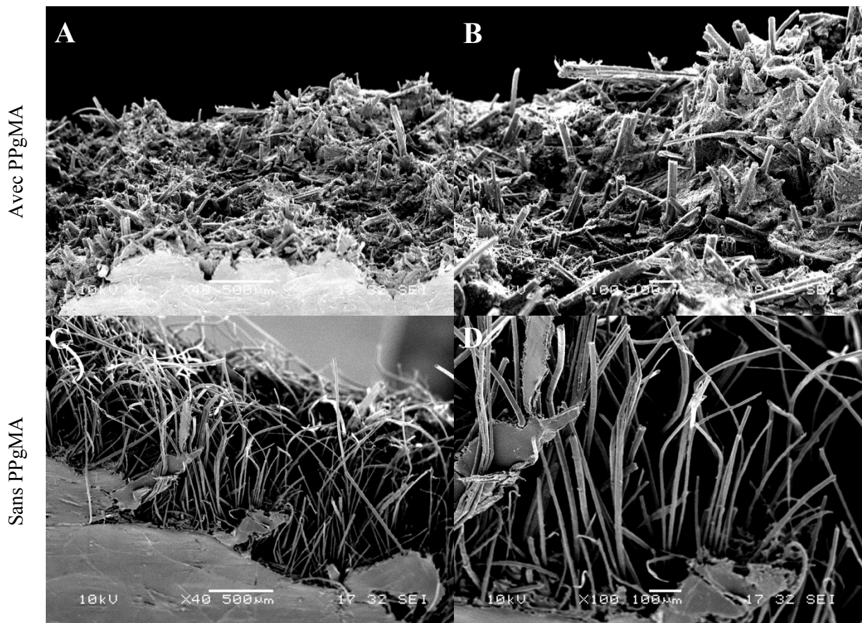
Figure 109 Observation par MEB de faciès de rupture en traction dans la direction MD de composites à matrice PP à renfort hydrolié. A et B : Avec agent couplant PPgMA (4%). C et D : Sans agent couplant. V_f=28,6 \% .
