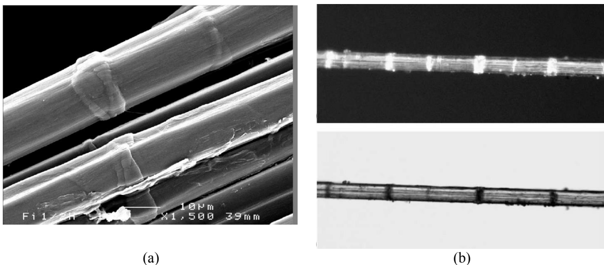
Figure 14 (a) Exemple de défauts observé au MEB (Baley, 2002) (b) Kink bands sur une fibre élémentaire de lin observé par microscopie optique en lumière polarisée (haut) et non polarisée (bas), diamètre de fibres ca. 23µm (Andersons et al., 2009a).
