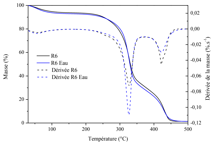
Figure 68 Analyse thermogravimétrique des échantillons R6 et R6Eau.
