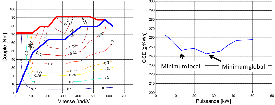
(a) Cartographie de rendement moteur EB0 avec représentation de l'OOL en bleu
