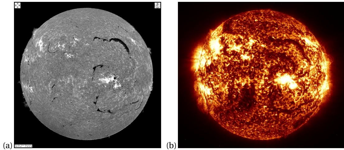
FIGURE 5.1. – (a) Images de BBSO en H\alpha 656.3 nm et de (b) SoHO/EIT He II 30.4 nm à la même date, le 3 janvier 2001.
