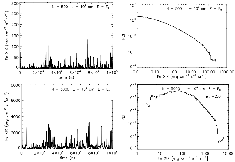
FIGURE 3.2. – Séries temporelles (à gauche) et distributions (à droite) des intensités simulées dans la raie du Fe XIX 111.8nm ( \log T_{\max} = 6.9 ) dans des boucles de demi-longueur L = 10\text{Mm} , constituées de N = 500 brins (en haut) ou N = 5000 brins (en bas), et soumises au chauffage issu de l'automate cellulaire avec une puissance de dissipation moyenne de 5 \times 10^{-4} \text{W} \cdot \text{m}^{-3} . Figure 7 de Parenti et al. (2006).
