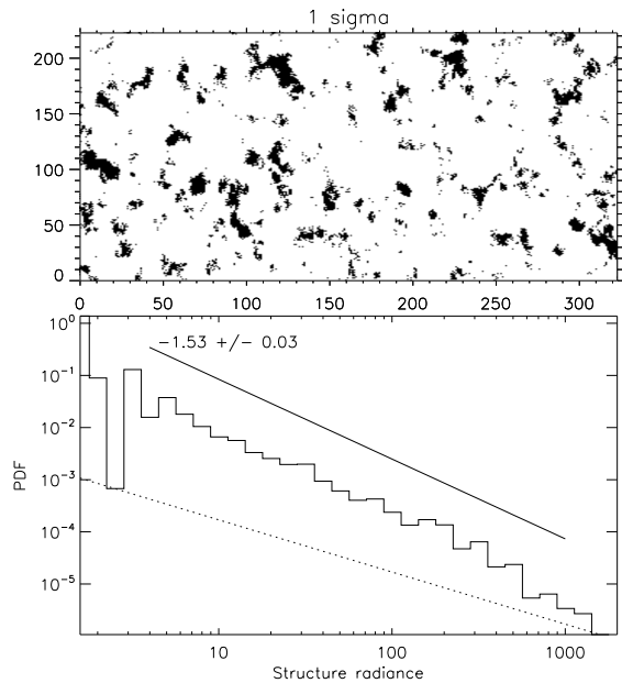
FIGURE 4.7. – En haut: structures (pixels noirs) dépassant un seuil du maximum de la radiance spectrale de S VI 93.3 nm, sur une partie du champ central le 21 juillet 1996. En bas: distribution de probabilité de la radiance spectrale intégrée sur ces structures, et ajustement d'une loi de puissance. La ligne pointillée représente une structure par barre d'histogramme (celles-ci étant de largeur variable). Fig. 9 de Buchlin et al. (2006) .
