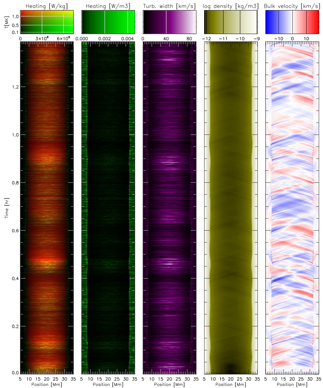
FIGURE 3.5. – De gauche à droite : température et chauffage par unité de masse, chauffage par unité de volume, largeur turbulente (largeur gaussienne correspondant à la moyenne RMS de la vitesse u_{\perp} de SHELLATM), logarithme de la masse volumique, et vitesse longitudinale, en fonction de la position dans la boucle et du temps, pour la suite de la simulation de la Fig. 3.4. Les échelles de couleur sont indiquées en haut (le code couleurs est à deux composantes dans la première colonne, le rouge représentant la température et le vert le chauffage).
