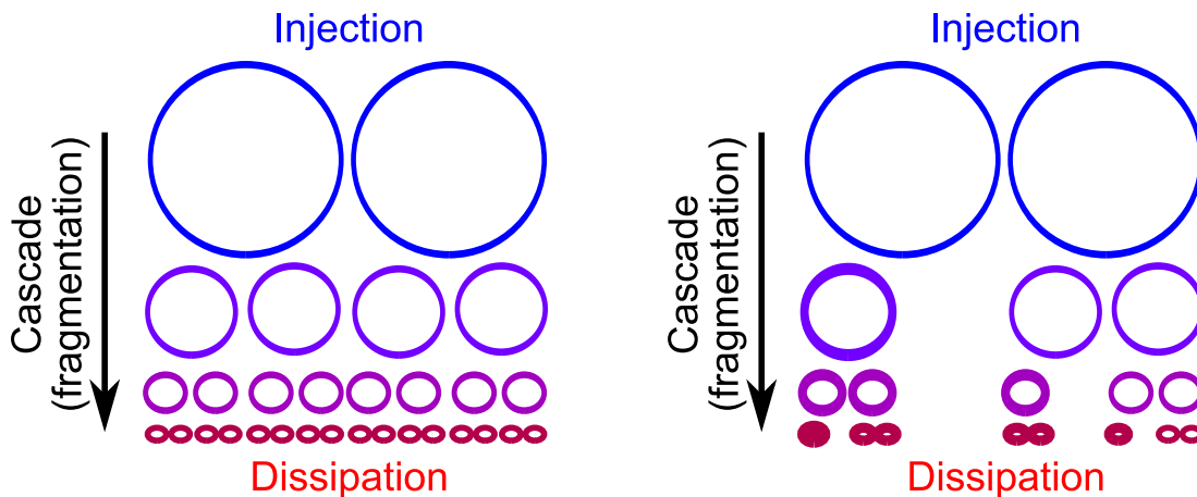
FIGURE 1.4. – Cascade de Richardson : les grands tourbillons se fragmentent en tourbillons de plus en plus petits, jusqu’aux échelles de dissipation. À gauche : cas non-intermittent ; à droite : cas intermittent.
