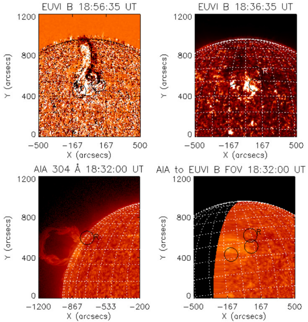
FIGURE 5.3. – En haut : différence d’images successives et image de l’éruption observée par EUVI dans la bande à 30.4nm. En bas : l’image correspondante vue par AIA, et sa reprojexion sur une sphère solaire vue de la position de STEREO B. Les cercles indiquent la position des pieds de la protubérance telle que vue par STEREO B, et la position d’une structure prise comme référence (R). Adapté de la Fig. 4 de Koleva et al. (2012) .
