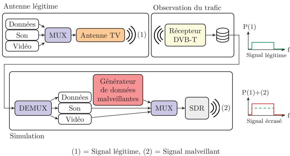
FIGURE 4.1 – Plateforme d'expérimentations DVB
