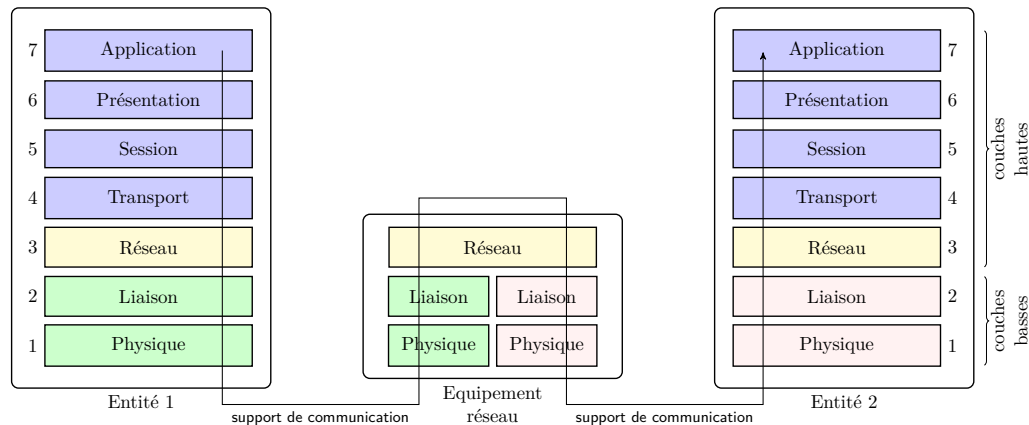
FIGURE 5.2 – Modèle OSI
