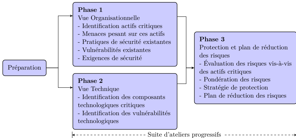
FIGURE 2.8 – Méthode OCTAVE
