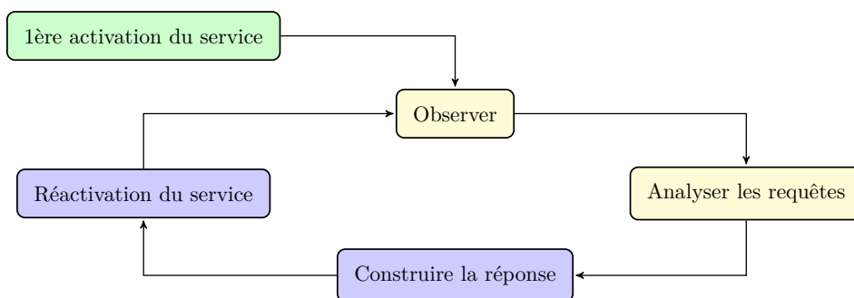
FIGURE 2.10 – Méthode itérative
