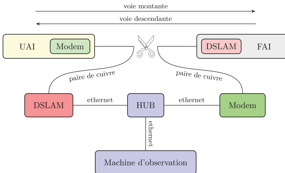
FIGURE 3.2 – Plateforme d'observation d'une boucle locale ADSL
