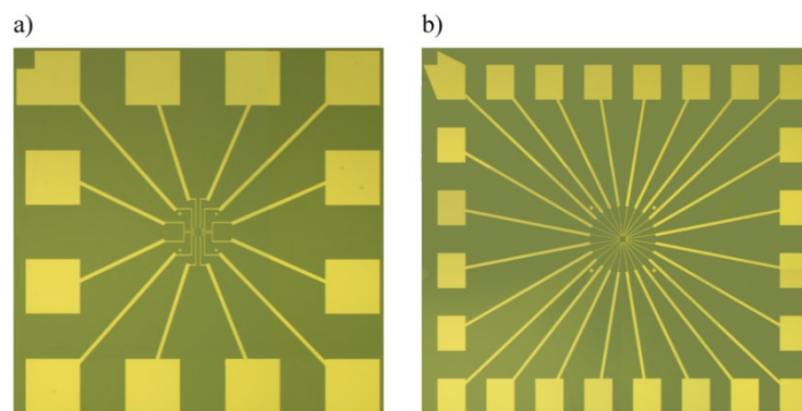
Figure 2-22: Image optique des électrodes macroscopiques utilisées. a),b) La zone de 100x100 μm 2 où a lieu la lithographie électronique pour la fabrication des memristors se situe au centre du motif (exemples à 12 ou 24 électrodes). La taille totale d'un échantillon étant de 5 mm.
