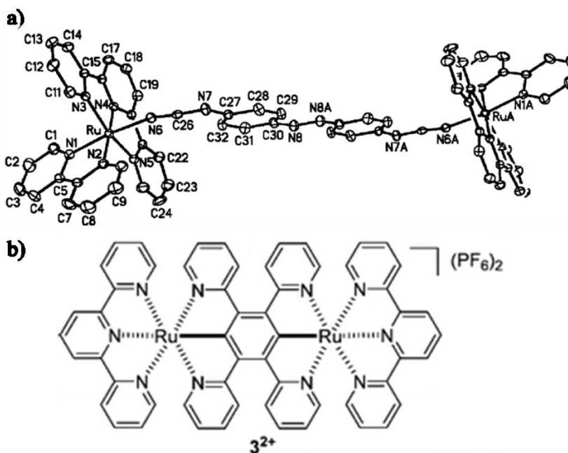
Figure 4-8 : Schéma d'un complexe [\{Ru(trpy)(bpy)\}_2(\mu-adpc)][PF_6]_2 . Figure issue de 22 . Exemple d'un complexe de 1,2,4,5-tetra(2-pyridyl)benzene. Figure issue de 24 .
