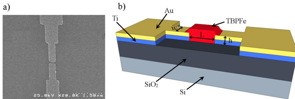
Figure 2-23: a) Image MEB d'une structure horizontale avant greffage b) Schéma de principe d'une structure horizontale. Le rouge correspond à la TBPFe, le jaune à l'Or et le bleu au Ti. En pratique, les électrodes sont également entièrement recouvertes d'un film fin greffé non représenté par souci de clarté.
