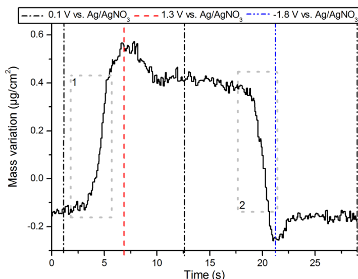
Figure 2-11 : Masse échangée au cours d'un balayage des potentiels pour un film de TBPF e électrogreffé sur un quartz en carbone. Milieu d'analyse : 0,1 M de TBAPF 6 / acétonitrile, V = 200 mV.s -1 ).
