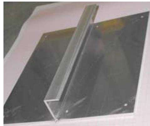
Figure 122 : Pièce de structure de fuselage (en matériau métallique) et éprouvette représentative.
