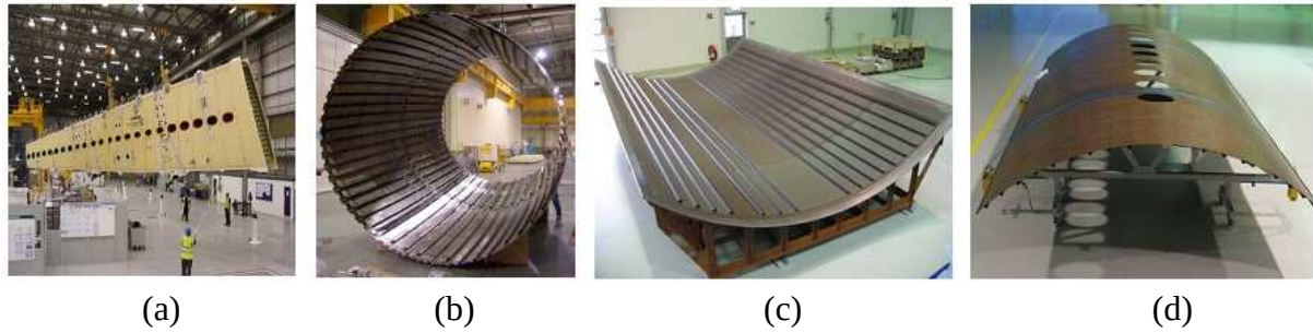
Figure 2 : Structures primaires (aile et section de fuselage désassemblé) de l'Airbus A380 en matériaux composites CFRPs [2].
