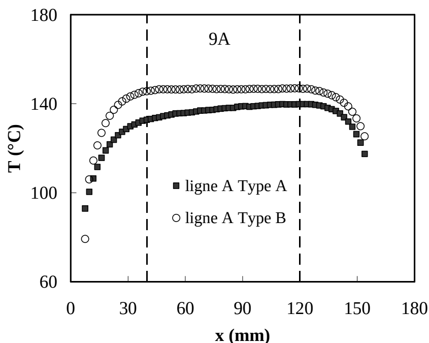
Figure 56 : Profil de température le long de la ligne A, à 9A, pour des éprouvettes croisées [0/90]_4 de Type A et de Type B.
