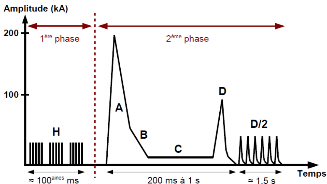
Figure 130 : Schématisation des courants électriques transitoires associés à un impact de foudre (Baldacim et al. [104]).
