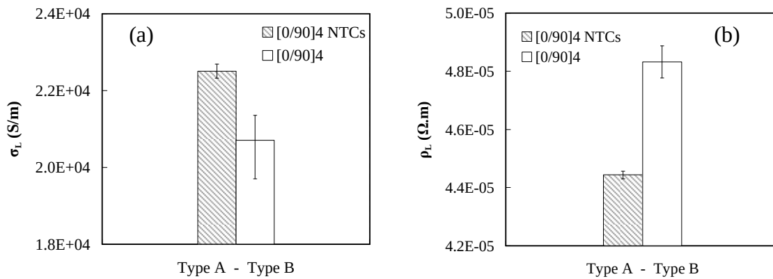
Figure 47 : (a) Conductivité et (b) résistivité électrique équivalente longitudinale d'éprouvettes UD [0/90] 4 de Type A et de Type B.
