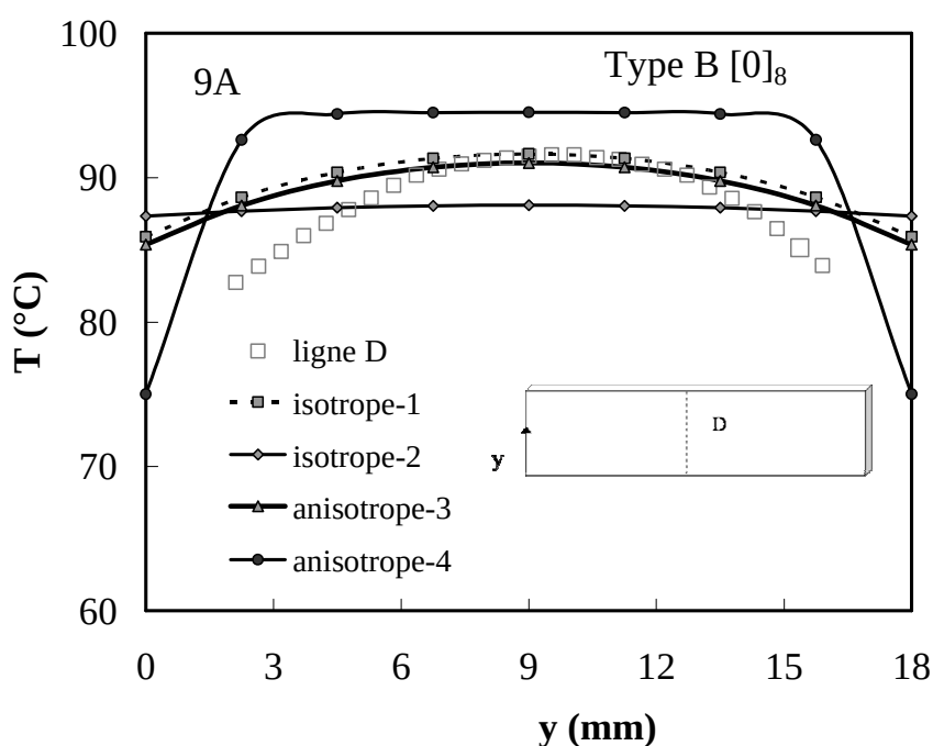
Figure 119 : Profils de température sur la surface d'une éprouvette de Type B unidirectionnelle [0]_8 : comparaison entre les mesures expérimentales (ligne E) et simulations numériques ABAQUS (ligne E) prenant en compte un flux de chaleur sortant des extrémités de l'éprouvette ( I = 9A ), pour différentes valeurs et différents niveaux d'anisotropie du tenseur de conductivité thermique, \lambda .
