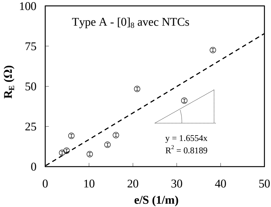
Figure 81 : Résistance électrique dans le sens de l'épaisseur, R_E , en fonction de du facteur de forme de l'éprouvette, e/S , pour un échantillon [0]_8 de Type A.
