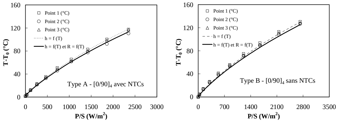
Figure 105 : Température moyenne d'éprouvettes croisées [0/90]_4 (a) de Type A et (b) de Type B en fonction de la puissance électrique dissipée divisée par la section de passage du courant : données expérimentales et simulations numériques issues du modèle thermoélectrique (deux courbes simulées : h dépendant avec la température, h et R_L dépendantes de la température).
