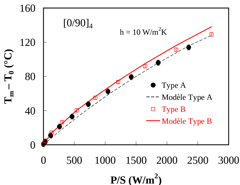
Figure 102 : Température moyenne d'éprouvettes croisées [0/90] 4 de Type A et de Type B en fonction de la puissance électrique dissipée divisée par la section de passage du courant : données expérimentales et simulations numériques issues du modèle thermoélectrique ( h = 10 \text{ W/m}^2\text{K} pour les deux échantillons).
