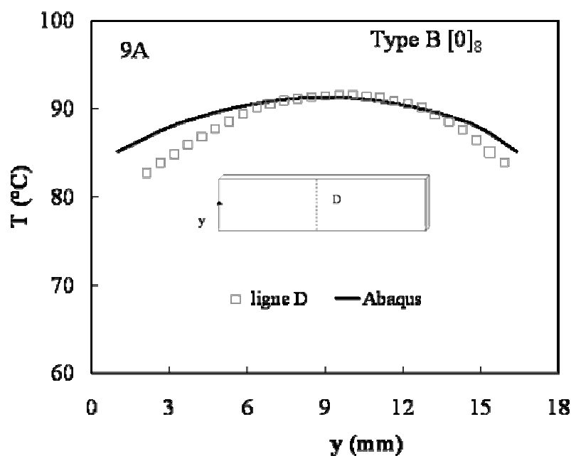
Figure 117 : Profils de température sur la surface d'une éprouvette de Type B unidirectionnelle [0]_8 : comparaison entre les mesures expérimentales (lignes A, B, C) et simulations numériques ABAQUS (ligne A) prenant en compte un flux de chaleur sortant des extrémités de l'éprouvette (a) pour différentes valeurs du courant injecté (b) comparaison à 9A.
