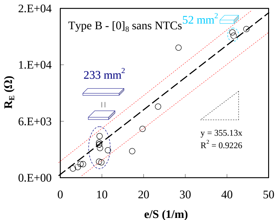
Figure 85 : Résistance électrique dans le sens de l'épaisseur, R_E , en fonction de du facteur de forme de l'éprouvette, e/S , pour un échantillon [0]_8 de Type B. Etude de la dispersion des mesures.
