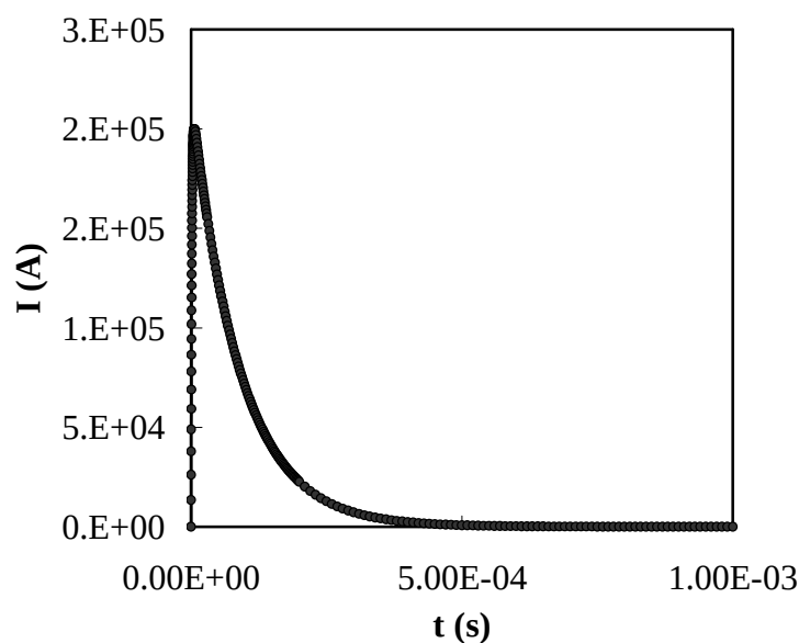
Figure 131 : Courant électrique associé à un impact de foudre (« deuxième phase » du chargement électrique) en fonction du temps selon Baldacim et al. ([105])
