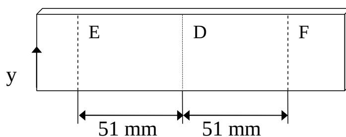
Figure 57 : Illustration schématisée des trois lignes E, D et F verticales situées sur la surface des éprouvettes et choisies pour visualiser les profils de la température.
