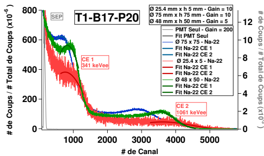
Figure 2.31 – Spectres en énergie mesurés au CEA du scintillateur T1-B17-P20 à 3 dimensions après irradiation gamma.
