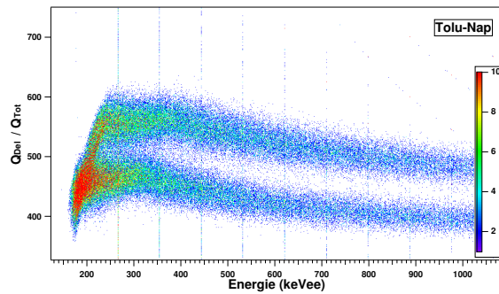
Figure 4.40 – Spectre de discrimination n/\gamma du liquide du laboratoire Tolu-Nap ( ^{241}\text{AmBe} ).
