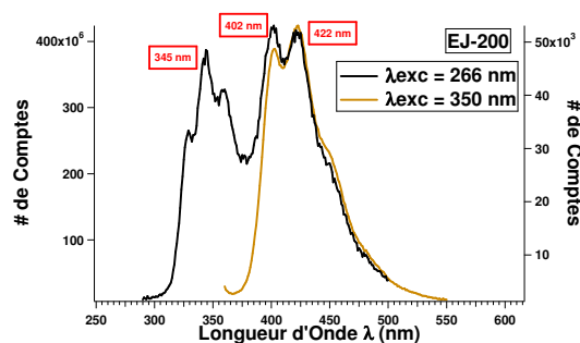
Figure 2.9 – Spectre d'émission de l'EJ-200 pour des excitations fixées à 266 nm et 350 nm.
