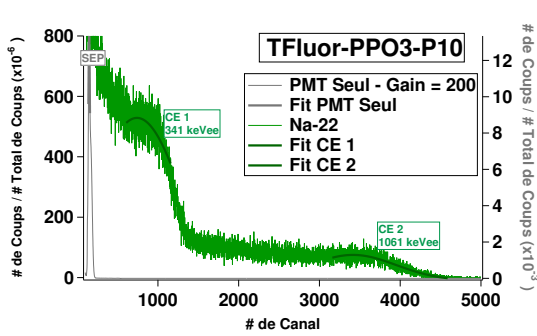
Figure 2.35 – Spectre en énergie mesuré au CEA du scintillateur TFluor-PPO3-P10.
