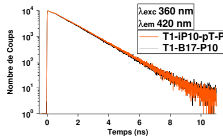
Figure 2.22 – Mesure de photon unique pour la détermination de la durée de vie du scintillateur synthétisé sur la base des travaux de Brooks avec un constitué de biphenyle à 17 wt% et du POPOP à 0,1 wt%. Leur épaisseur est de 5 mm.
