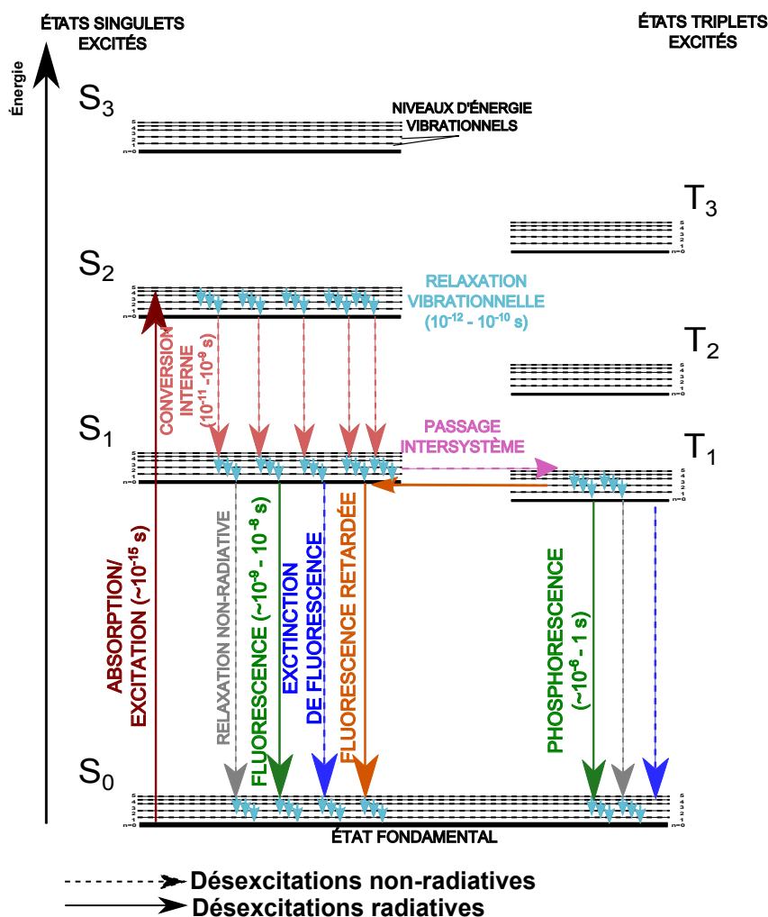
Figure 1.2 – Diagramme de Perrin-Jablonski décrivant les différentes transitions possibles dans un fluorophore après excitation. Ces transitions se divisent entre le type radiatif : fluorescence (10 -9 - 10 -6 s) ou phosphorescence (10 -6 s à plus de quelques dizaines de secondes); et non-radiatif : relaxations vibrationnelles (faibles variations d'énergie), conversion interne depuis des états d'énergie plus élevée, relaxation non-radiative pouvant correspondre à une extinction de fluorescence et pour finir le passage intersystème qui peut donner lieu à une composante de fluorescence retardée si une énergie suffisante est apportée au système.
