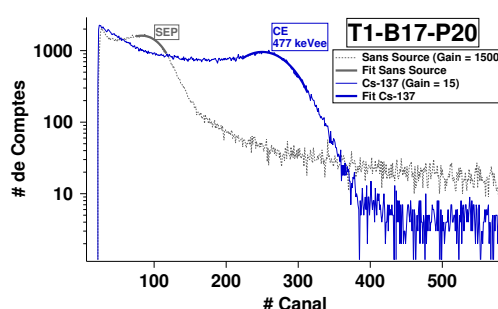
Figure 2.28 – Spectres en énergie mesurés au NCBJ du scintillateur T1-B17-P20 \varnothing 48 mm \times h 50 mm.
