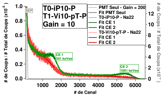
Figure 2.33 – Spectres en énergie mesurés au CEA des scintillateurs T0-iP10-P et T1-Vi10-pT-P après irradiation gamma.
