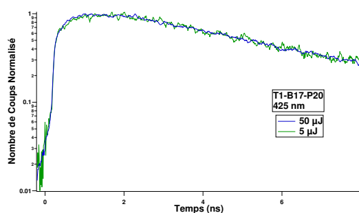
Figure 5.24 – Déclins de luminescence à 5 et 50 \mu\text{J} sur 10 \text{ ns} du plastique T1-B17-P20 à 425 \text{ nm} .
