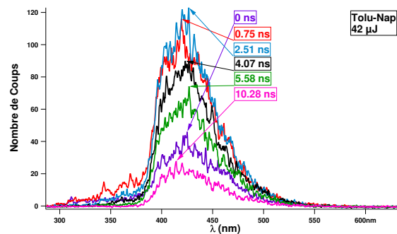
Figure 5.45 – Spectres obtenus par l'illumination à 42 \mu\text{J} sur 50 ns du liquide 1,8-naphtalimide dans le toluène (Tolu-Nap) à différents instants.
