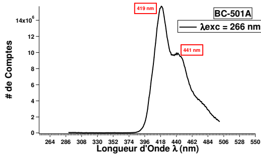
Figure 2.8 – Spectre d'émission du BC-501A pour une excitation fixée à 266 nm.
