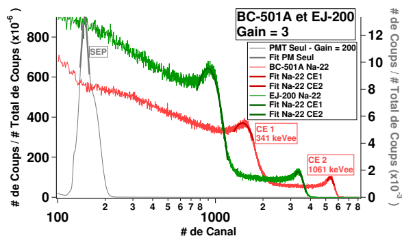
Figure 2.25 – Spectres en énergie des scintillateurs BC-501A ( \varnothing 50\text{ mm} \times h 50\text{ mm} ) et EJ-200 ( \varnothing 30\text{ mm} \times h 30\text{ mm} ) au CEA après irradiation gamma.
