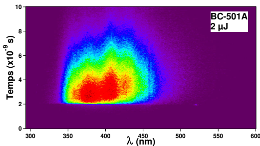
Figure 5.12 – Image enregistrée avec la streak caméra du liquide BC-501A à 2 \mu\text{J} sur 10 ns.
