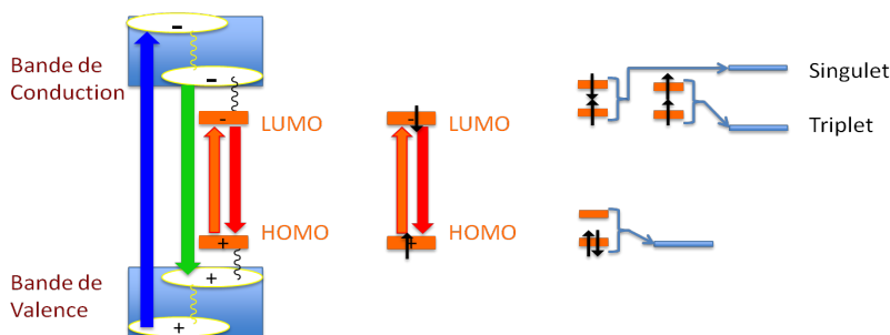
Figure 1.4 – Schéma général des processus communs de désexcitation radiative des matériaux luminescents.
