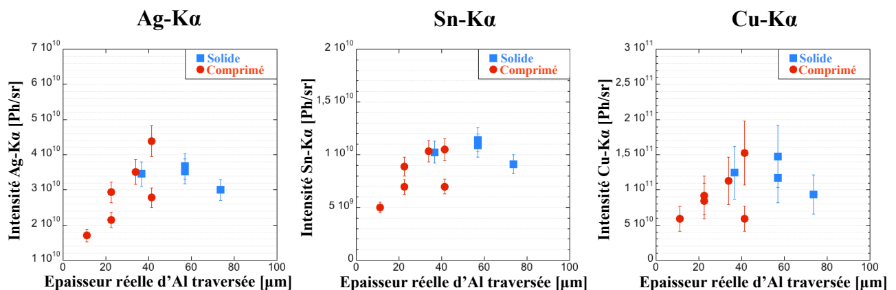
Figure 6.4: Evolution des émissions absolues des traceurs d'argent (gauche), d'étain (milieu) et de cuivre (droite) pour les cibles solides (carrés) et comprimées (disques) en fonction de l'épaisseur réelle d'aluminium traversée. Ces valeurs sont corrigées de la transmission des différents matériaux.
