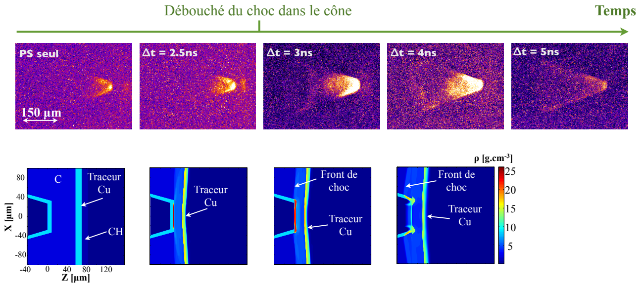
Figure 6.12: Résultats expérimentaux (haut) obtenus en imageant l'émission \text{Cu-K}\alpha de la cible. Le retard entre les deux faisceaux laser augmente en se déplaçant vers la droite. Ces images sont comparées à des résultats de simulations hydrodynamiques 2D (bas).
