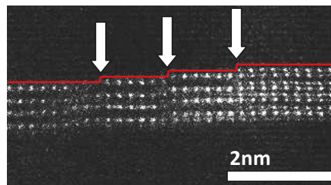
Figure 13: image HAADF-STEM en axe de zone <112> d'un précipité T 1 épais cisailé sur un échantillon vieilli 18h à 155°C et 70h à 190°C et déformé plastiquement 2%.
