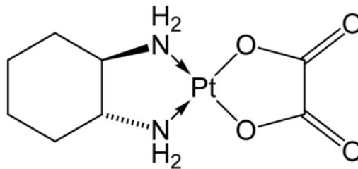
Figure 6 : structure de la molécule d'oxaliplatine.
