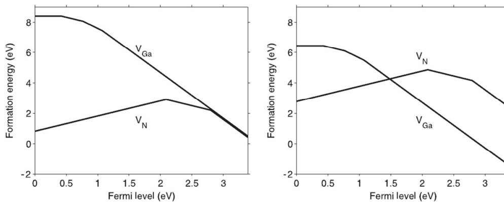
Figure IV-52 : Energie de formation des lacunes d'azote V_N et de gallium V_{\text{Ga}} dans du GaN riche en gallium (gauche) et riche en azote (droite) en fonction de la position du niveau de Fermi par rapport au maximum de la bande de valence [245]
