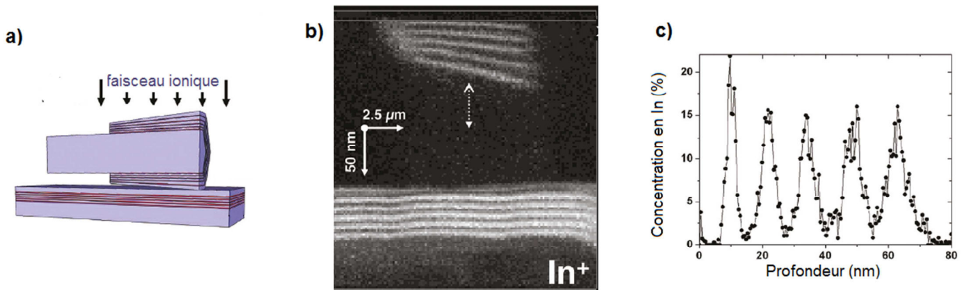
Figure I-21 : a) Schéma d'une analyse ToF SIMS sur un fil dispersé de \text{InGaN}/\text{GaN} à puits quantiques multiples. b) Cartographie de la concentration en ions \text{In}^+ extraits du fil et du substrat. Uniquement La partie supérieure du fil est analysé en raison des temps d'abrasion trop long. c) Estimation de la concentration en indium en fonction de la profondeur au niveau des puits quantiques.
