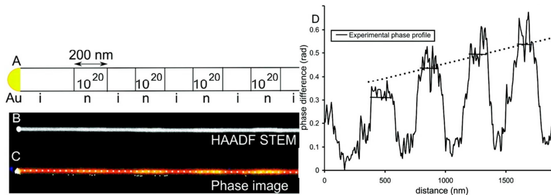
Figure I-28 : a) Représentation schématique d'un nanofil dopé n b) image STEM, c) image de phase, d) profil de phase. [122]
