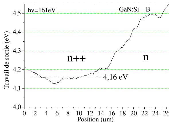
Figure IV-43 : Profil de travail de sortie du fil B sous illumination synchrotron à h\nu=161 eV.
