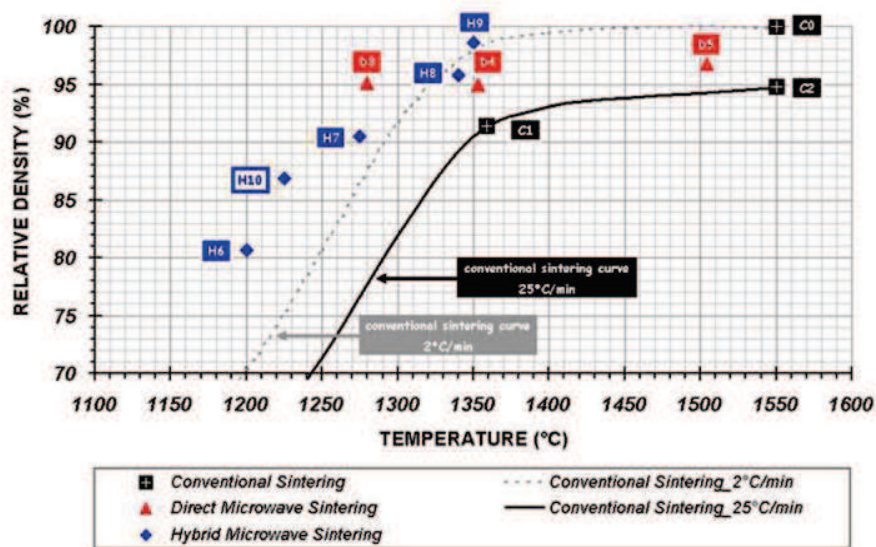
Figure A.II.29 : Variations de la densité relative en fonction de la température maximale de frittage pour différents modes de chauffage : C conventionnel, D et H micro-ondes direct et hybride [CHA10].
