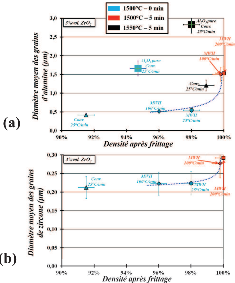
Figure C.II.29 : Variations de la taille moyenne des grains d'alumine (a) et de zircon (b) en fonction de la densité relative finale des échantillons d'alumine-zircon à 3%vol. Y-ZrO 2 frittés conventionnellement (Conv.) et par micro-ondes hybride (MO) dans différentes conditions (vitesses de chauffage, palier en température...).
