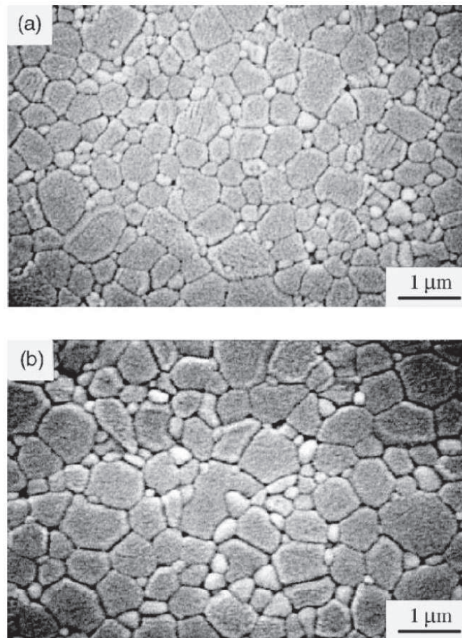
Figure A.II.18 : Photographies MEB de coupes transversales d'échantillons d'alumine (200 nm)-15%mol.ZrO 2 (10 nm), frittés à : (a) 1425°C, (b) 1475°C [RAO03].
