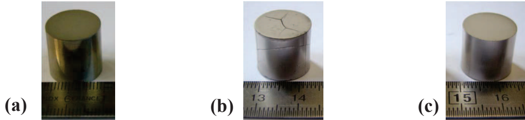
Figure B.I.11 : Comprimés de nickel : (a) à cru, (b) après frittage induction sans déliantage préalable et (c) après frittage induction avec déliantage (fréquence de 150 kHz).
