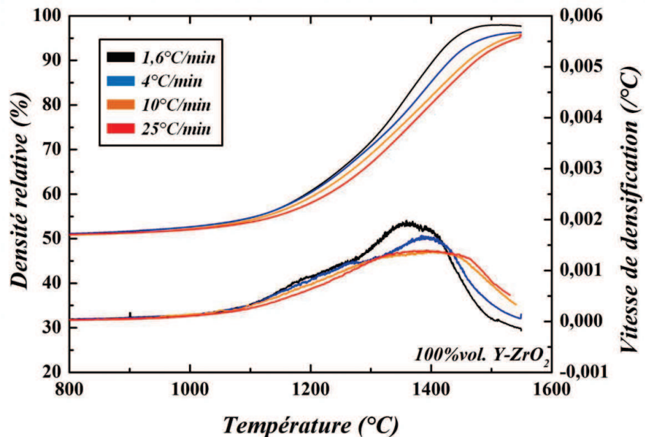
Figure C.I.2 : Variations de la densité relative et de la vitesse de densification en fonction de la température de frittage pour différentes vitesses de chauffage ( 1,6 , 4 , 10 et 25^{\circ}\text{C}/\text{min} ) dans le cas de la poudre de zircone yttrée seule ( 100\% vol. \text{Y-ZrO}_2 ).
