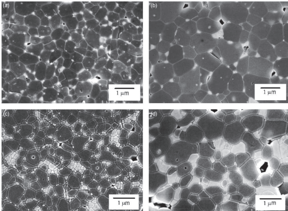
Figure A.II.20 : Evolution microstructurale de composites Al_2O_3 - ZrO_2 contenant 5 et 30%vol. ZrO_2 : (a) 5%vol. ZrO_2 , à 1600^\circ C sans palier, (b) 5%vol. ZrO_2 , 1600^\circ C avec un palier de 30h, (c) 30%vol. ZrO_2 , 1600^\circ C sans palier, et (d) 30%vol. ZrO_2 , 1600^\circ C avec un palier de 30h [CAS05].
