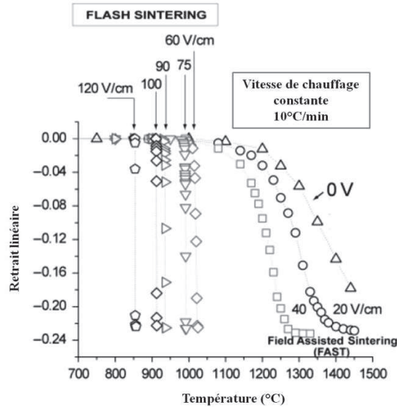
Figure A.3 : Influence des paramètres opératoires sur l'évolution du retrait linéaire en fonction de la température lors d'un frittage flash de zircone quadratique [COL10].
