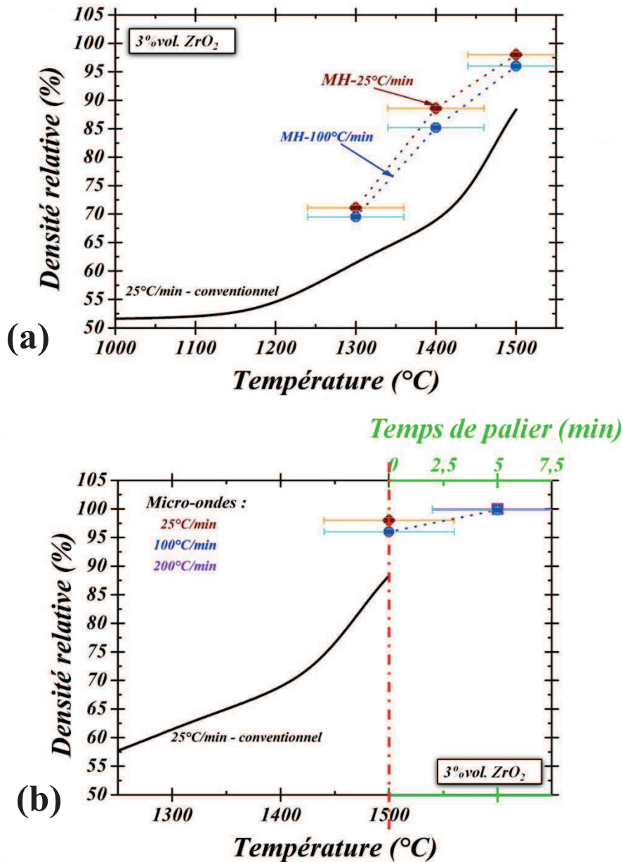
Figure C.II.12 : Densité finale des composites alumine-zircone à 3%vol. Y-ZrO 2 en fonction de la température maximale de frittage en conventionnel (25°C/min) et en micro-ondes hybride (MWH – 25, 100 et 200°C/min – pyromètre IR) : (a) effet de la vitesse de chauffage ; (b) effet du palier en température.
