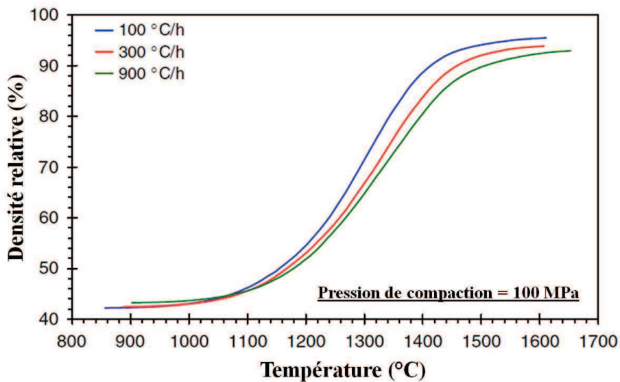
Figure A.II.3 : Courbes de densification de comprimés à cru de zircone yttrée à 3%mol. Y_2O_3 (60 nm, densité à cru 42-43%) obtenues pour différentes vitesses de chauffage : 1, 7, 5 et 15°C/min [BER07b].
