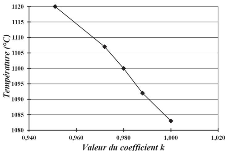
Figure B.II.14 : Effet de la valeur du coefficient sur la valeur de la température mesurée (température du four et donc de l'échantillon composite à 3%vol. Y-ZrO 2 = 1100°C).
