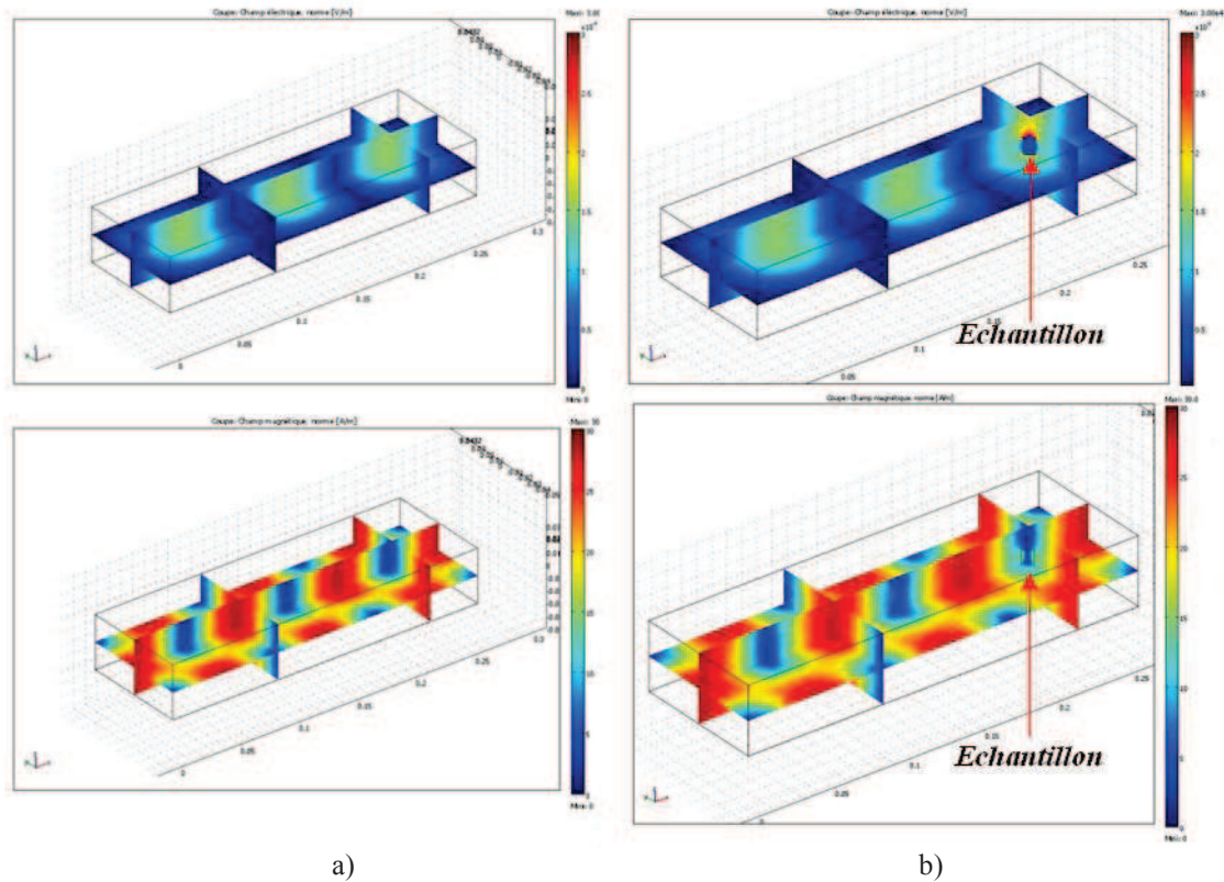
Figure a.8 : Distribution des champs électromagnétiques dans la cavité : (a) cavité vide ; (b) avec un échantillon (avec une permittivité relative de 10) dans la cavité [BOU10].
