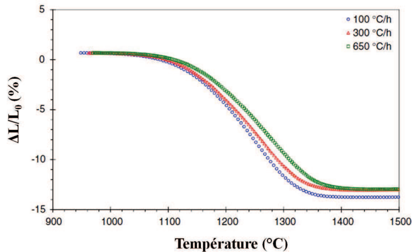
Figure A.II.1 : Courbes de retrait linéaire obtenues pour différentes vitesses de chauffage (1.7, 5 et 11°C/min) dans le cas de comprimés d'alumine \alpha ultrapure (110 nm, densité à cru : 63%) [BER07a]
