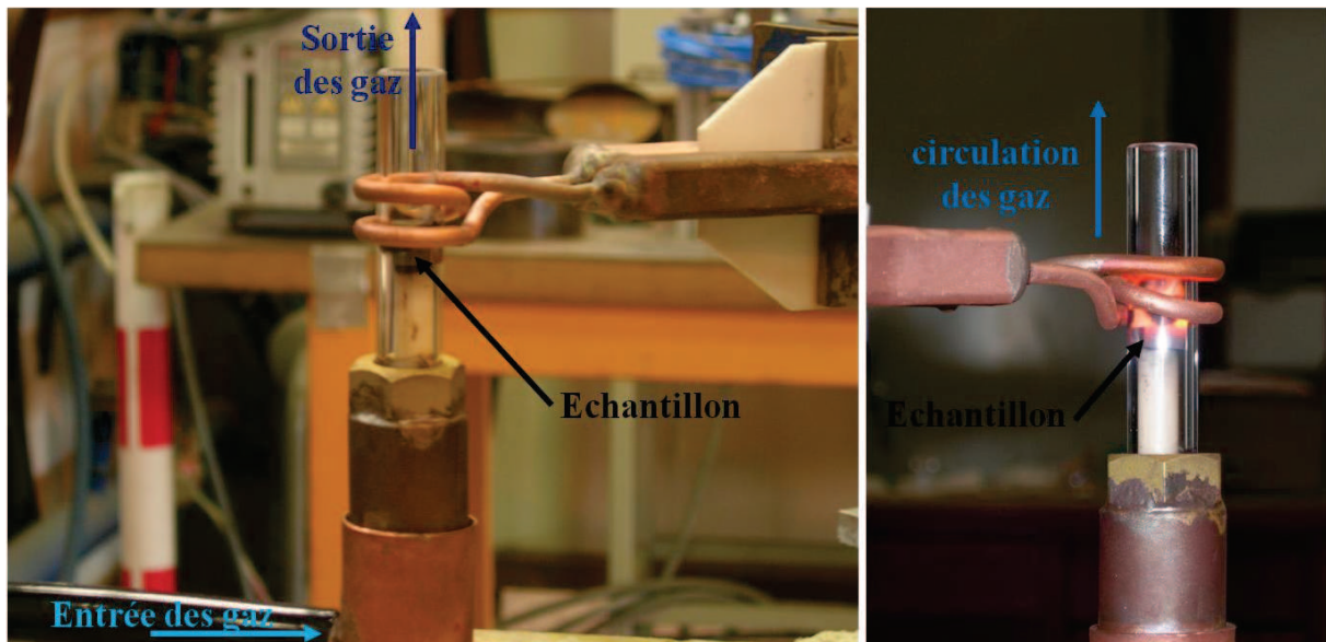
Figure D.I.1 : Installation utilisée pour réaliser les premiers essais « exploratoires » au printemps 2008.
