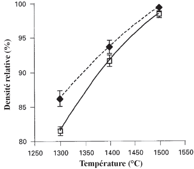
Figure A.II.30 : Evolution de la densité relative en fonction de la température de frittage pour une poudre de zircone yttrée (3%mol. Y_2O_3 ) lors d'un chauffage à 2^\circ C/min : (□) chauffage conventionnel, (◇) chauffage micro-ondes [NIG96].
