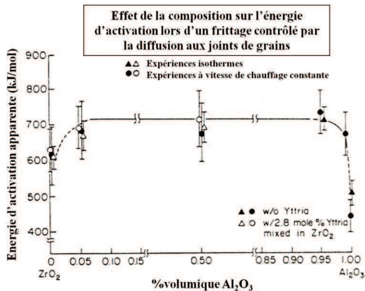
Figure A.II.14 : Variations de l'énergie d'activation apparente pour le frittage du système Al 2 O 3 /ZrO 2 en fonction de la teneur en ZrO 2 dans l'alumine [WAN91].
