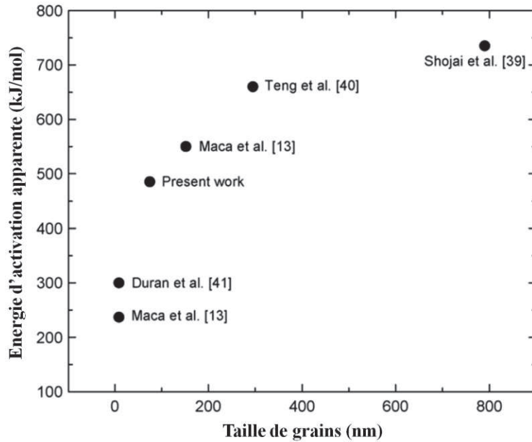
Figure A.II.5 : Effet de la taille des particules élémentaires d'une poudre de zircone yttrée à 3%mol. Y_2O_3 (Y-TZP : Ytria Tetragonal Zirconia Polycrystal) sur l'énergie d'activation apparente pour le frittage [MAZ09].
