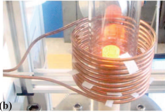
Figure D.I.6 : Bobines utilisées pour les expériences de frittage par induction : (a) 150 kHz et (b) 50 kHz.
