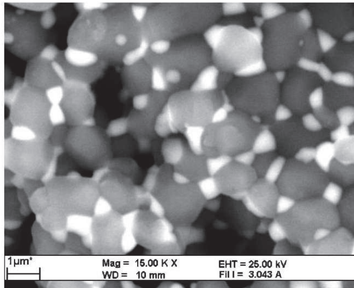
Figure A.II.21 : Image MEB en électrons rétrodiffusés d'une coupe transversale, polie et attaquée, d'un échantillon fritté à 1450^\circ C pendant 30 min. [BIA06].
