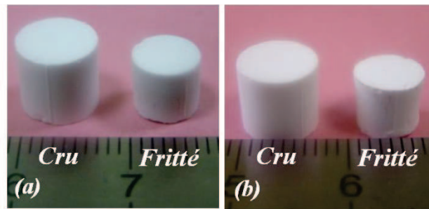
Figure C.II.8 : Comprimés d'alumine-zircone à 3%vol. Y-ZrO_2 , avant et après frittage micro-ondes direct jusqu'à 1500°C à deux vitesses de chauffage : (a) 25°C/min ; (b) 100°C/min.
