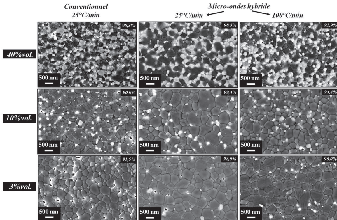
Figure C.II.25 : Effet de la vitesse de chauffage (25 et 100°C/min) et du procédé de chauffage (conventionnel et micro-ondes hybride) sur la microstructure pour les trois composites alumine-zircon à 40, 10 et 3%vol. Y-ZrO 2 (1500°C sans palier).
