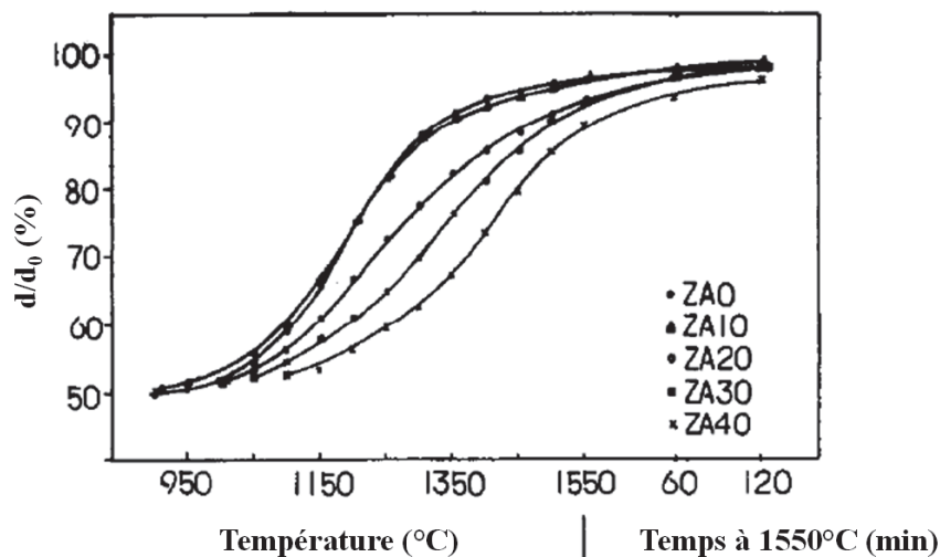
Figure A.II.6 : Courbes de densification de comprimés de zircone/alumine (ZA0 sans alumine, ZA10 10%vol. d'alumine, ZA40 40%vol. d'alumine) lors d'un frittage à vitesse de chauffage constante de 10^\circ\text{C}/\text{min} jusqu'à 1550^\circ\text{C} suivi d'un maintien à 1550^\circ\text{C} pendant 2 h [SHI95].
