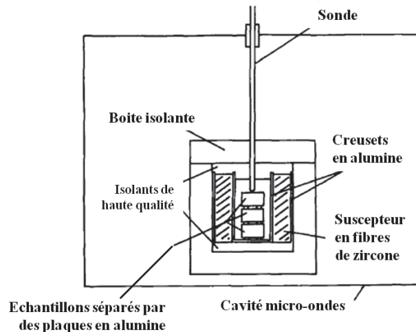
Figure A.II.38 : Représentation de l'installation de frittage micro-ondes indirect (avec suscepteur) dans une cavité multimodes à 2,45 GHz [SAM92].
