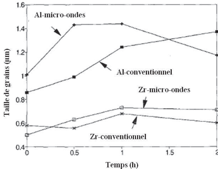
Figure A.II.40 : Variations de la taille de grains avec le temps de palier à la température de frittage (1500°C) dans le système Al_2O_3 -20% m. ZrO_2 lors d'un chauffage conventionnel ou par micro-ondes [SAM92].
