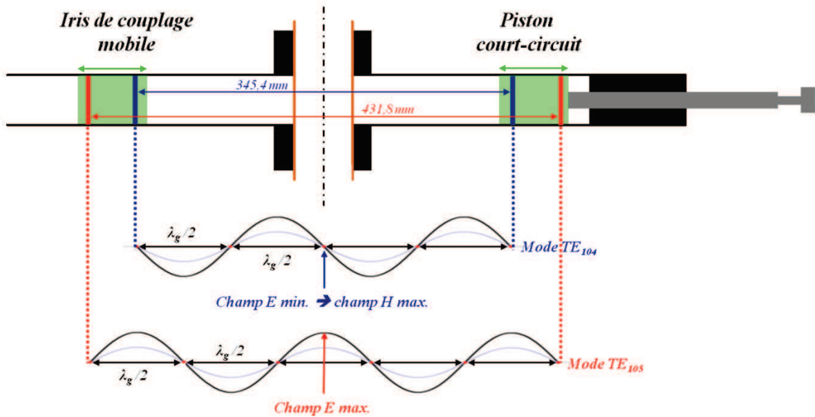
Figure a.7 : Cavité et champ électrique de l'onde stationnaire à la résonance pour les modes TE_{104} (champ magnétique maximum au centre de la cavité) et TE_{105} (champ électrique maximum au centre).
