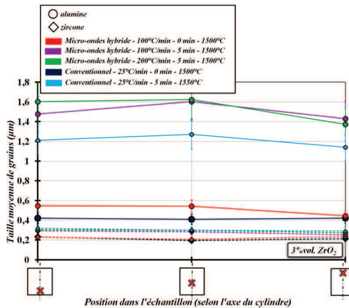
Figure C.II.24 : Mesures de la taille de grains dans les échantillons d'alumine-zircone à 3%vol. Y-ZrO 2 frittés conventionnellement et par micro-ondes hybride dans différentes conditions (mesure de la température avec un pyromètre IR).
