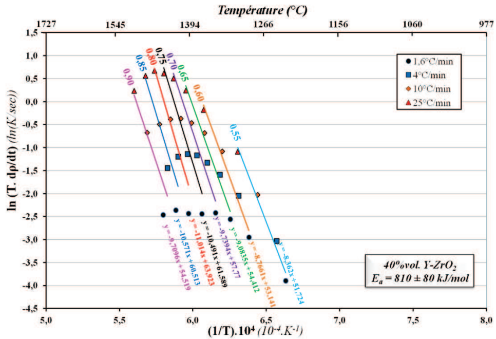
Figure a.12 : Diagramme d'Arrhenius obtenu pour le mélange Al_2O_3 - ZrO_2 à 40%vol. Y-ZrO_2 lors d'essais de frittage à vitesses de chauffage constantes.
