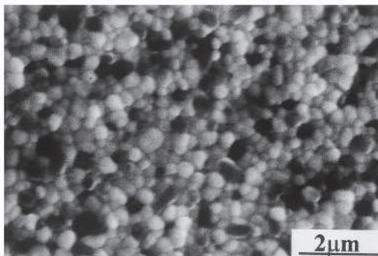
Figure A.II.42 : Micrographie MEB montrant une microstructure représentative d'un échantillon de Y-ZrO_2 - 20\%m. Al_2O_3 fritté par micro-ondes à 1500^\circ C (attaque thermique pour révéler la microstructure - Grains d' Al_2O_3 en noir) [TRA00].
