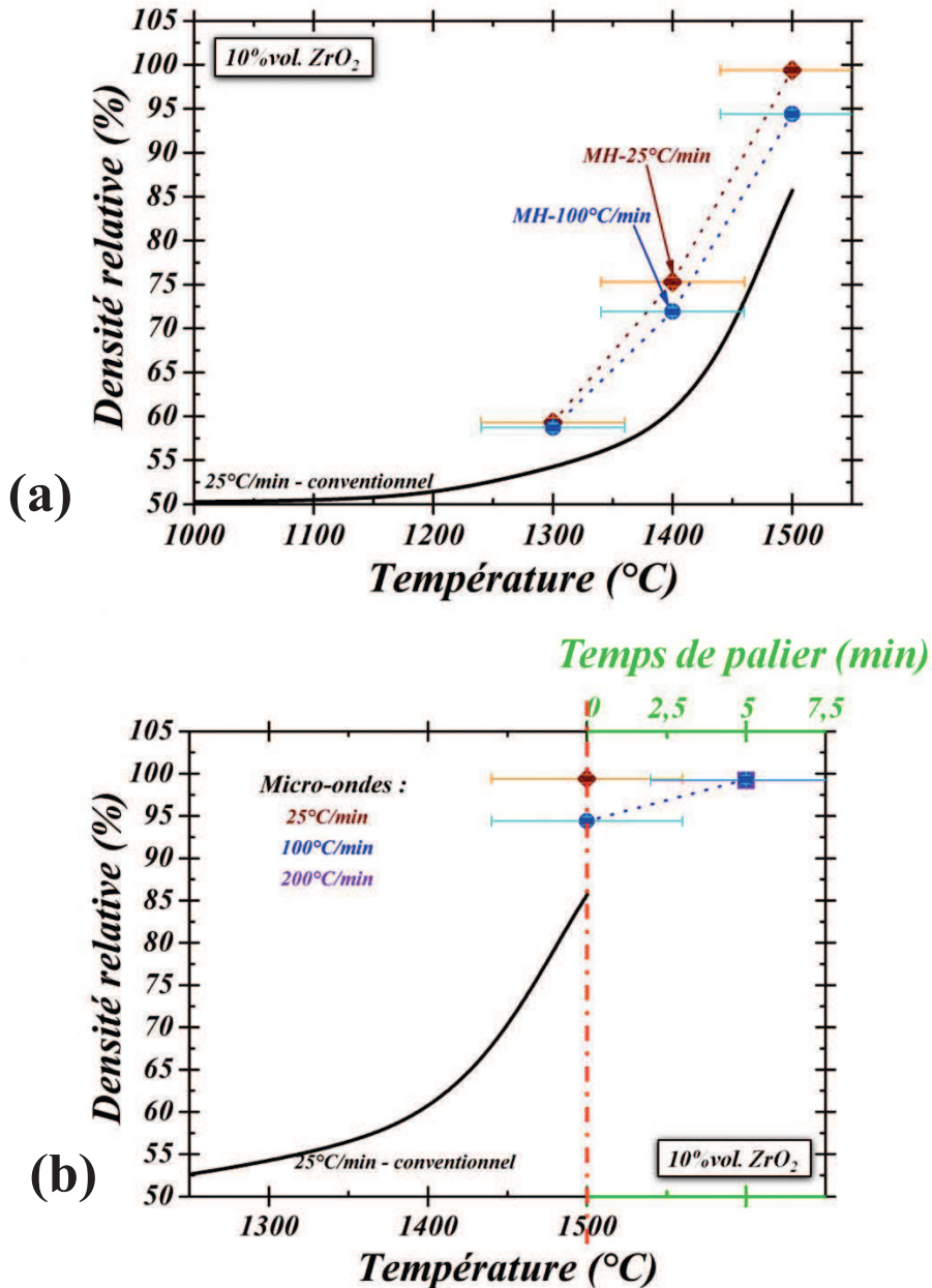
Figure C.II.11 : Densité finale des composites alumine-zircone à 10%vol. Y-ZrO 2 en fonction de la température maximale pour le frittage conventionnel (25°C/min) et par micro-ondes hybride (MWH – 25, 100 et 200°C/min – pyromètre IR) : (a) effet de la vitesse de chauffage ; (b) effet du palier en température.
