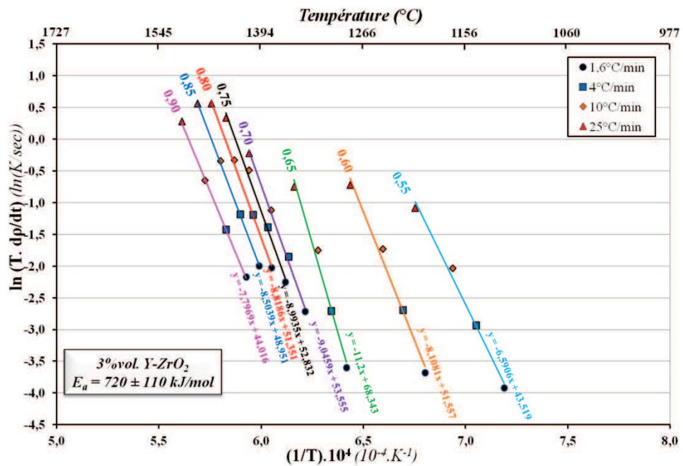
Figure a.13 : Diagramme d'Arrhenius obtenu pour le mélange Al_2O_3 - ZrO_2 à 3%vol. Y-ZrO_2 lors d'essais de frittage à vitesses de chauffage constantes.
