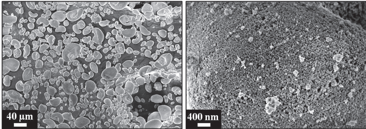
Figure B.I.2 : Poudre de zirconie yttrée à 3%mol. Y_2O_3 (BZ-3Y - lot n°16129 – Baikowski Fr.).
