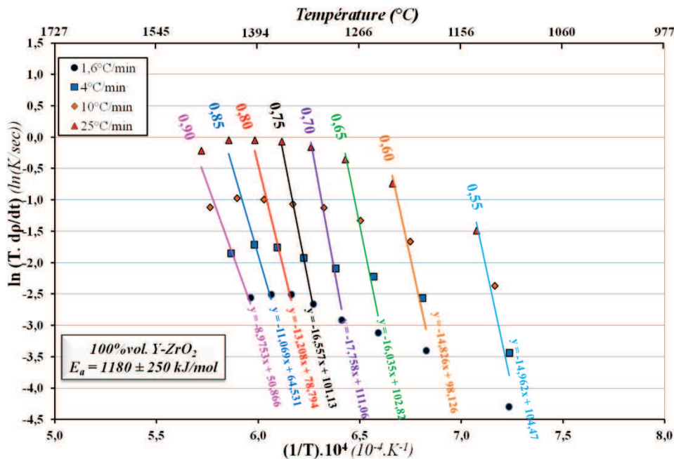
Figure a.11 : Diagramme d'Arrhenius obtenu pour la poudre de zircon pure (30 nm) lors d'essais de frittage à vitesses de chauffage constantes.
