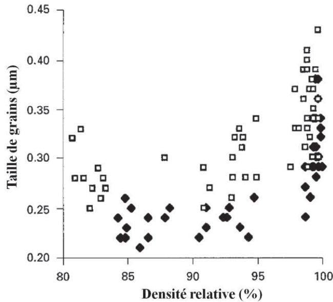
Figure A.II.31 : Variations de la taille de grains en fonction de la densité relative lors du frittage à 2^\circ C/min d'une poudre de zircone yttrée à 3%mol. Y_2O_3 : (□) chauffage conventionnel, (◇) chauffage par micro-ondes [NIG96].
