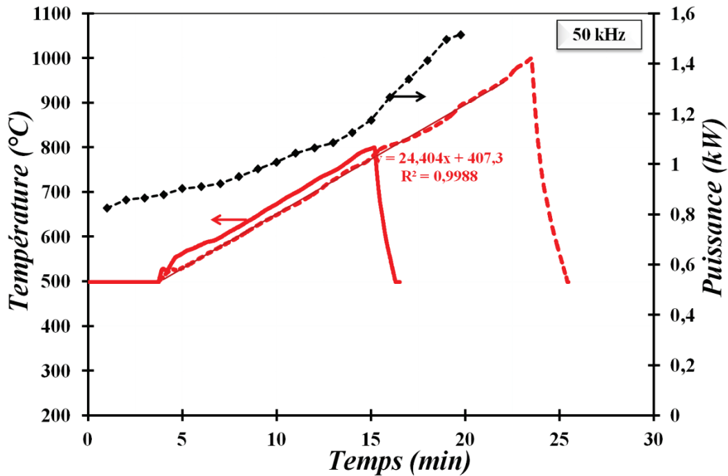
Figure D.III.13 : Ajustement de la puissance du générateur pour contrôler une vitesse de chauffage constante lors d'une expérience de frittage par induction à 50 kHz.
