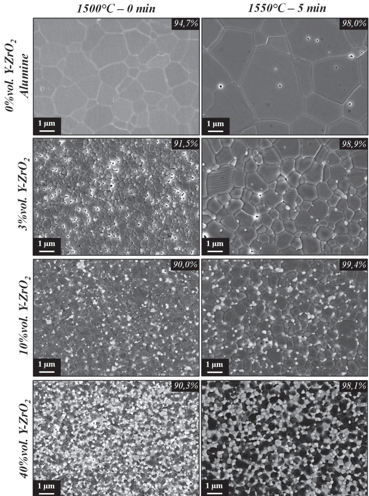
Figure C.I.6 : Micrographies MEB au cœur d'échantillons céramiques (alumine seule (0%vol. Y-ZrO 2 ) et composites alumine-zircone (3, 10 et 40%vol. Y-ZrO 2 )), frittés conventionnellement à une vitesse de chauffage de 25°C/min jusqu'à différentes températures (1500 et 1550°C), selon une coupe transversale polie et attaquée thermiquement.
