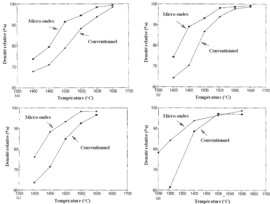
Figure A.II.39 : Variations de la densité relative finale avec la température de frittage lors d'un chauffage conventionnel et par micro-ondes (30°C/min) pour des systèmes Al_2O_3-ZrO_2 dans différentes proportions : (a) Alumine pure, (b) alumine + 20% m. de zirconne, (c) alumine + 50% m. de zirconne, et (d) zirconne pure [SAM92].
