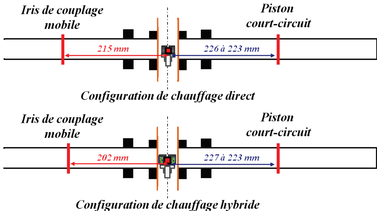
Figure a.9 : Résumé des conditions expérimentales de frittage par micro-ondes (positions de l'iris et du piston court-circuit) en configuration de chauffage direct (a) et hybride (b).
