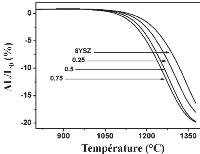
Figure A.II.12 : Courbes de retrait linéaire en fonction de la température lors d'un frittage à 8°C/min jusqu'à 1380°C de la poudre de zircone yttrée à 8%mol. Y_2O_3 avec différentes teneurs en NiO : 0, 0.25, 0.5 et 0.75%mol. [BAT11].
