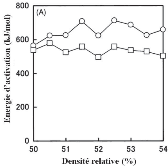
Figure A.II.10 : Energie d'activation apparente pour la densification lors de l'étape initiale du frittage (densité relative entre 50 et 54%). Les ronds (○) et les carrés (□) représentent respectivement la poudre 3YS et 3YSE [MAT05].
