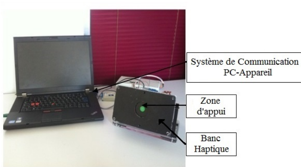
FIGURE 3.1 – Le banc préliminaire utilisé pour produire les signaux vibrotactiles.
