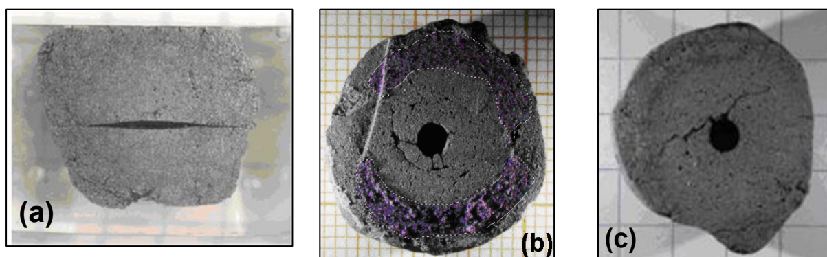
Figure III-9 : Observation au microscope optique des surfaces de collage : (a) Deux moitiés collées d'une boulette coupée au milieu, réduites et enrobées avec une résine type époxy sans être séparées: essai à 1100°C, pendant 1h, sous H 2 pur. (b) Surface de collage, après la séparation : boulette coupée au milieu et réduite à 1100°C, pendant 1h, sous H 2 pur ( F_{\text{collage}} > 50\text{N} ). Traces de collage visibles. (c) Surface de collage, après la séparation : boulette coupée au milieu et réduite à 1000°C, pendant 1h, sous H 2 pur ( F_{\text{collage}} = 0.94\text{ N} ). Traces de collage pas visibles.
