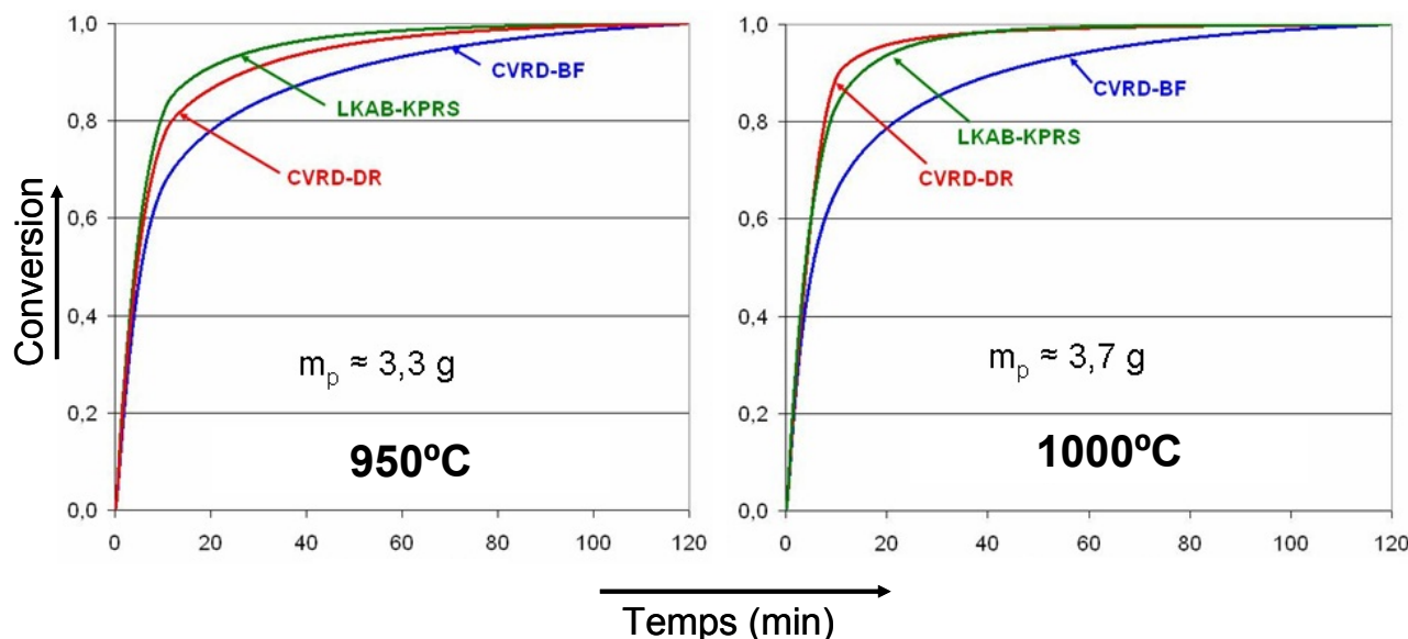
Figure II-5 : Comparaison entre les cinétiques de réduction des boulettes CVRD-BF, CVRD-DR et LKAB-KPRS réduites par \text{H}_2 (2 L/min de débit gazeux \text{H}_2/\text{He} 60/40 % vol.) : à gauche : 950°C ( m_p \approx 3,3 \text{ g} ) et à droite : 1000°C ( m_p \approx 3,7 \text{ g} ).
