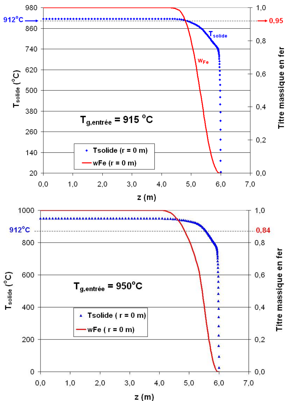
Figure V-14 : Variation du titre massique en fer et de la température du solide en fonction de la position axiale z , au centre de la cuve ( r = 0 m), pour les cas d'un mélange gazeux alimenté à 915^\circ\text{C} et 950^\circ\text{C} . Boulettes du type CVRD-DR ( d_p = 0,014 m, \varepsilon_{\text{ini},b} = 0,33 , a_{\text{sp},b} = 0,0604 m 2 /g). Les autres conditions sont les mêmes que dans le cas de référence.
