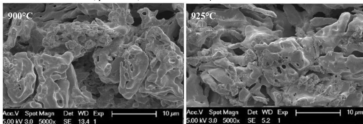
Figure II-26 : Images MEB du fer obtenu par la réduction de boulettes CVRD-DR par H 2 (2 L/min de débit gazeux H 2 /He 60/40 % vol.) (Détecteur SE). Réduction à 900°C ( gauche ) ; Réduction à 925°C ( droite ).
