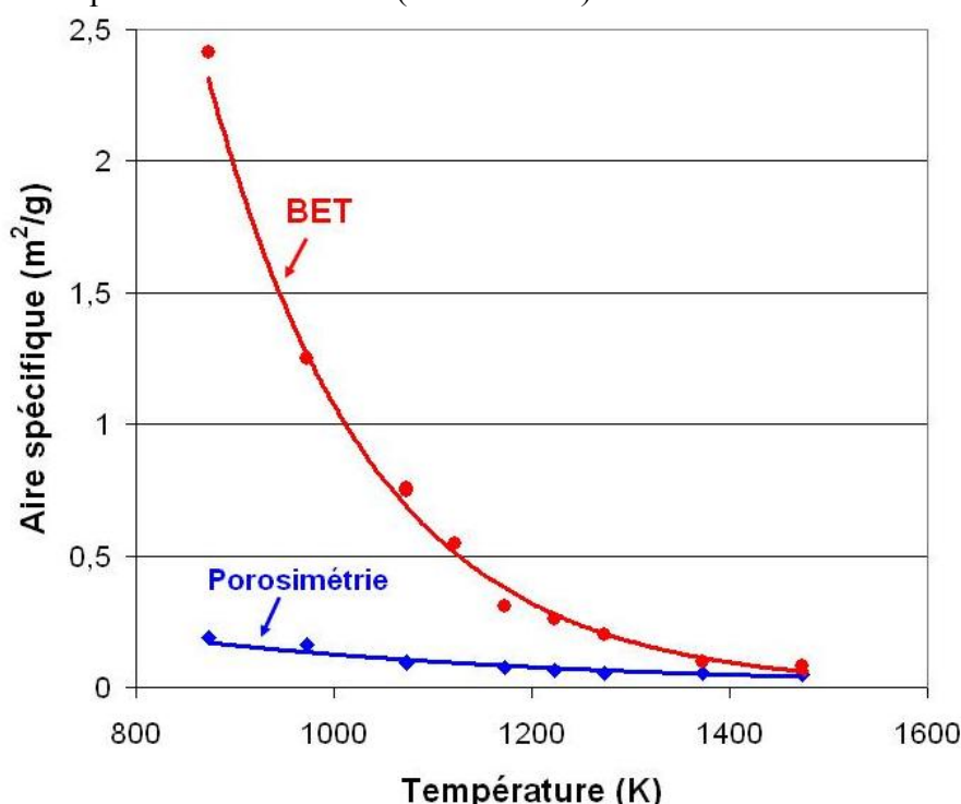
Figure II-46 : Surface spécifique moyenne ( a_{sp} ) du fer final formé par réduction de boulettes à différentes températures (2 L/min de débit gazeux H_2/He 60/40 % vol.) – méthode BET et porosimétrie.
