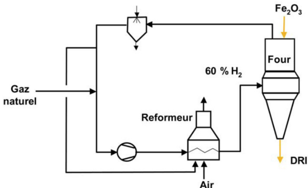
Figure I-1 : Schéma du procédé de réduction directe du four à cuve [3].
