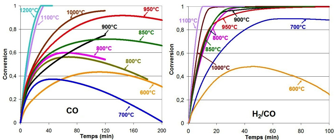
Figure II-36 : Courbes de réduction de boulettes CVRD-DR ( m_p \approx 4.7 g) par CO (gauche) et par le mélange gazeux ULCORED (droite), à différentes températures (2 L/min de débit gazeux Gaz réducteur/He 60/40 % vol.).
