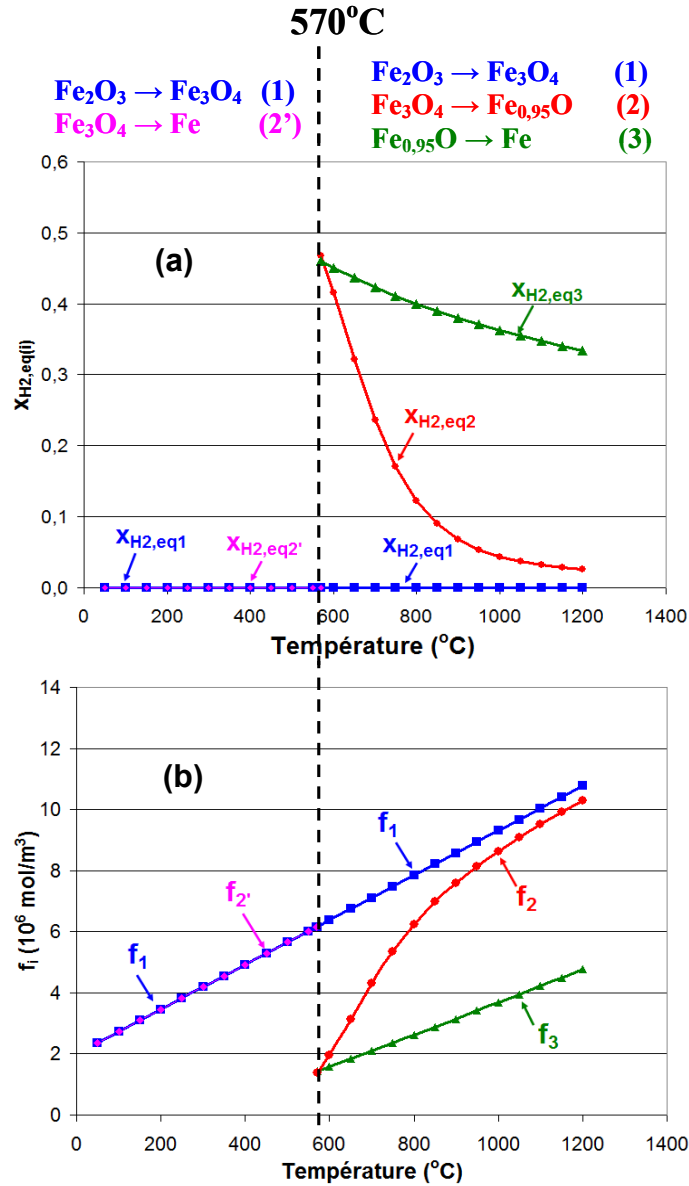
Figure IV-9 : (a) Variations du titre molaire en \text{H}_2 à l'équilibre ( x_{\text{H}_2,eq(i)} ) et (b) des forces motrices f_{(i)} , pour chacune des réactions ( i = 1, 2, 2' et 3). Cas d'un mélange 60% \text{H}_2 -40% He initialement.
