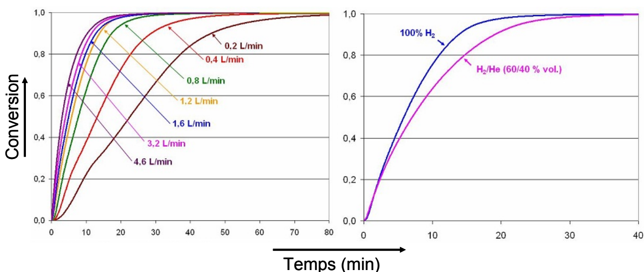
Figure II-6 : Réduction de boulettes CVRD-DR ( m_p \approx 5,5 \text{ g} , d_p \approx 14,5 \text{ mm} ) par \text{H}_2 pur, à 900°C : Effet du débit gazeux ( gauche ). Effet de l'inerte dans le gaz ( droite ).
