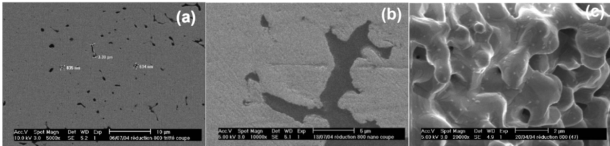
Figure I-17 : Images MEB des échantillons finaux obtenus par réduction, avec H_2 , à 800^\circ C , des morceaux de fritté (a), d'une nanopoudre (b) et d'une poudre (c) d'hématite [3].
