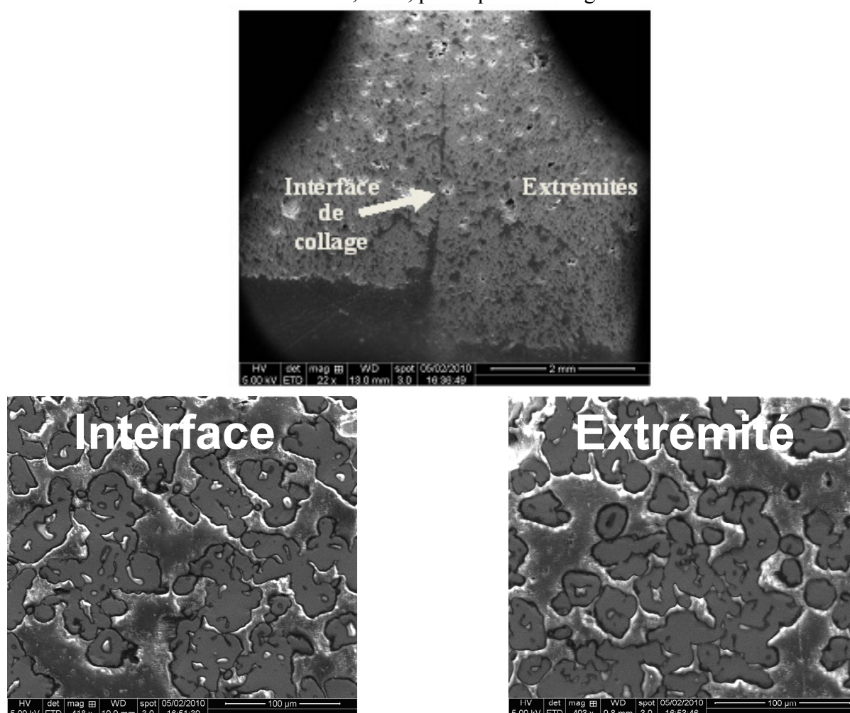
Figure III-10 : Observation au MEB des surfaces de collage entre deux moitiés d'une boulette réduite et enrobée avec une résine type époxy : essai à 1100°C, pendant 1h, sous H 2 /CO 50/50 % vol.
