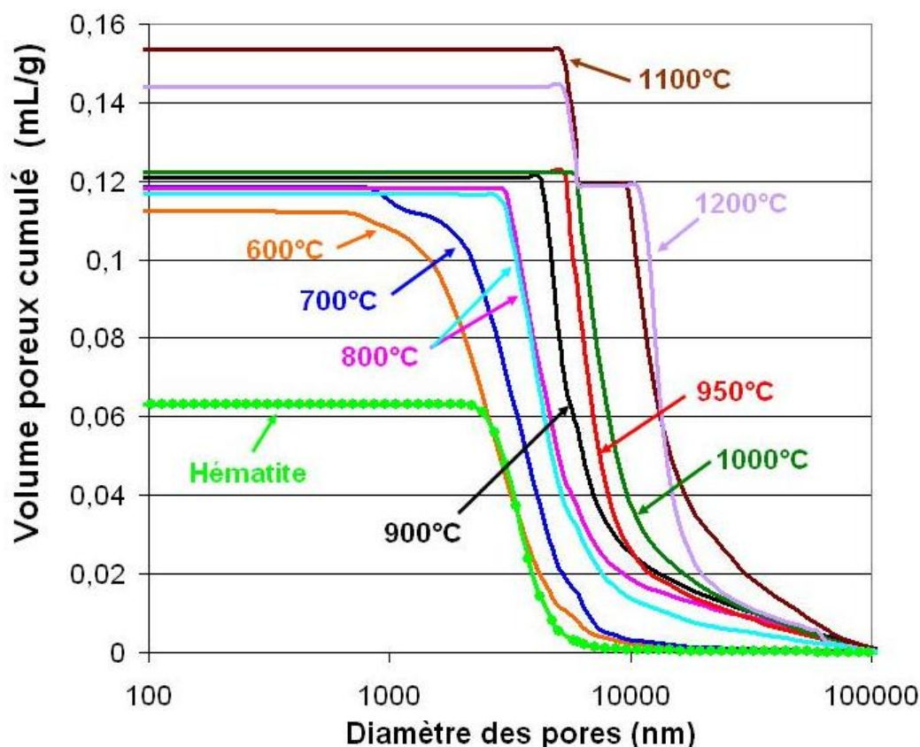
Figure II-42 : Volume poreux cumulé en fonction du diamètre des pores dans le fer final obtenu par la réduction, à différentes températures, de boulettes LKAB-KPRS ( m_p \approx 4,7 g ; 2 L/min de débit gazeux \text{H}_2/\text{He} 60/40 % vol.).
