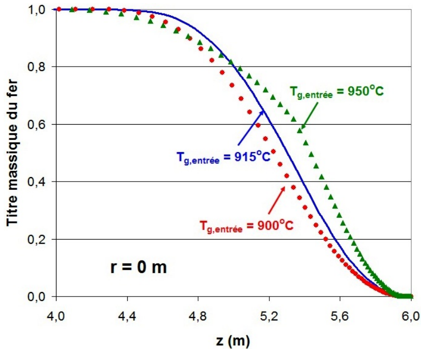
Figure V-13 : Variation du titre massique en fer dans le solide en fonction de la position axiale z , au centre de la cuve ( r = 0 m), pour les cas d'un mélange gazeux alimenté à 900°C, 915°C et 950°C. Boulettes du type CVRD-DR ( d_p = 0,014 m, \varepsilon_{ni,b} = 0,33 , a_{sp,b} = 0,0604 m 2 /g). Les autres conditions sont les mêmes que dans le cas de référence.
