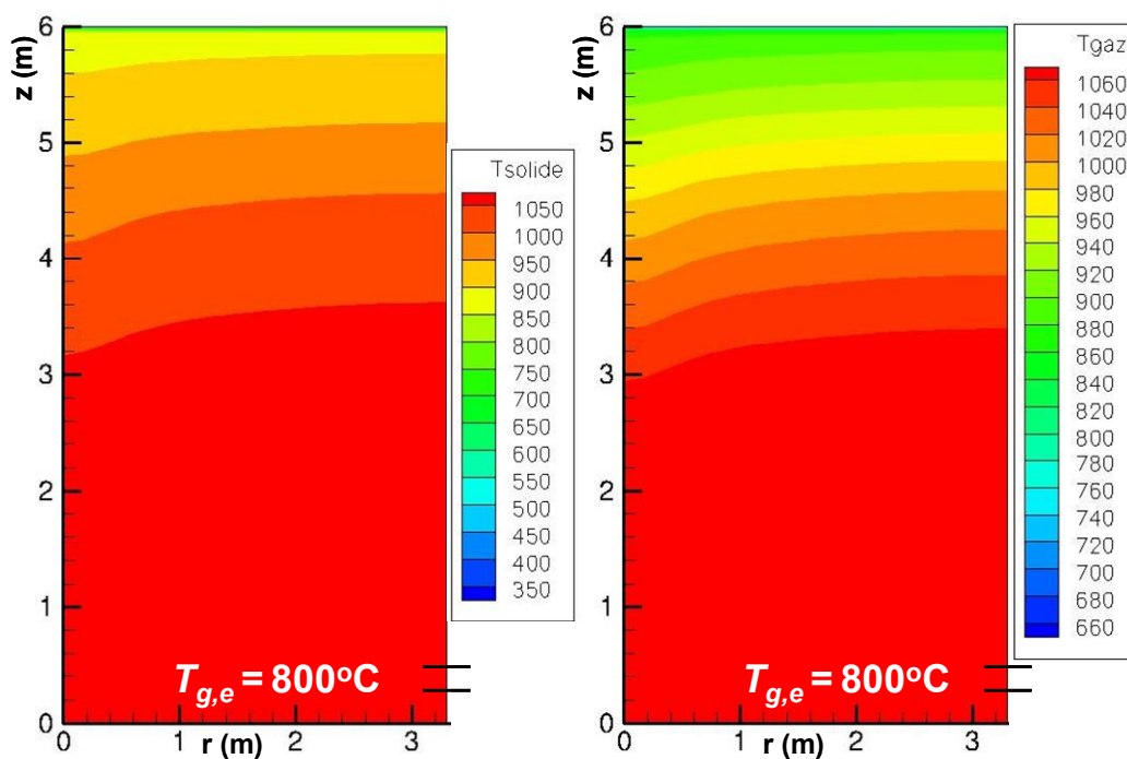
Figure V-7 : Évolution de la température du solide et du gaz (en K) à l'intérieur de la cuve dans les conditions de référence, avec des boulettes du type CVRD-DR ( d_p = 0,014 m, \varepsilon_{ini,b} = 0,33 , a_{sp,b} = 0,0604 m 2 /g).
