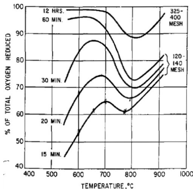
Figure I-18 : Effet de la température sur le taux de réduction de la magnétite (120 à 400 mesh) par H_2 pur [22].
