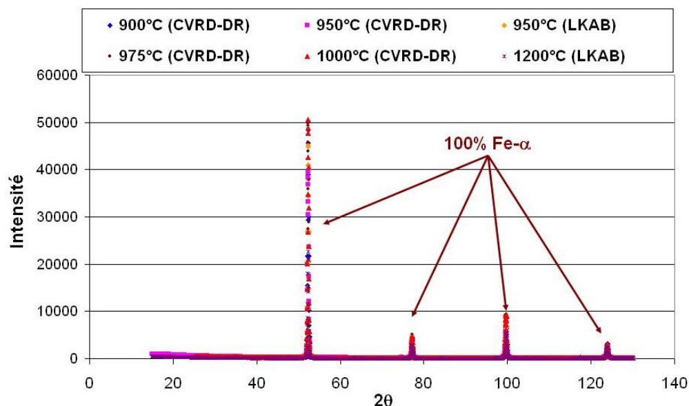
Figure II-17 : Spectres DRX de boulettes CVRD-DR et LKAB-KRPS complètement réduites par H 2 à différentes températures (2 L/min de débit gazeux H 2 /He 60/40 % vol.).
