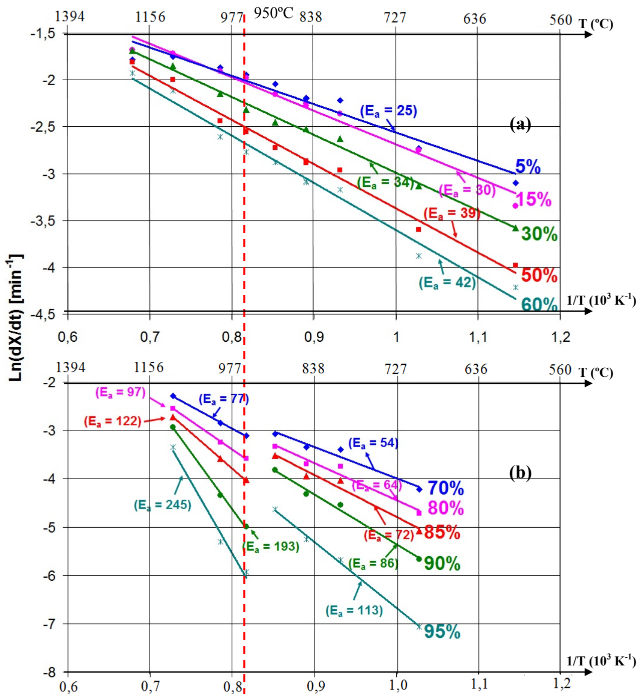
Figure II-28 : Diagramme Arrhenius représentant la réduction des boulettes LKAB-KPRS par H_2 , à différentes températures et conversions (2 L/min de débit gazeux H_2/He 60/40 % vol.) : (a) X < 60\% ; (b) X > 60\% . ( E_a en kJ/mol).
