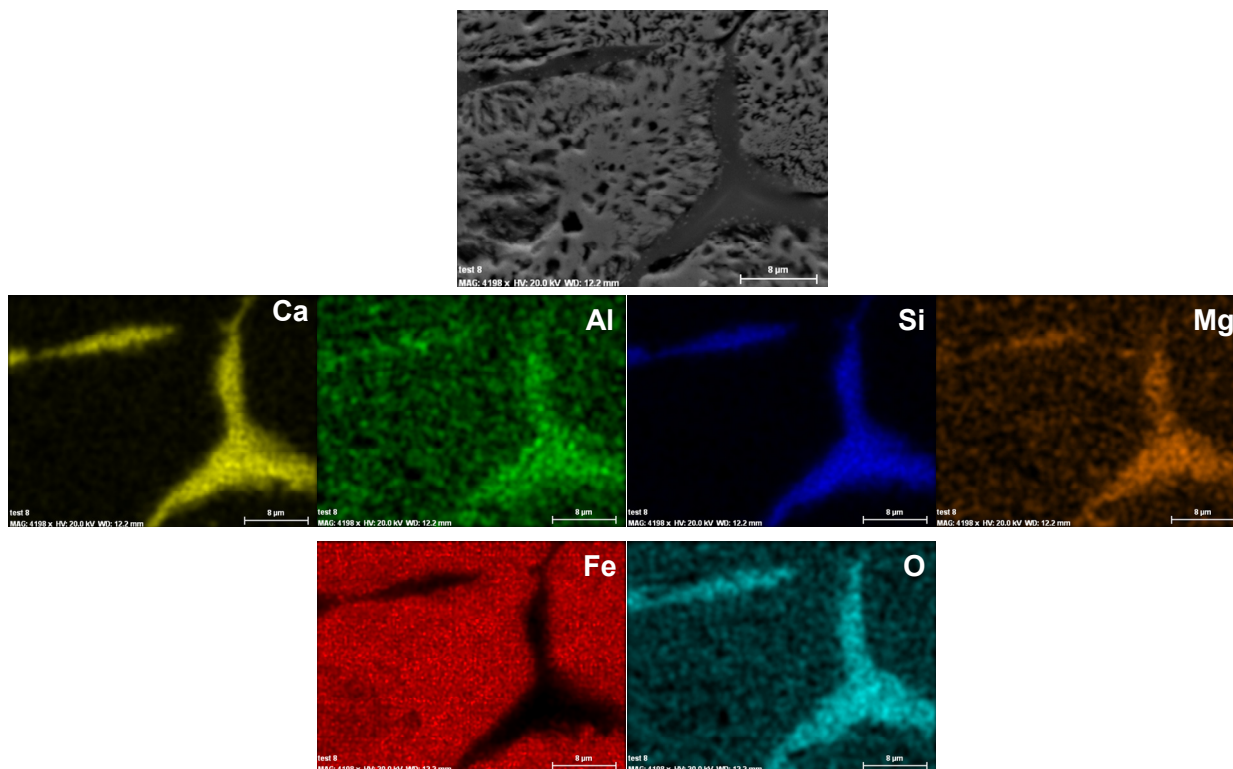
Figure III-19 : Images MEB SE (en haut) et images X (en bas) des éléments Al, Si, Ca, Mg, O (impuretés) et Fe. Boulette CVRD-DR réduite par H_2 , à 700°C (2 L/min de débit gazeux H_2/He 60/40 % vol.).
