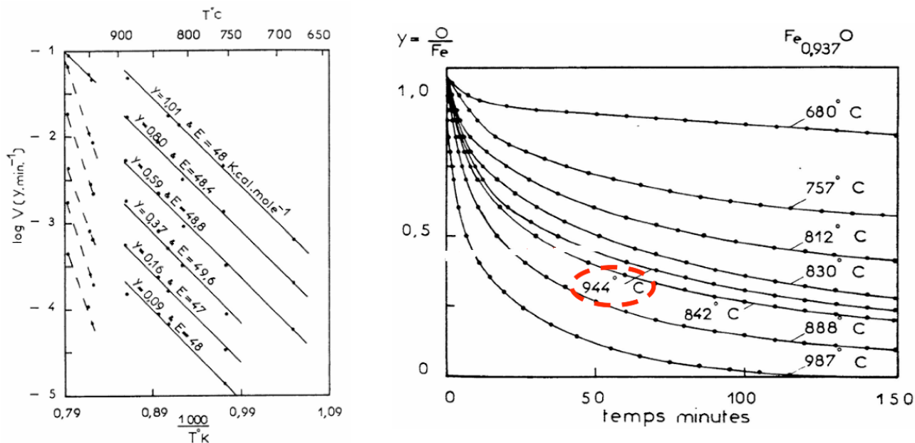
Figure II-20 : Réduction de la wüstite en poudre par H_2 pur, à différentes températures : Evolution de l'énergie d'activation ( kcal/mol ) pendant la transformation ( gauche ) ; courbes de perte de masse (atomes d'oxygène par rapport aux atomes de fer) à différentes températures ( droite ) [16].
