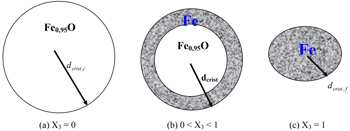
Figure AIII-1: Schéma de la réaction wüstite → fer : variation de la taille des cristallites ( d_{crist} ) au cours de la transformation ( X_3 = conversion de la réaction 3).
