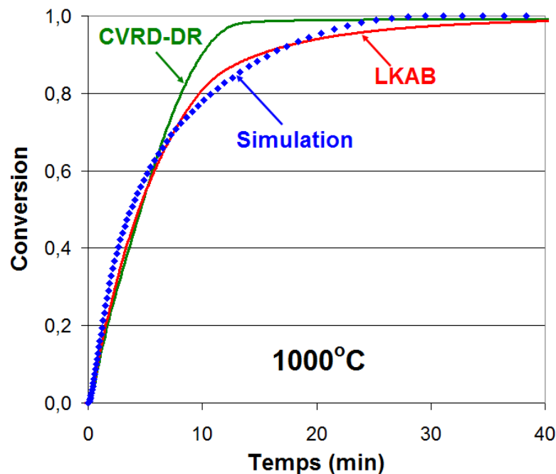
Figure IV-24 : Comparaison entre les résultats du modèle cinétique et les essais de thermogravimétrie. Simulation de la réduction des boulettes CVRD-DR et LKAB-KRPS ( d_p = 14 mm), à 1000°C, dans les conditions de référence (2 L/min de débit gazeux H_2/He 60/40 % vol.).
