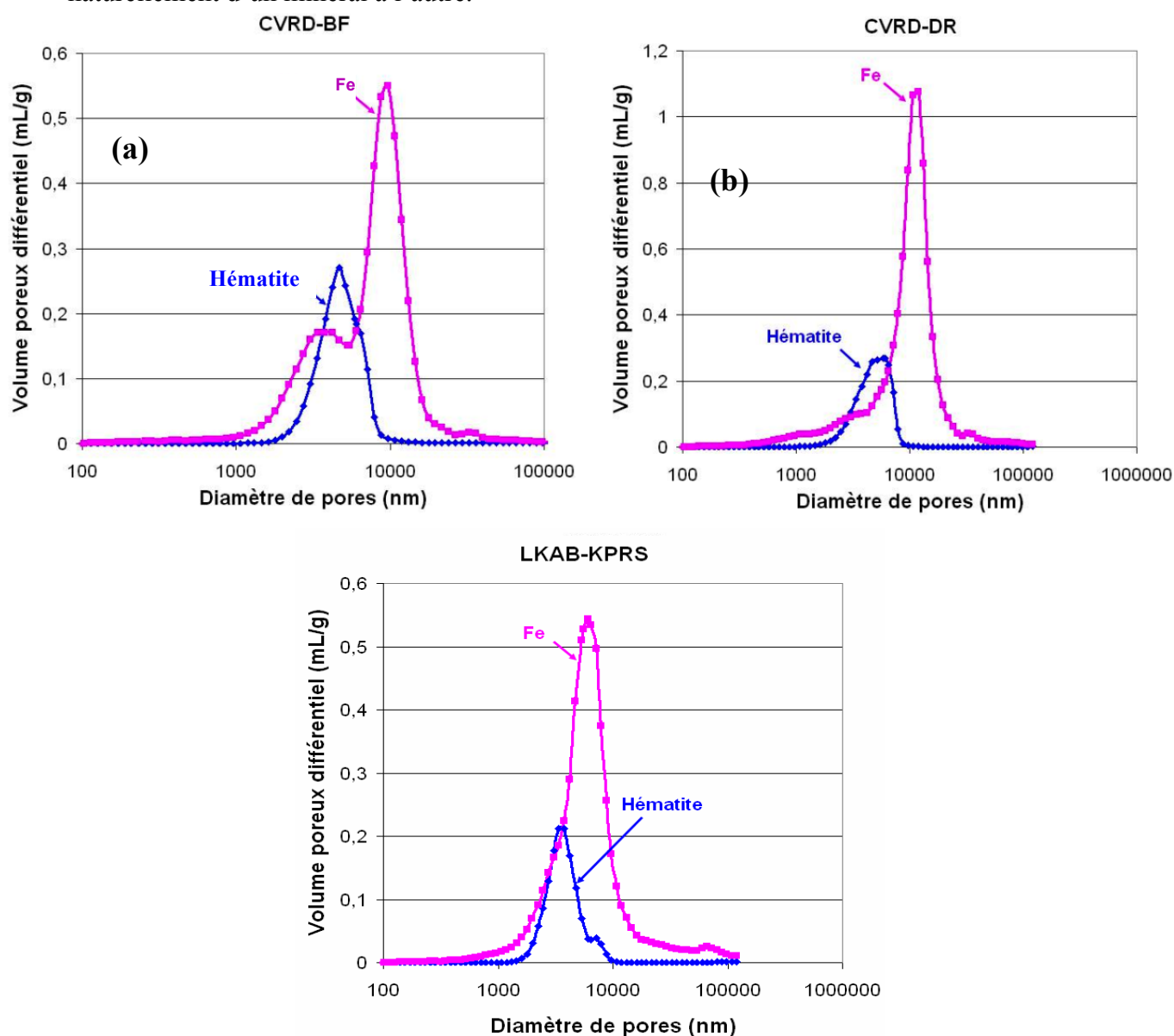
Figure II-39 : Distribution de taille des pores des différentes boulettes ( m_p \approx 3,7 g) réduites à 1000^\circ C : (a) CVRD-BF ; (b) CVRD-DR ; (c) LKAB-KPRS.
