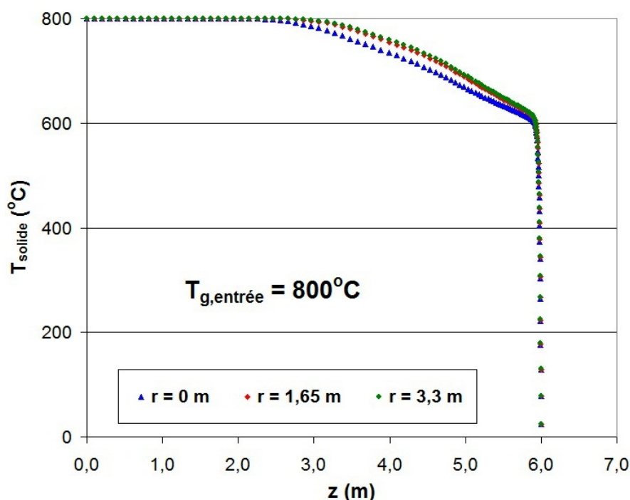
Figure V-10 : Variation de la température du solide avec l'hauteur du four, à différentes positions radiales ( r = 0 m, r = 1,65 m et r = 3,3 m). Conditions de référence, avec des boulettes du type CVRD-DR ( d_p = 0,014 m, \epsilon_{\text{ini},b} = 0,33 , a_{sp,b} = 0,0604 m 2 /g).
