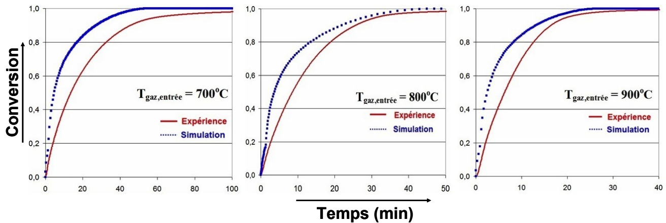
Figure IV-23 : Réduction de boulettes CVRD-BF par H_2 , à 700°C, 800°C et 900°C : courbes expérimentales et résultats obtenus par simulation de la cinétique du modèle REDUCTOR, initialement développé par Wagner [1].
