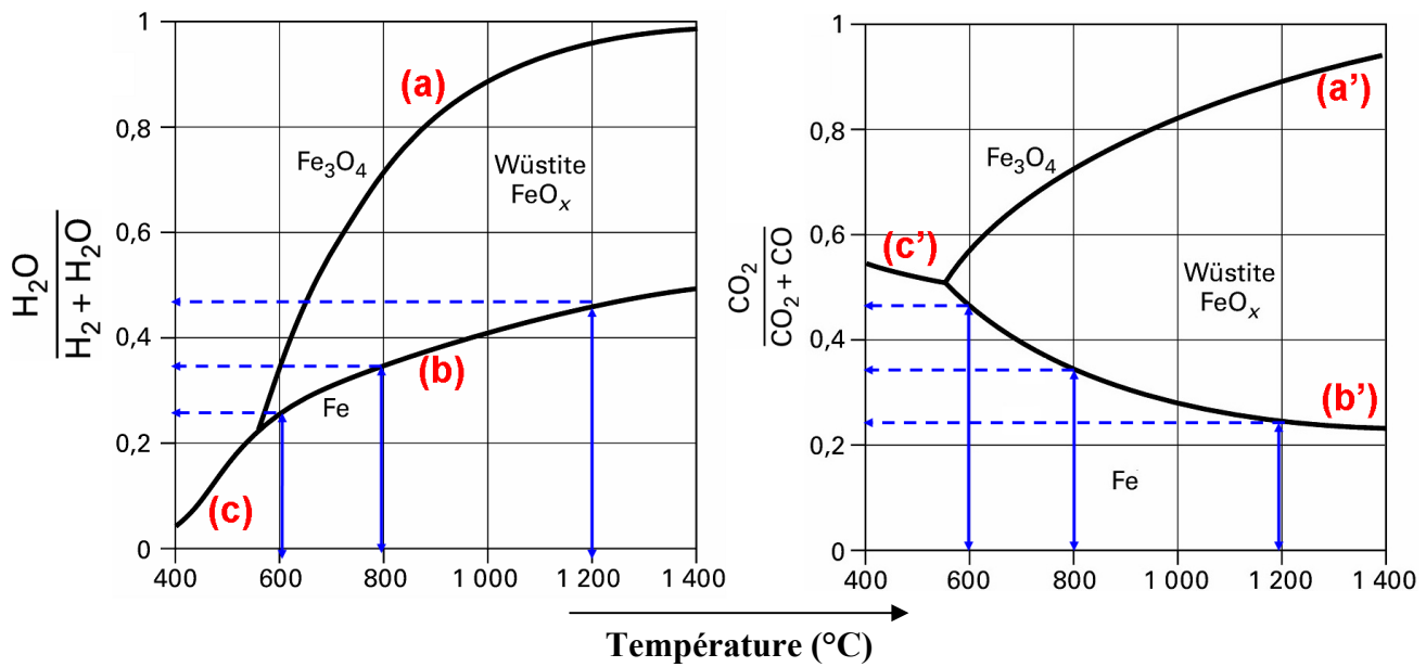
Figure I-6 : Diagrammes de Chaudron pour la réduction des oxydes de fer : domaines de stabilité des différents oxydes en fonction de la température et du pouvoir oxydant du gaz. Réduction par H_2 (gauche). Réduction par CO (droite). Les flèches représentent les forces motrices pour la réduction de la wüstite.
