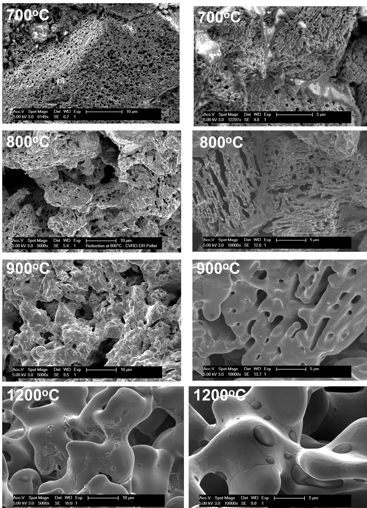
Figure II-21 : Images MEB (SE) des boulettes CVRD-DR complètement réduites par H_2 à 600°C, 700°C, 800°C, 900°C et 1200°C (2 L/min de débit gazeux H_2/He 60/40 % vol.). Images de gauche : grossissement de 5000x lors de l'enregistrement de l'image. Images de droite : grossissement de 10000x lors de l'enregistrement de l'image.
