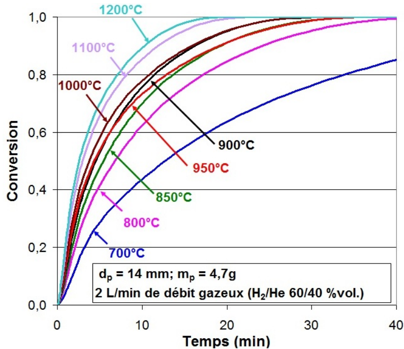
Figure IV-12 : Réduction des boulettes CVRD-DR ( d_p = 14 mm) à différentes températures (2 L/min de débit gazeux H_2/He 60/40 % vol). Résultats obtenus à partir des simulations avec le nouveau modèle cinétique.
