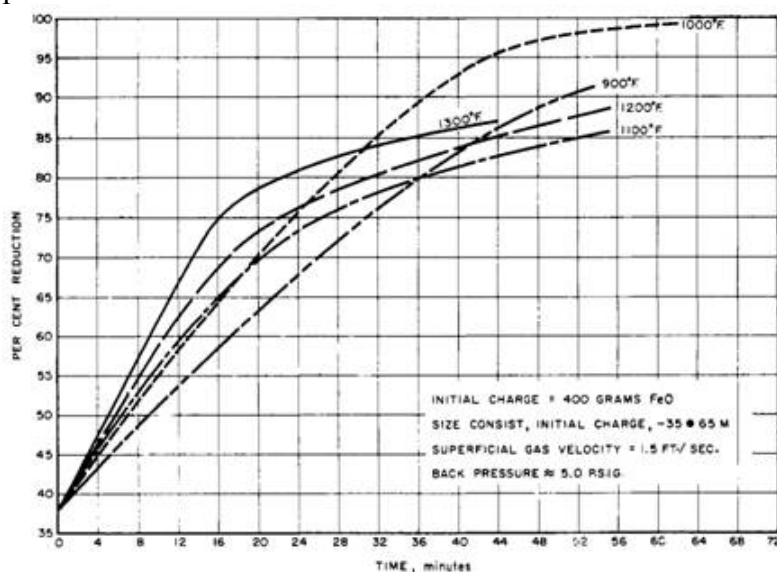
Figure I-20 : Effet de la température sur la cinétique de réduction par H_2 de fines de minerai de fer dans un lit fluidisé [13]
