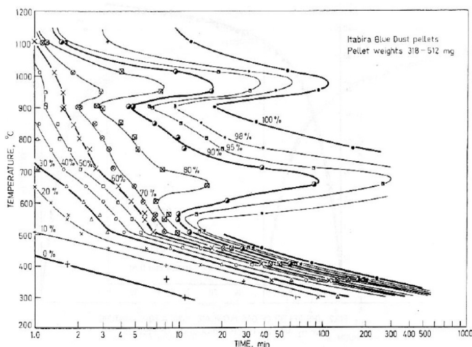
Figure II-16 : Effet de la température sur le temps de réduction de boulettes d'hématite par H_2 pur, pour différents degrés de conversion [51].
