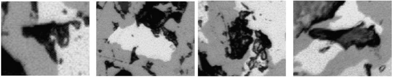
Figure I-27 : Images MEB de fines d'hématite partiellement converties en magnétite. Pores fermés avec surfaces partiellement réduites [40].
