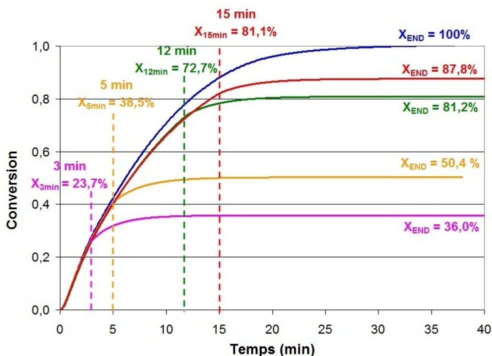
Figure II-31 : Courbes des réductions interrompues à 900°C : boulettes CVRD-DR partiellement réduites par H_2 (2 L/min de débit gazeux H_2/He 60/40 % vol.).
