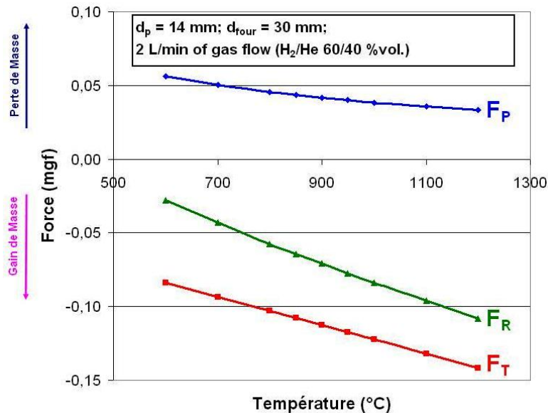
Figure AV-1 : Force résultante sur la boulette, à l'intérieur de la thermobalance TG96 : 2 L/min de débit gazeux H 2 /He 60/40 % vol., d p = 14 mm, d four = 30 mm. F p (force de poussée), F T (force de traînée), F R (force résultante)
