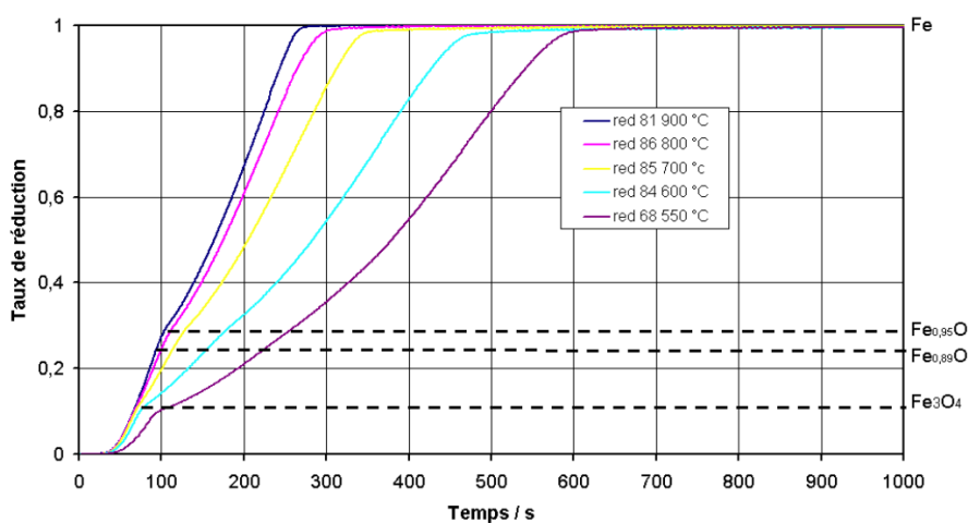
Figure I-21 : Influence de la température sur la réduction, par H_2 , de poudre synthétique d'hématite [3].
