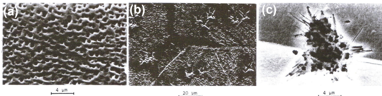
Figure I-34 : Images MEB des piqûres sur les surfaces d'échantillons denses de wüstite \text{Fe}_{0,90}\text{O} réduits par le mélange \text{H}_2/\text{H}_2\text{O} . (a) 900°C, 90 % \text{H}_2 , 30 s ; (b) 800°C, 90 % \text{H}_2 , 60 s ; (c) 900°C, 70 % \text{H}_2 , 30 s [33].
