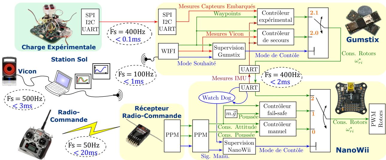
FIGURE III.2 – La structure logicielle du quadrirotor X 4 -MaG. Différents modes de fonctionnement sont disponibles afin de sécuriser la plateforme. Le mode expérimental de la Gumstix permet de tester de nouveaux algorithmes utilisant une charge expérimentale (capteurs embarqués). Dans le mode expérimental ou de secours , la Nanowii se contente de transmettre les consignes aux rotors calculées par la Gumstix. Un bloc de supervision Gumstix permet de basculer automatiquement sur le contrôleur de secours , si le robot s'écarte trop de son objectif. De même, en cas de défaillance de la Gumstix, le superviseur Nanowii enclenche le mode fail-safe pour stabiliser au mieux le robot, en attendant une reprise manuelle. Enfin, le mode manuel de la Nanowii permet d'asservir la poussée et l'attitude sur les consignes envoyées par la radio-commande. Ce mode manuel peut être enclenché à tout moment par l'utilisateur car il dispose de la priorité la plus élevée.
