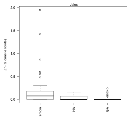
Figure 6.25 : Boxplots présentant le pourcentage atomique en Zn en surface du solide suite à l'analyse systématique des minéraux présents dans les échantillons de Jales témoin, HA et GA.
