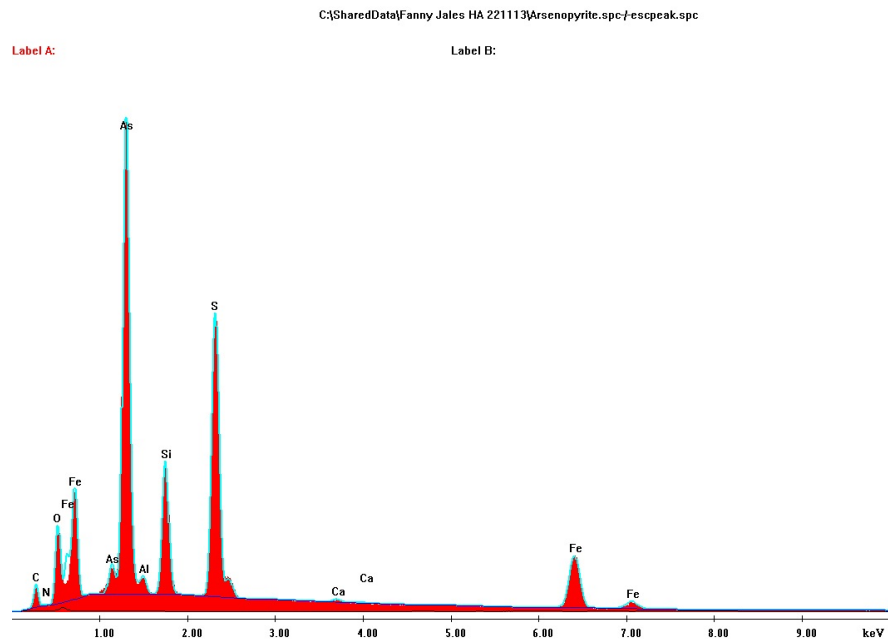
(c) Spectre EDS de la zone notée (a) de la figure 6.9 : Arsénopyrite
