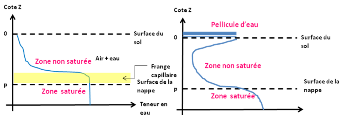
Figure 2.5 : Représentation schématique des transferts d'eau dans le sol (Dingman, 2002).
