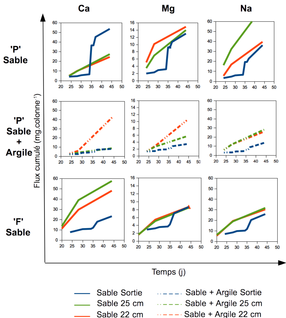
Figure 4.12 : Flux cumulés de Ca, Mg et Na obtenus par 'F' et 'P' à partir du jour 24 de l'expérience, dans les colonnes de sable et de sable + argile.
