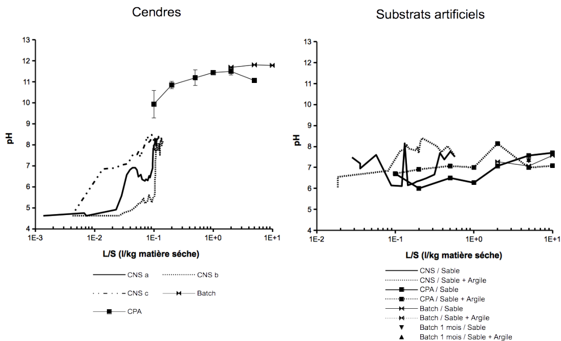
Figure 4.16 : pH en fonction du ratio L/S pour les colonnes non saturées (pour les réplicats CNSa, CNSb, CNSc), les colonnes à percolation ascendantes CPA et les batchs.
