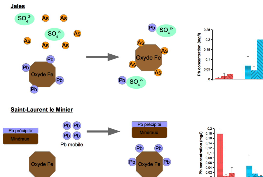
Figure 6.65 : Schéma conclusion des mécanismes d'immobilisation du Pb lors de l'apport de GA aux sols de Jales et Saint-Laurent le Minier.
