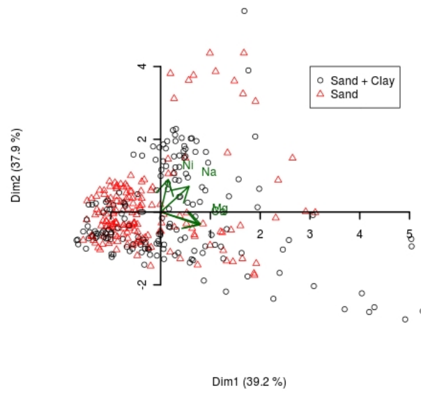
Figure 4.8 : Projection des échantillons en fonction du type de substrat sur un plan factoriel F1 * F2.
