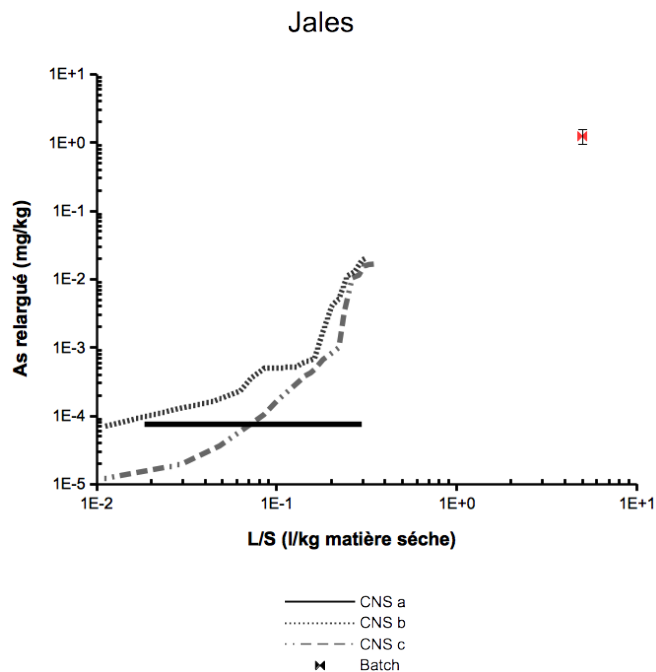
Figure 4.18 : As relargué en fonction du ratio L/S pour les colonnes non saturées (pour les réplicats CNSa, CNSb, CNSc) et les batchs pour le sol de Jales.
