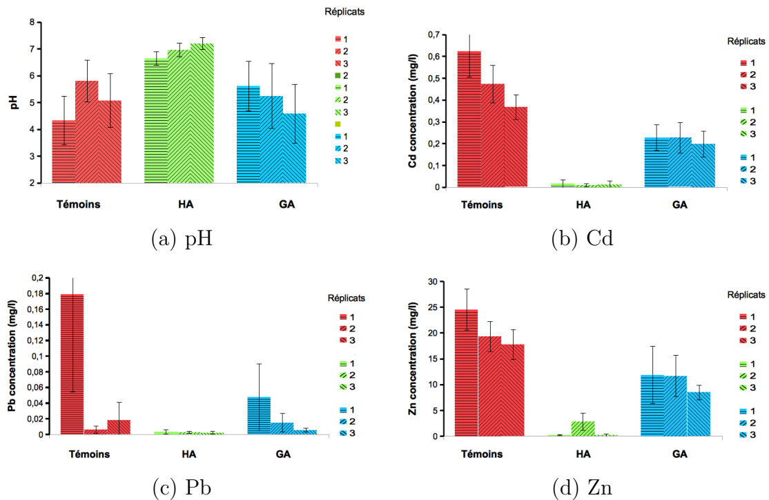
Figure 6.52 : Valeurs moyennes du pH et des concentrations en Cd, Pb et Zn des solutions de percolation dans les colonnes de laboratoire pour des ratios L/S allant de 0,1 à 0,4 l\ kg^{-1} dans le sol de Saint-Laurent le Minier. Les barres verticales représentent les écarts-types sur l'ensemble des prélèvements de chaque colonne.
