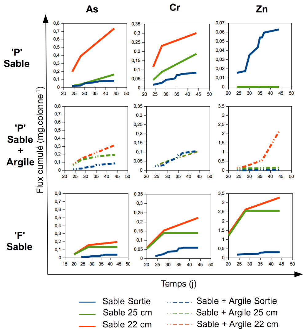
Figure 4.13 : Flux cumulés de As, Cr et Zn obtenus par 'F' et 'P' à partir du jour 24 de l'expérience, dans les colonnes de sable et de sable + argile.
